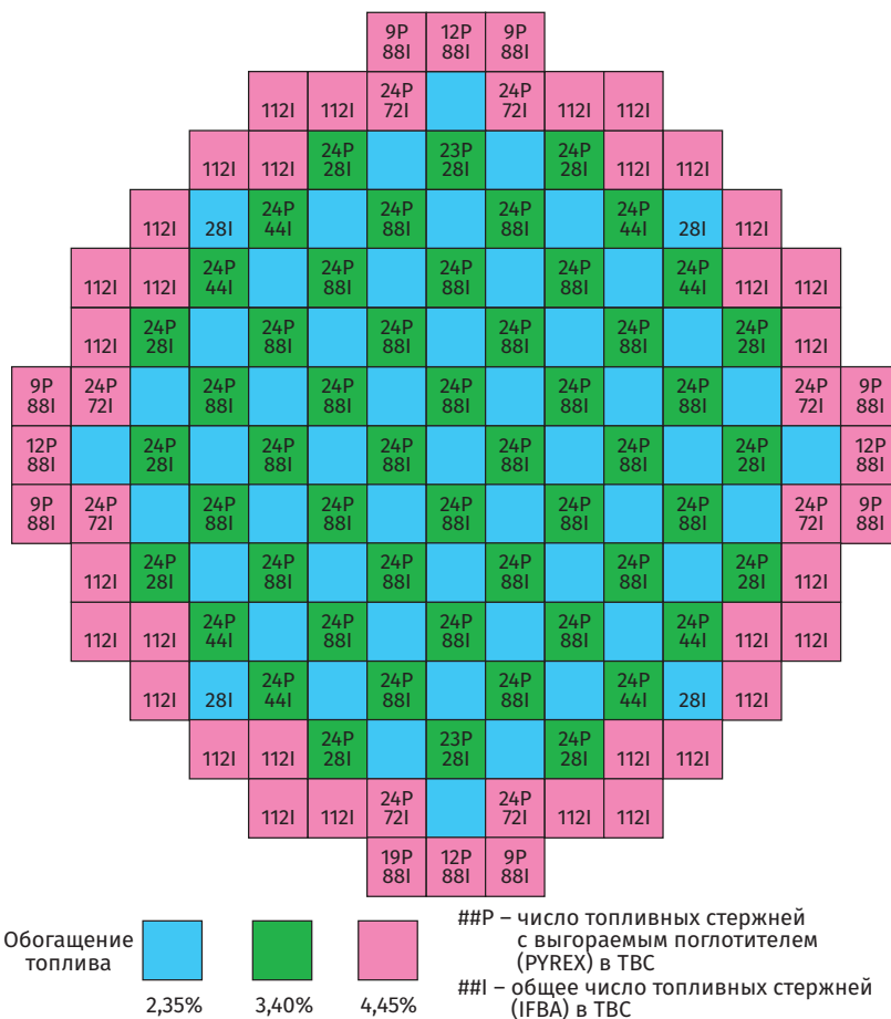
Рис. 3.8. Картограмма размещения ТВС различного обогащения топлива в активной зоне AP1000
