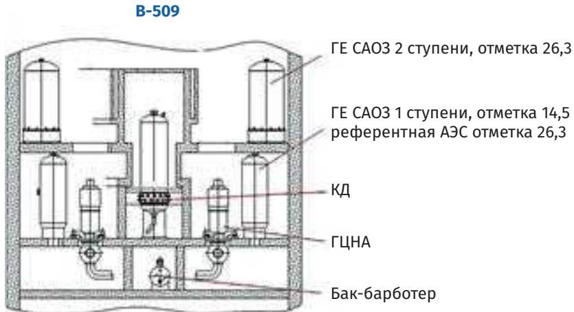
Рис. 2.69. Расположение гидроемкостей САОЗ первой ступени в проекте В-509 АЭС «Аккую»
