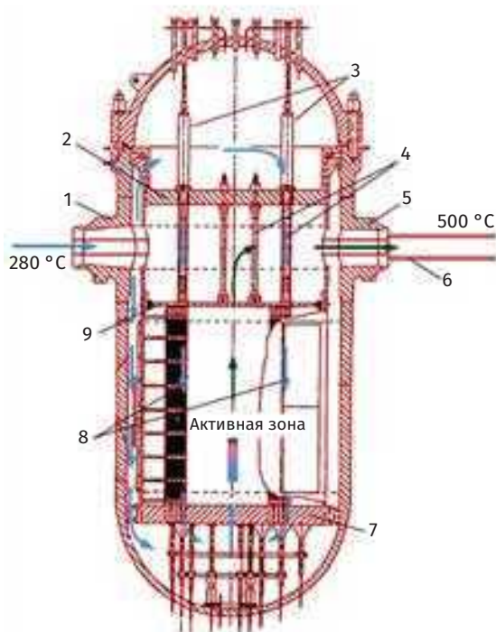
Рис. П2.31. Реактор SCWR INEEL – первый вариант реактора.
