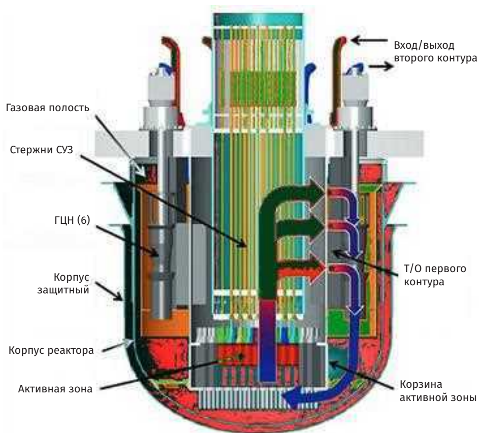
Рис. П2.20. Конструкция реактора и схема потоков теплоносителя концептуальной установки Westinghouse PLFR
