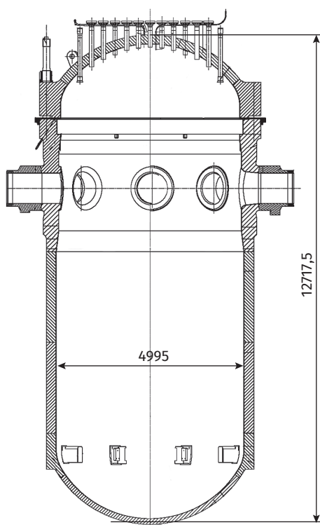
Рис. 3.28. Корпус реактора EPR-1600 с крышкой
