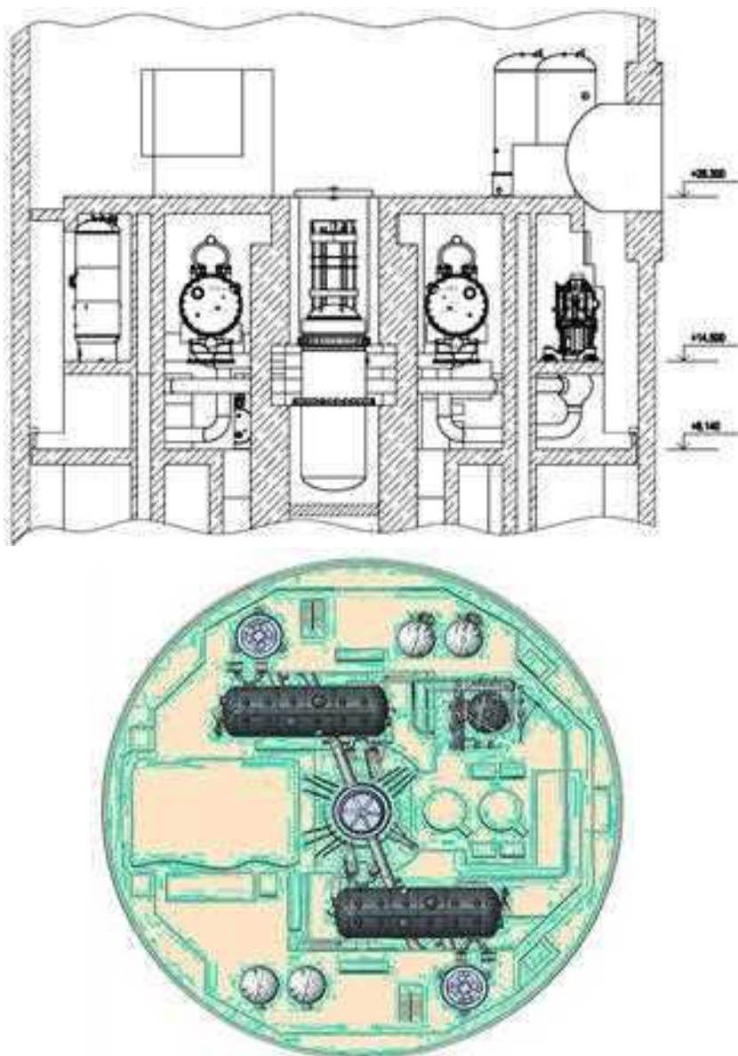
Рис. 2.75. Компоновка элементов РУ В-551С в герметичной оболочке
