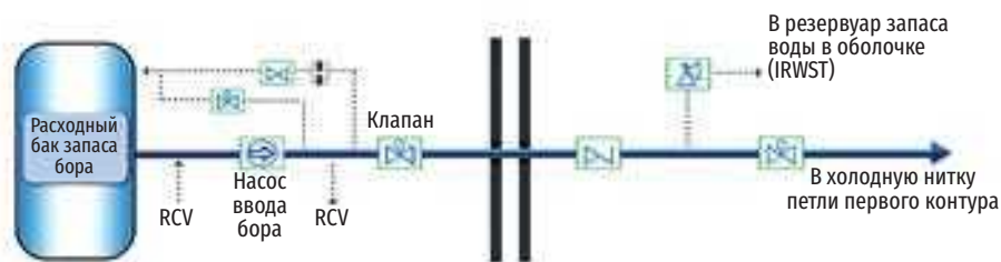
Рис. 3.106. Упрощенная схема канала системы аварийного ввода бора HPR1000 [RBS] (EBS)] (RCV – система подпитки-продувки 1 контура)
