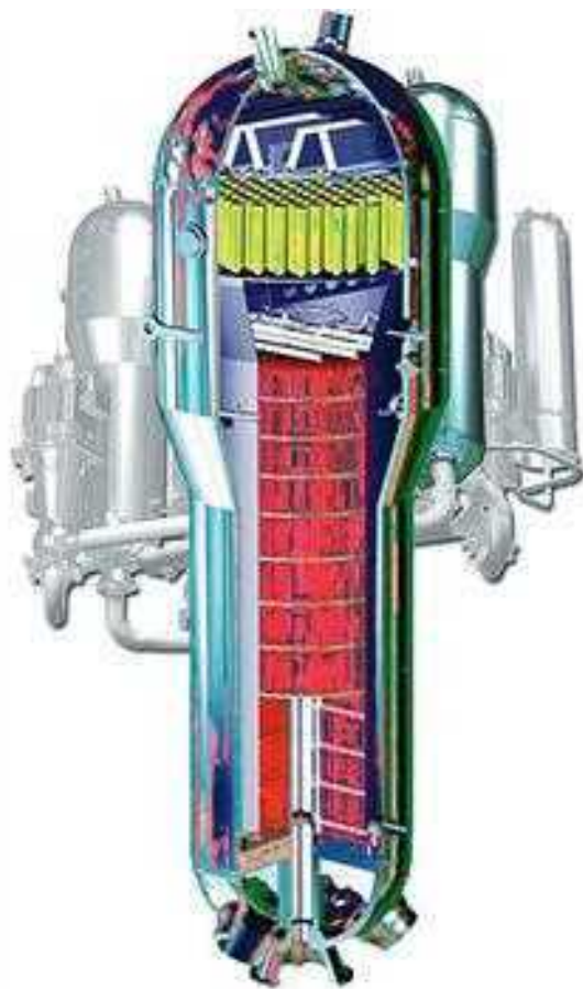
Рис. 3.68. Общий вид конструкции парогенератора в разрезе APR1400
