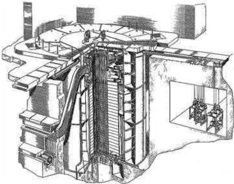
Рис. 1.5. Конструкция графитового реактора АМ-1
