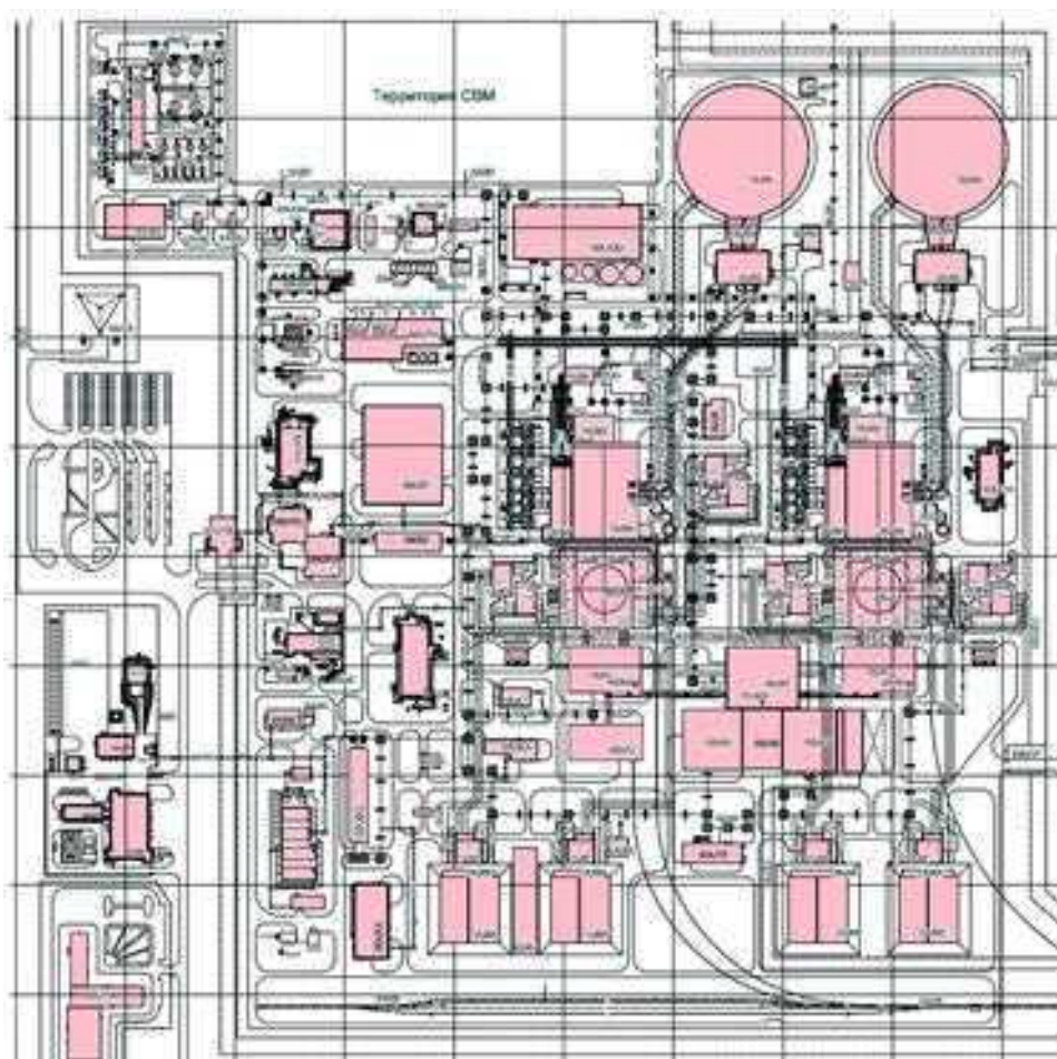
Рис. 2.85. Схема генерального плана Кольской АЭС-2
