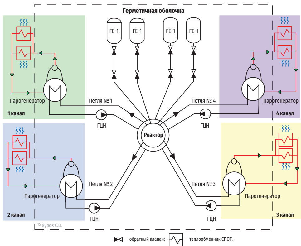
Рис. 2.26. Система пассивного отвода тепла. Проект В-392М (НВАЭС-2)
