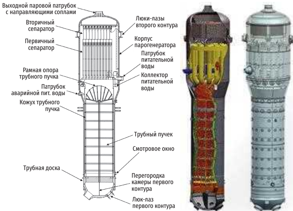
Рис. 3.102. Схема внутренних устройств парогенератора HPR1000
