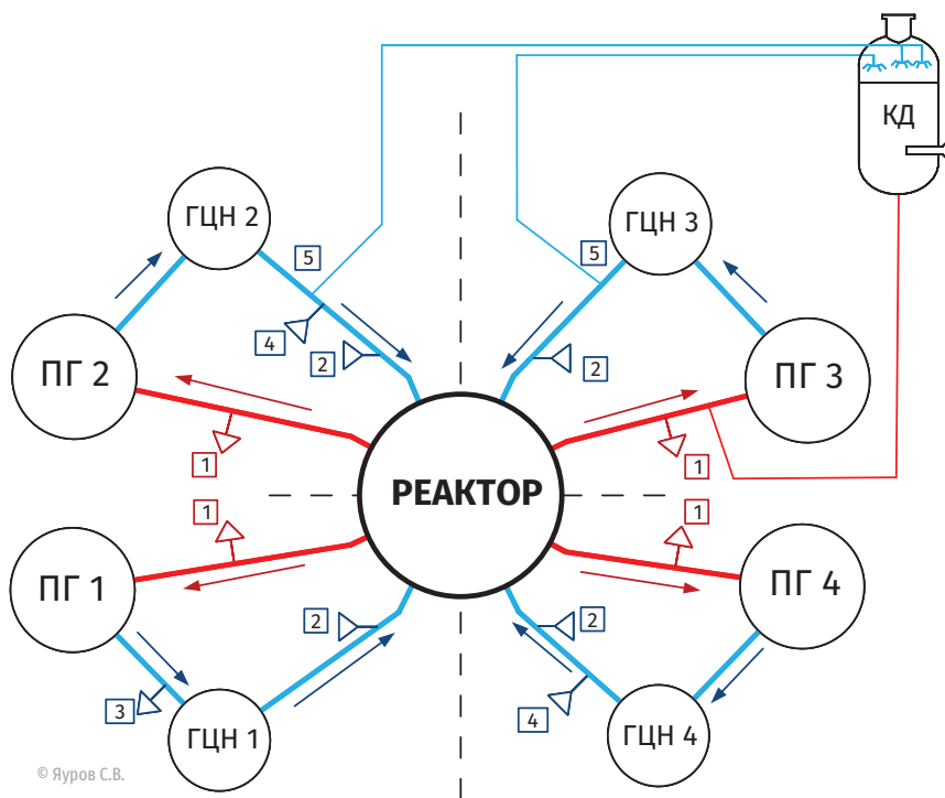
Рис. 3.26. Конфигурация оборудования и трубопроводов первого контура EPR-1600. 1 – система отвода остаточного тепла реактора (SIS/RHRS); 2 – система дополнительного борирования [RBS (EBS)], система аварийного впрыска/система отвода остаточного тепла реактора [RIS/RRA (SIS/RHRS)]; система гидроемкостей (гидроаккумуляторов); 3 – забор воды в систему подпитки-продувки 1 контура RCV (CVCS); 4 – подача воды в систему подпитки-продувки 1 контура RCV (CVCS); 5 – линии впрыска компенсатора давления (КД)
