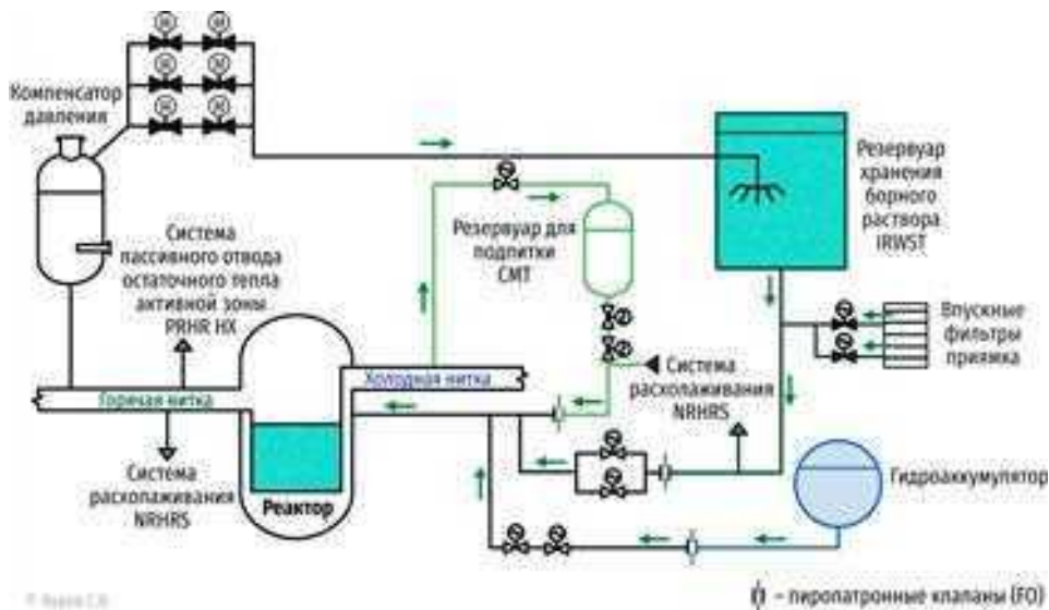
Рис. 3.17. Схема залива активной зоны реактора AP1000
