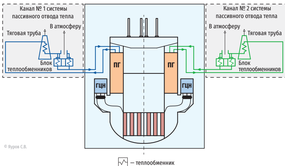
Рис. 1.24. Принципиальная схема системы пассивного отвода тепла. РУ РИТМ-200Н
