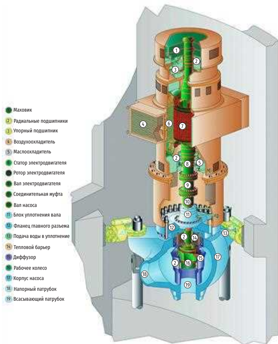
Рис. 3.38. Разрез главного циркуляционного насоса EPR-1600
