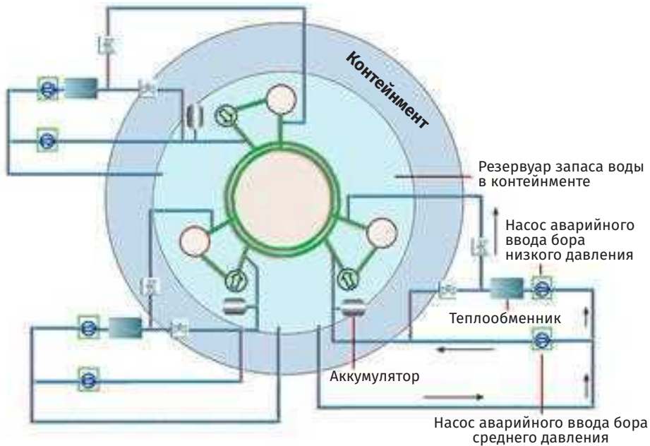
Рис. 3.105. Упрощенная схема системы аварийного впрыска бора RIS (SIS) HPR1000
