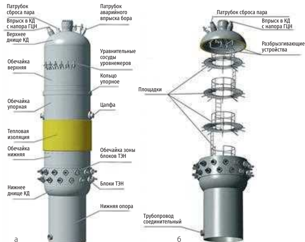
Рис. 2.15. Компенсатор давления. Проект В-392М (НВАЭС-2).
