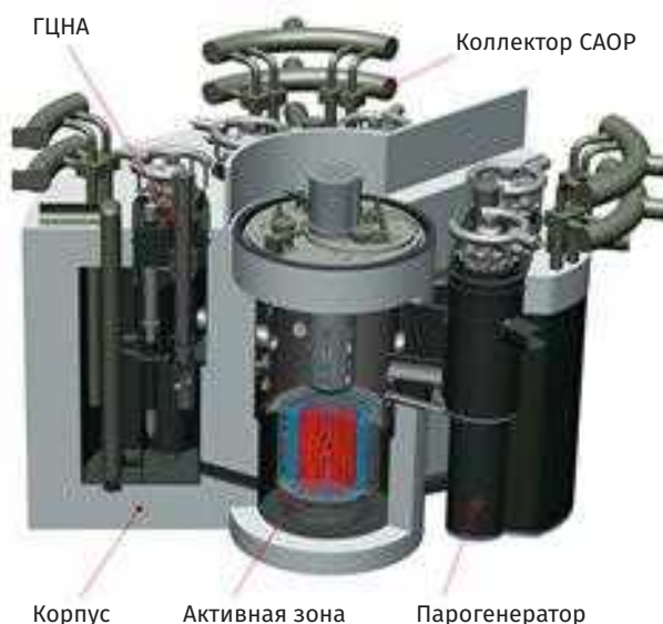
Рис. П2.10. Основные элементы РУ БРЕСТ-ОД-300
