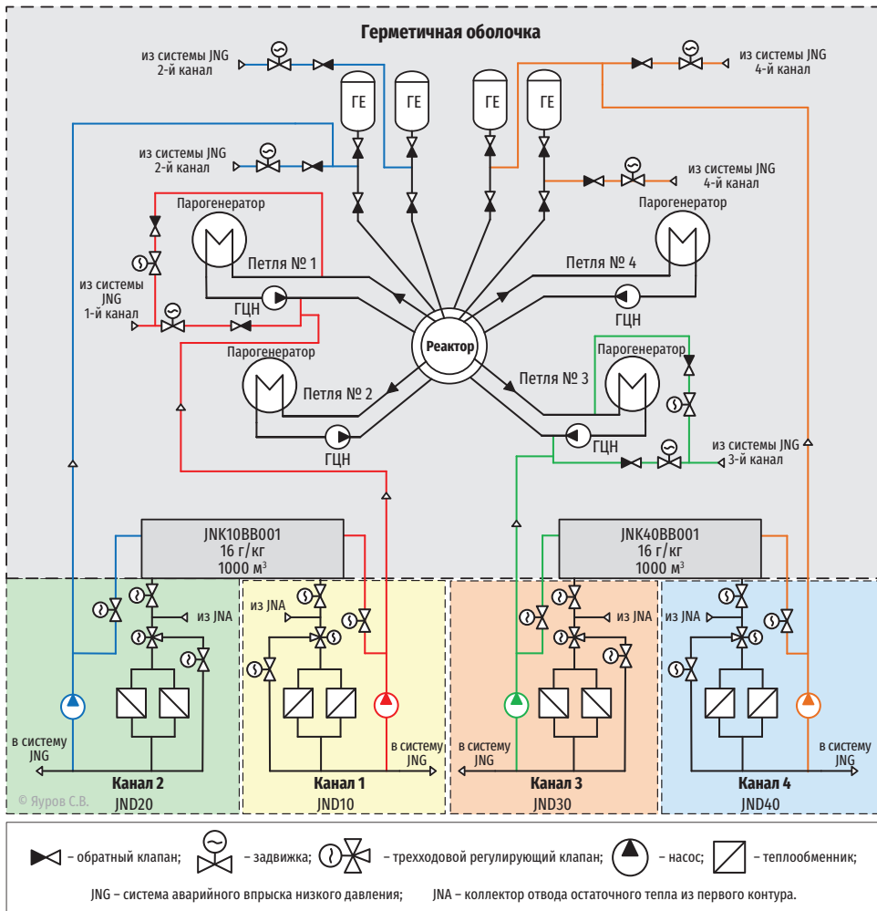
Рис. 2.36. Упрощенная технологическая схема системы аварийного впрыска высокого давления JND. Проект В-491 (ЛАЭС-2)
