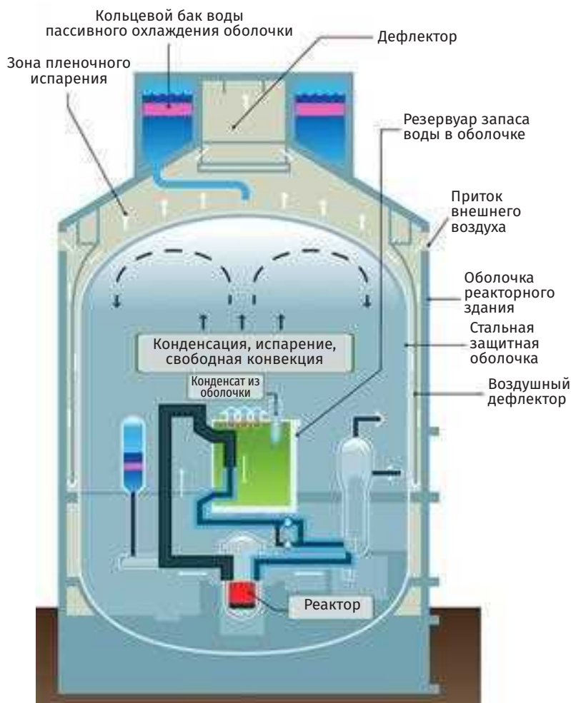
Рис. 3.19. Схема тепловых потоков пассивного охлаждения оболочки AP1000
