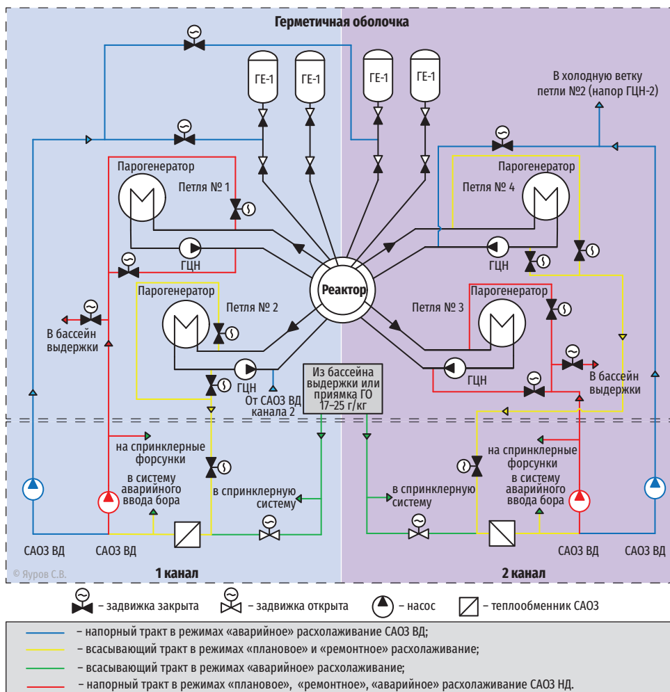
Рис. 2.58. Технологическая схема системы аварийного и планового расхолаживания и охлаждения бассейна выдержки проекта В-509 (АЭС «Аккую»)
