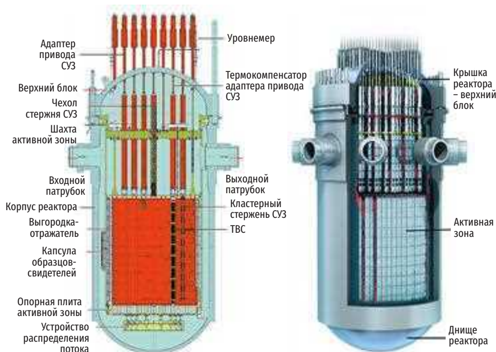
Рис. 3.27. Конструкция реактора EPR-1600
