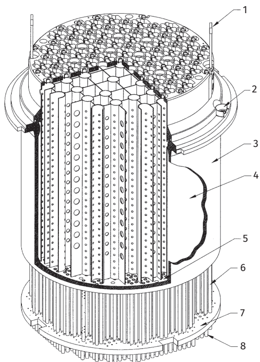
Рис. 3.58. Верхняя направляющая конструкция реактора APR1400.
