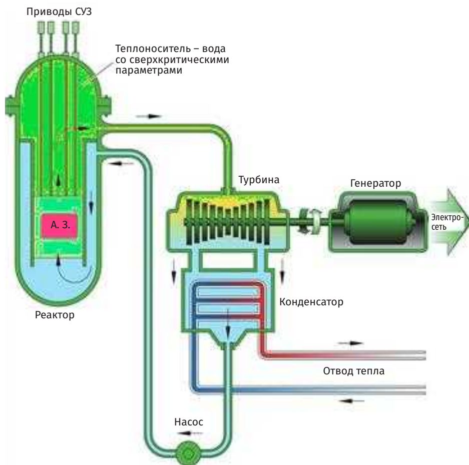
Рис. П2.30. Сверхкритический водоохлаждаемый реактор SCWR (SuperCritical Water-cooled Reactor)
