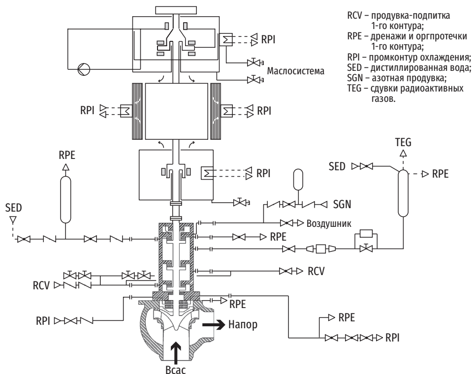
Рис. 3.37. Принципиальная схема ГЦН EPR-1600 и его вспомогательных систем
