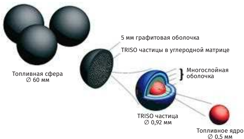
Рис. П2.41. Конструкция твэла шарообразного типа
