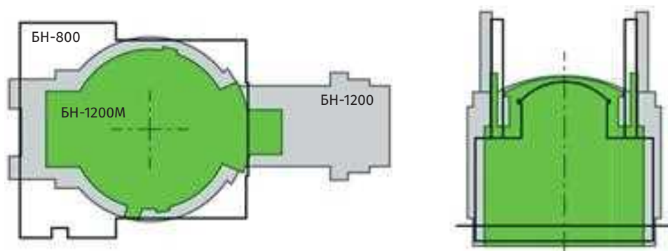
Рис. П2.29. Сравнение габаритных компоновок блоков БН-800, 1200 и 1200М
