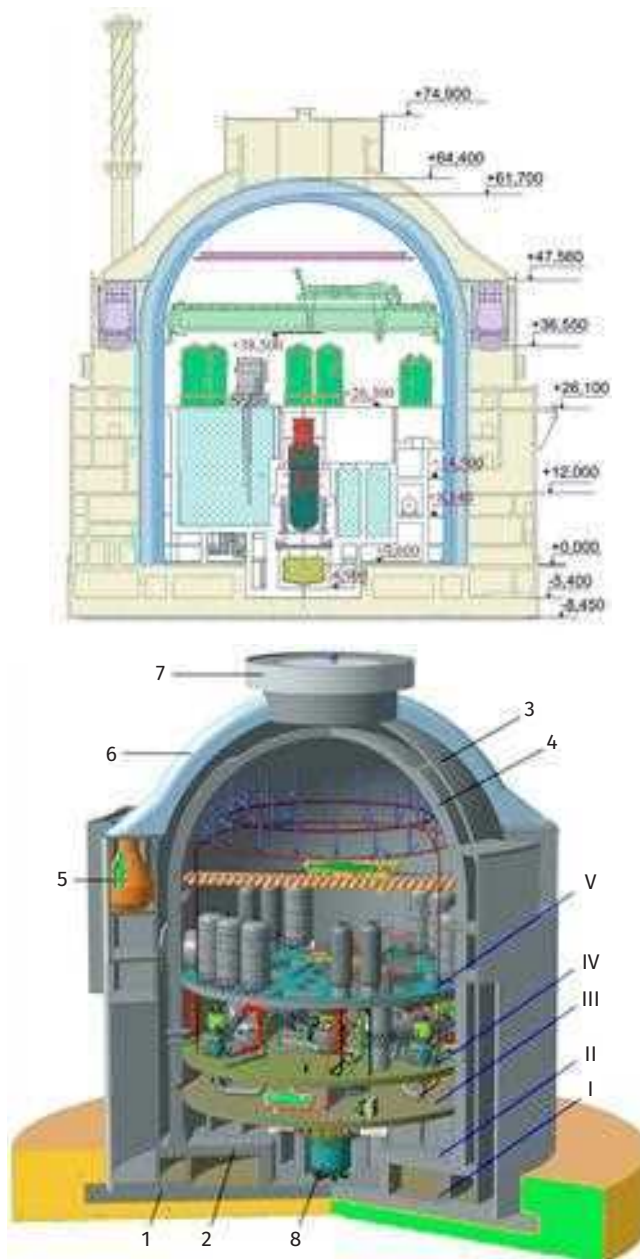
Рис. 2.32. Расположение оборудования в гермооболочке. Проект В-392М (НВАЭС-2).
