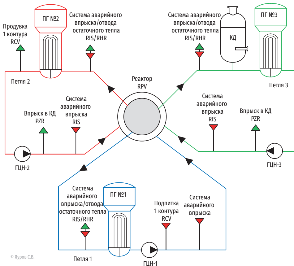
Рис. 3.86. Принципиальная схема первого контура HPR1000
