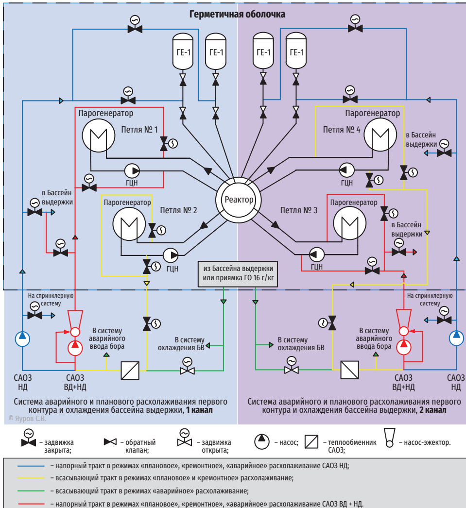
Рис. 2.23. Структура системы аварийного и планового расхолаживания первого контура и охлаждения бассейна выдержки (два канала). Проект В-392М (НВАЭС-2)
