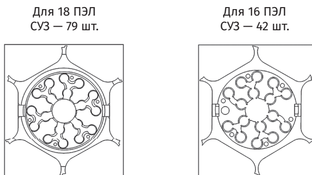
Рис. 2.53. Защитные трубы БЗТ
