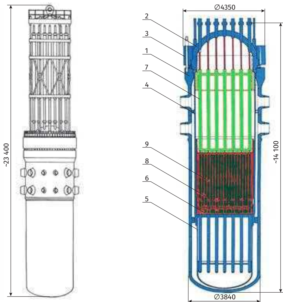
Рис. 1.12. Реактор ВВЭР-440.
