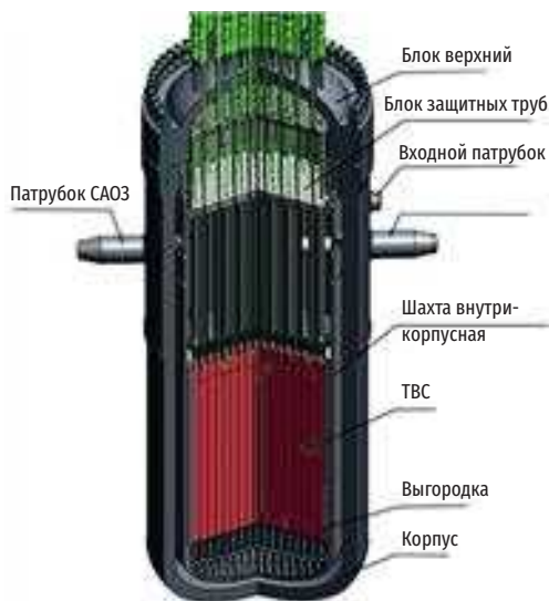
Рис. П2.37. Конструкция реактора ВВЭР-СКД-1700
