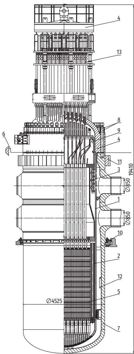
Рис. 2.76. Реактор проекта В-551С.
