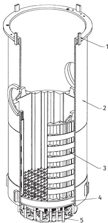
Рис. 3.57. Опорные конструкции активной зоны в шахте внутрикорпусных устройств РУ APR1400. 1 – направляющие; 2 – шахта внутрикорпусная; 3 – выгородка активной зоны; 4 – нижняя плита активной зоны; 5 – каналы устройств ВКУ
