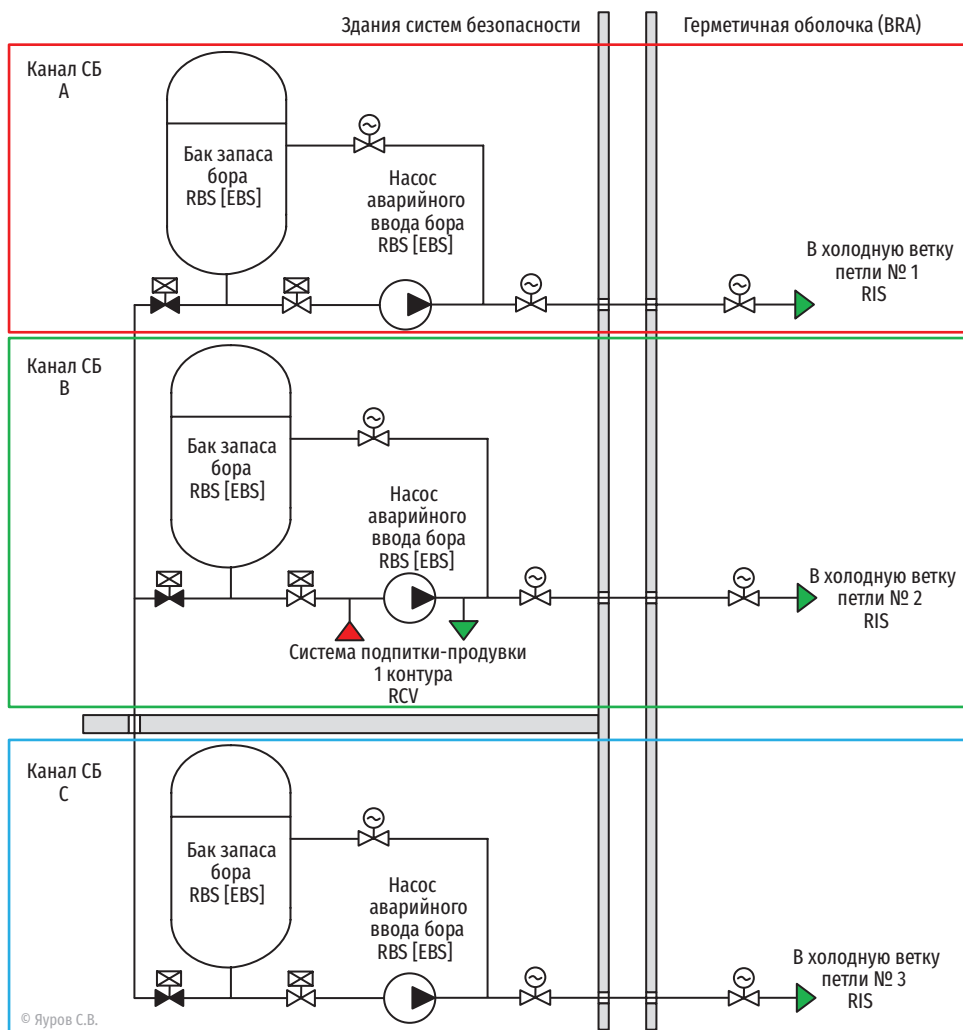
Рис. 3.107. Принципиальная схема системы аварийного ввода бора HPR1000 [RBS] (EBS)]
