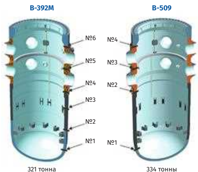
Рис. 2.50. Корпус реактора проектов В-392М и В-509
