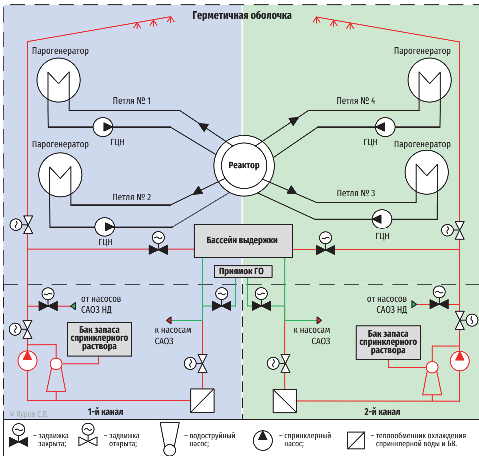
Рис. 2.28. Упрощенная схема подачи воды на форсунки спринклерной системы от насосов системы охлаждения бассейна выдержки FAK. Проект В-392М (НВАЭС-2)
