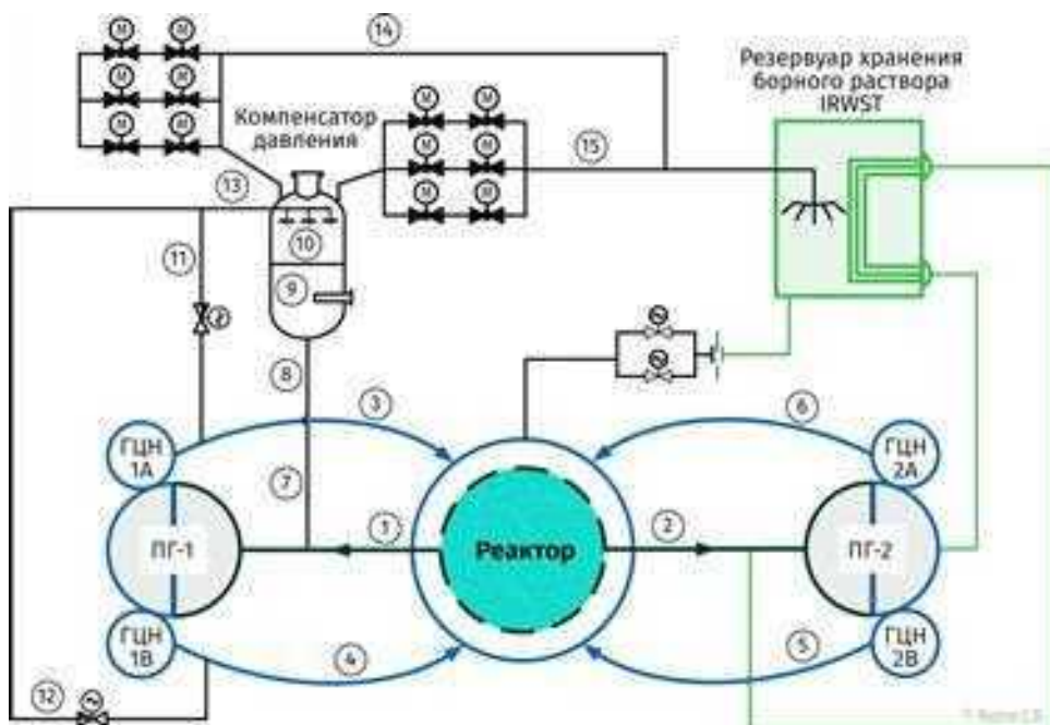
Рис. 3.10. Принципиальная схема подключения компенсатора давления в АР1000.
