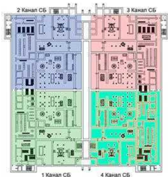
Рис. 2.81. Компоновка и расположение оборудования каналов СВ в здании обстройки энергоблока ВВЭР-С
