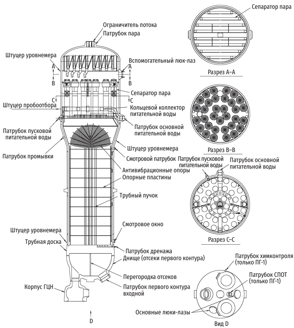
Рис. 3.14. Конструкция парогенератора AP1000
