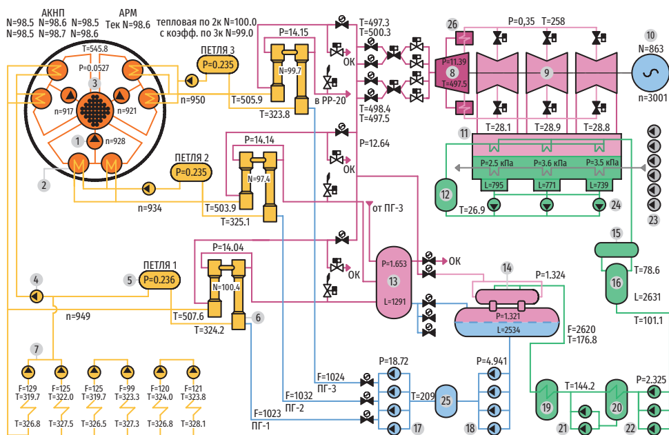
Рис. П2.26. Принципиальная тепловая схема и основное оборудование реакторной установки БН-800.
