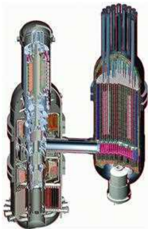
Рис. П2.42. Реакторс блоком преобразования энергии российской версии установки ГТ-МГР с призматическими блоками
