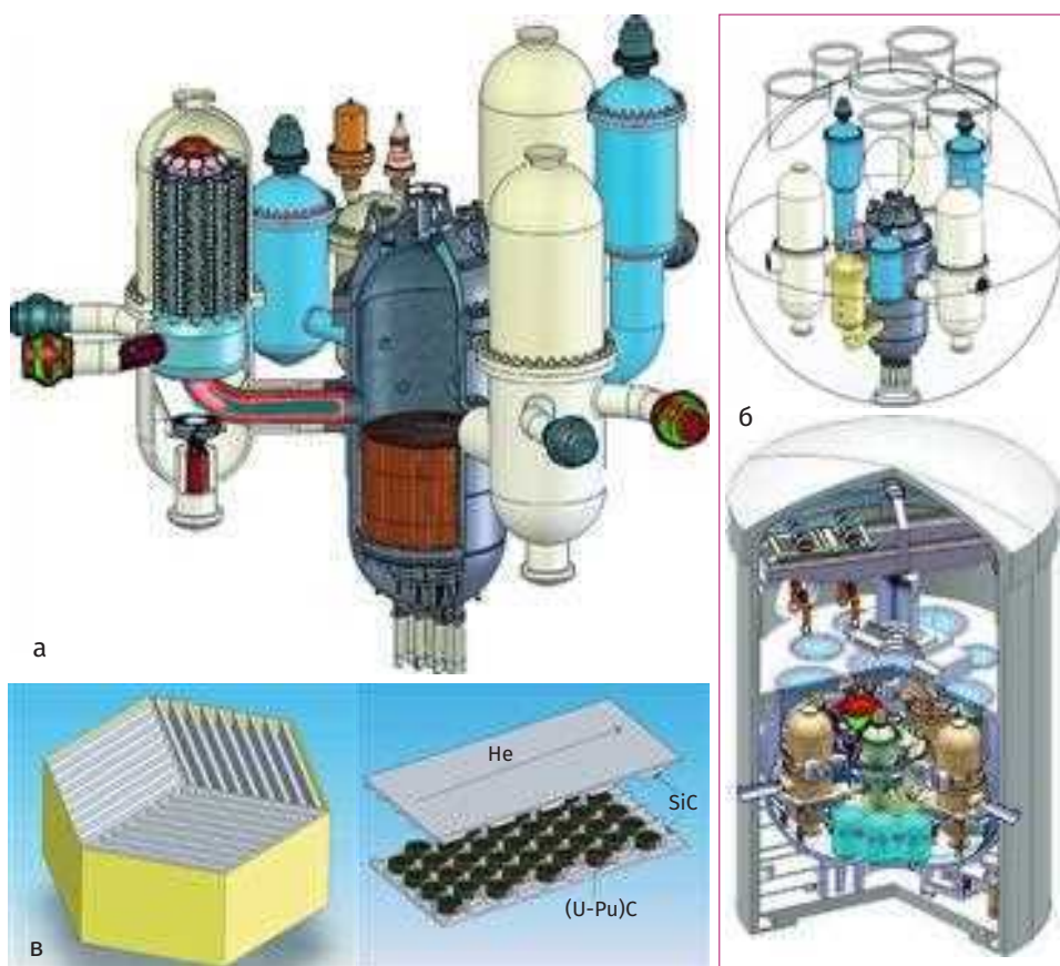
Рис. П2.4. Типовой проект GEN IV GFR.
