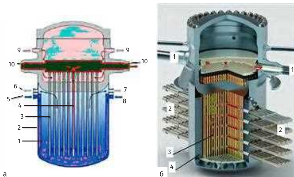
Рис. П2.34. Схема циркуляции (а) и общий вид (б) реактора Canadian SCWR.
