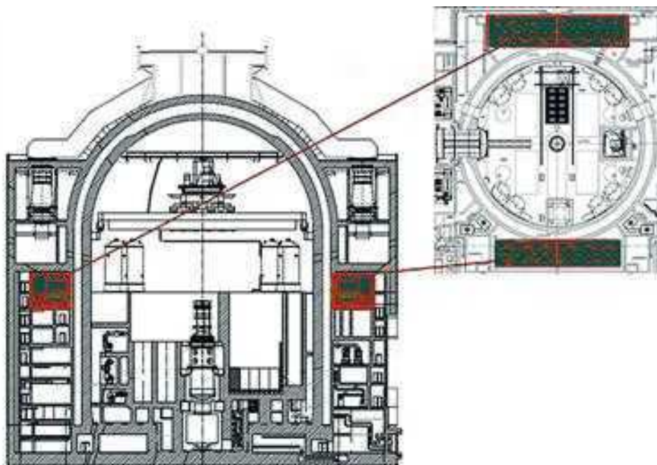
Рис. 2.70. Размещение ГЕ-3 САОЗ Проект В-509 (АЭС «Аккую»)
