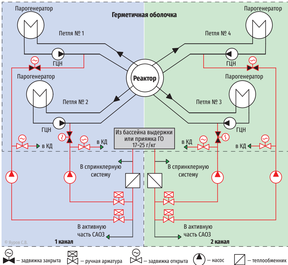
Рис. 2.57. Технологическая схема системы аварийного ввода бора проекта В-509 (АЭС «Аккую»)
