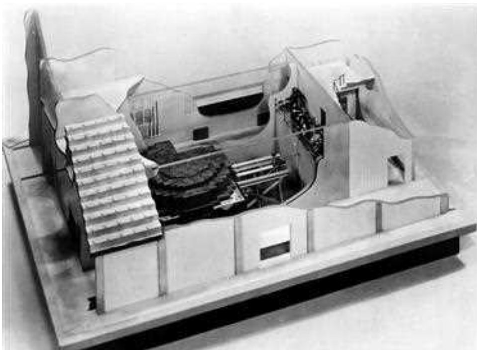
Рис. 1.4. Модель реактора Chicago Pile-1
