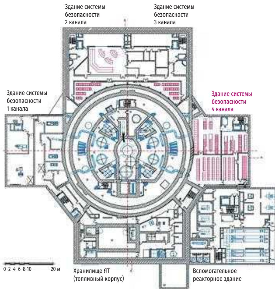
Рис. 3.47. План зданий «ядерного острова» энергоблока ERP-1600 и размещение оборудования РУ и СБ
