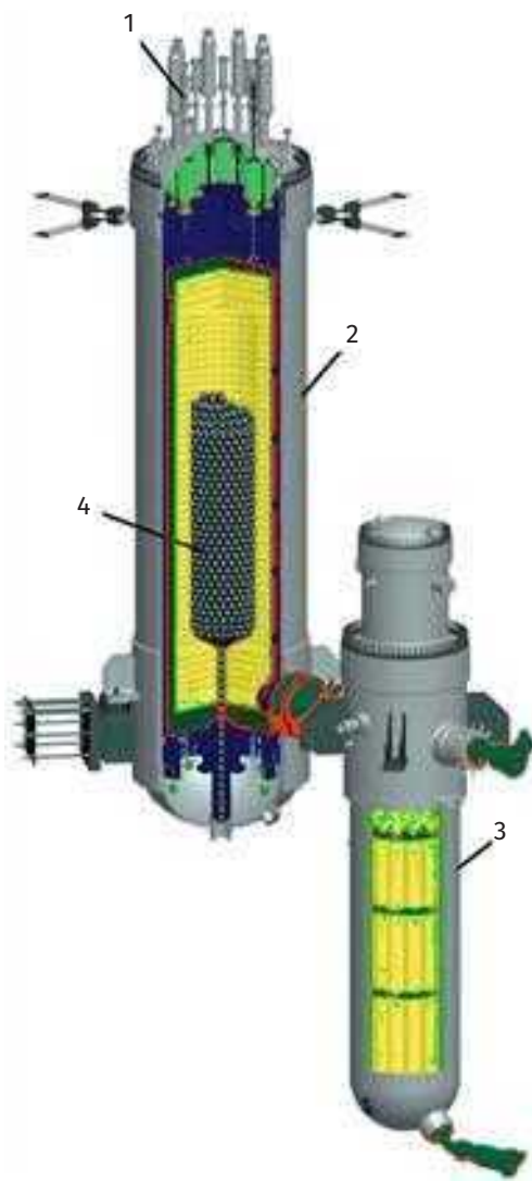
Рис. П2.45. Реакторный модуль установки HTR-PM.
