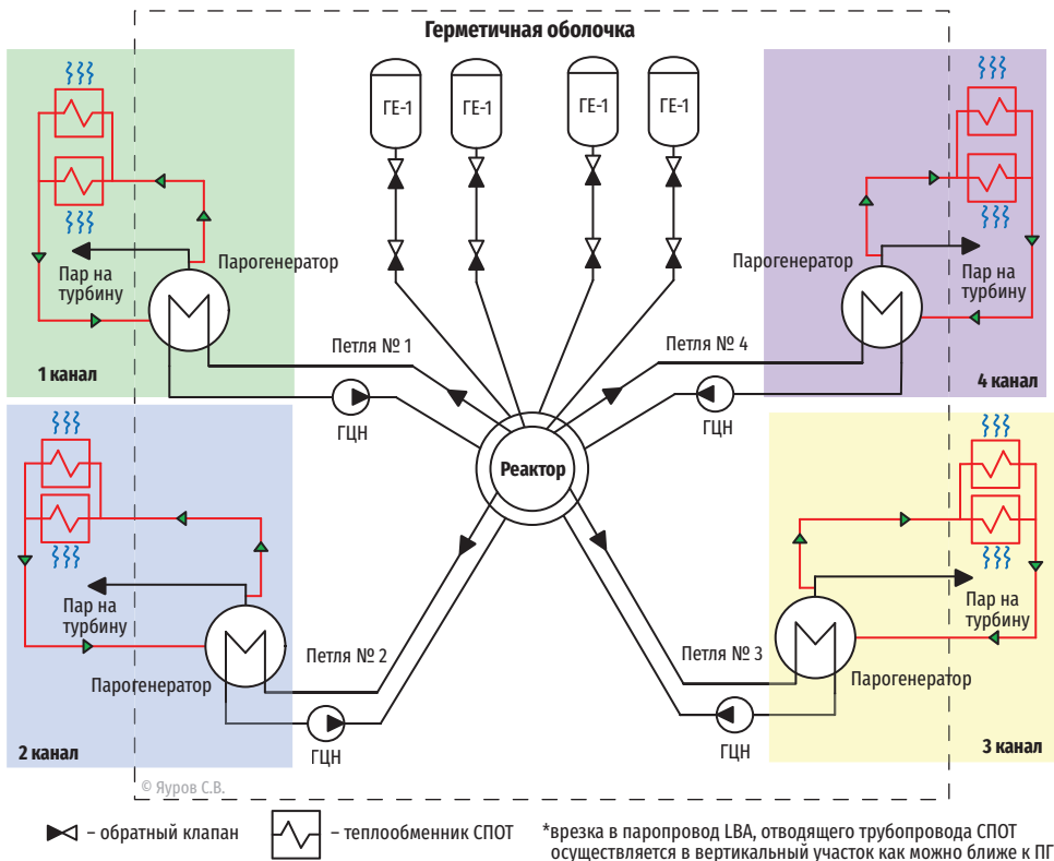
Рис. 2.62. Система пассивного отвода тепла JNB50-80. Проект В-509 (АЭС «Аккую»)
