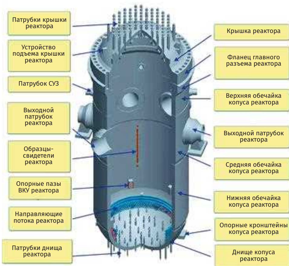
Рис. 3.54. Корпус реактора APR1400 с фланцевой крышкой в разрезе
