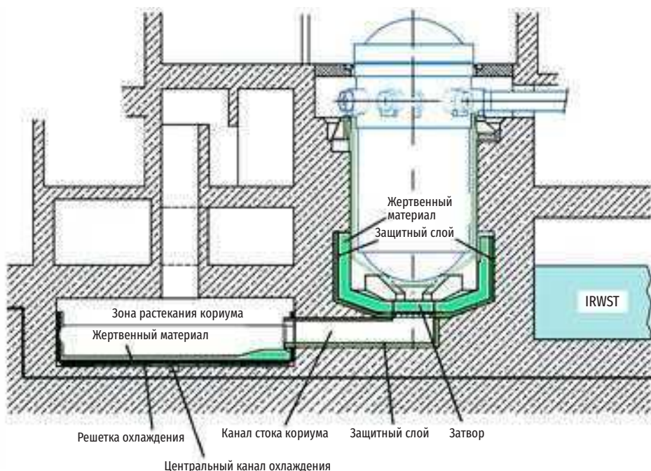
Рис. 3.44. Поперечный разрез конструкций зоны растекания кориума в EPR-1600
