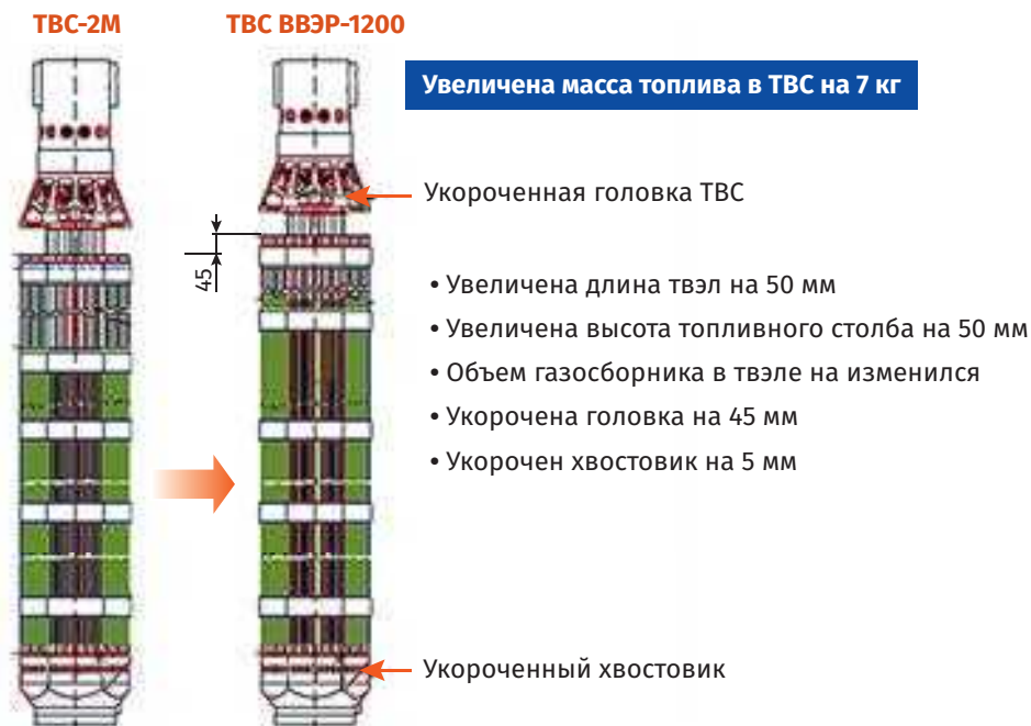
Рис. 2.12. Сравнение конструкций ТВС
