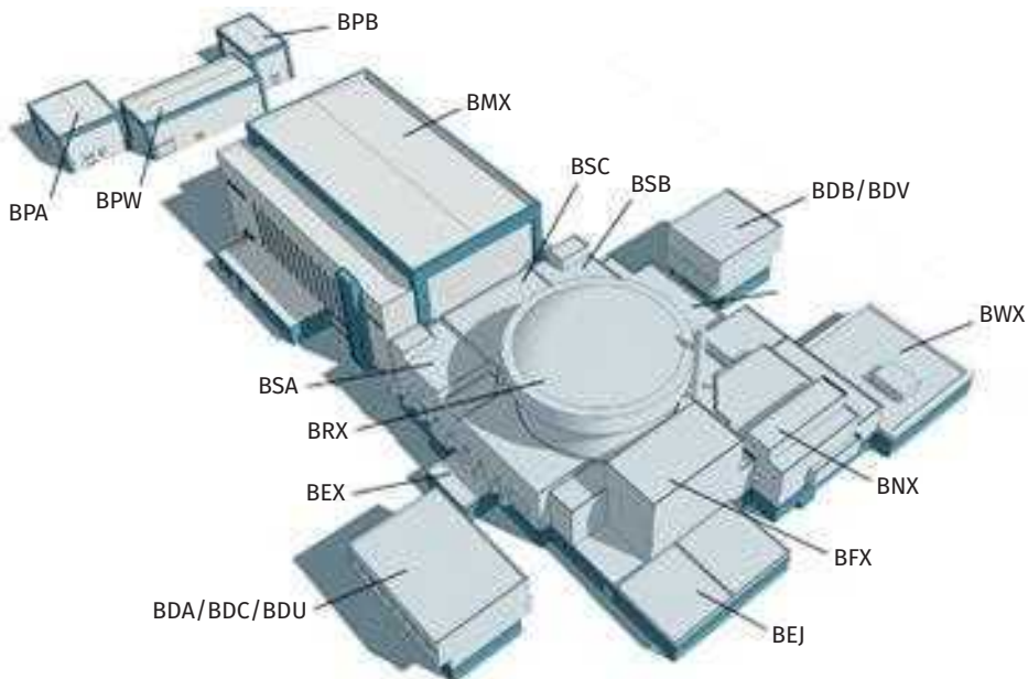
Рис. 3.113. Общий вид площадки для одного блока HPR 1000
