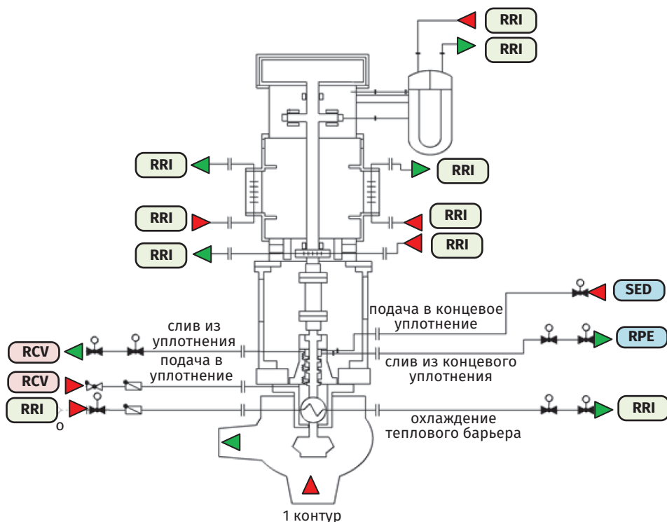
Рис. 3.101. Принципиальная схема систем главного циркуляционного насоса HPR1000.
