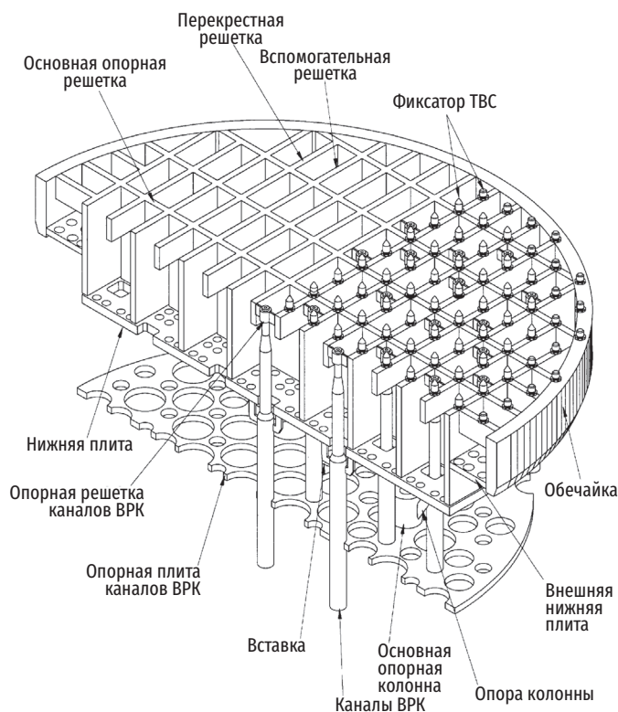
Рис. 3.60. Нижняя опорная конструкция реактора APR1400
