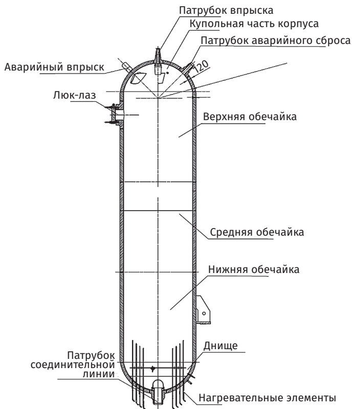
Рис. 3.97. Конструкция компенсатора давления HPR1000
