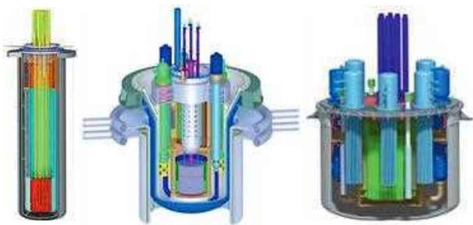
Рис. П2.16. Проекты реакторов серии CLEAR. Слева – CLEAR-A, в центре – CLEAR-M, справа – CLEAR-400
