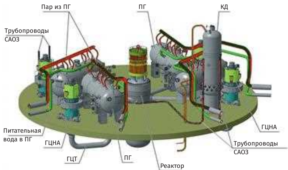
Рис. 2.2. Состав первого контура ВВЭР-1200. Проект В-392М (НВАЭС-2)
