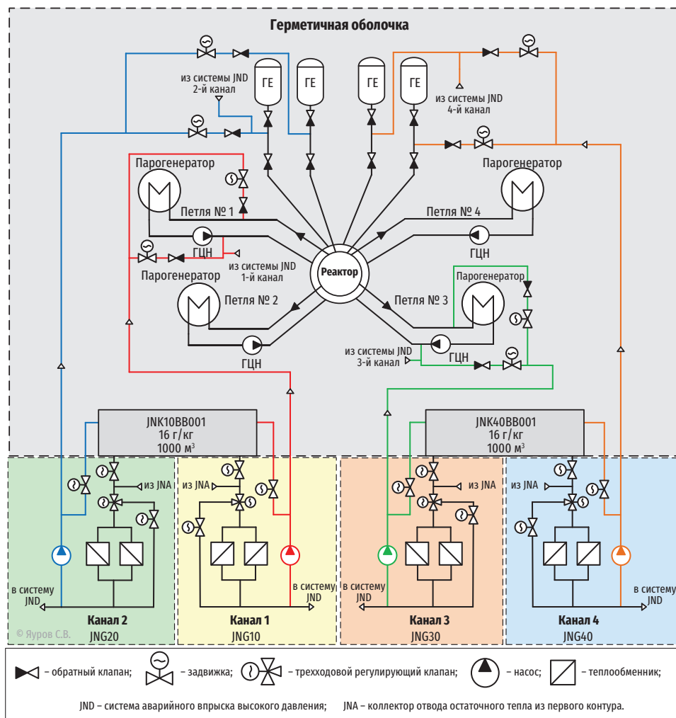
Рис. 2.35. Технологическая схема системы аварийного впрыска низкого давления JNG-1. Проект В-491 (ЛАЭС-2)
