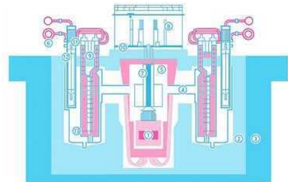
Рис. П2.11. Конструкция РУ БРЕСТ-ОД-300 (вид сбоку).
