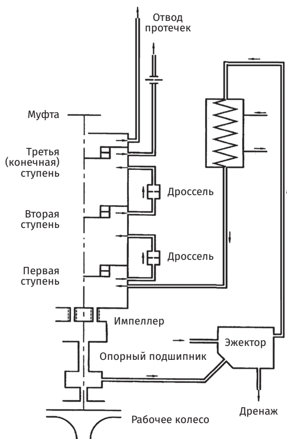
Рис. 3.67. Принципиальная схема узла уплотнения вала ГЦН APR1400
