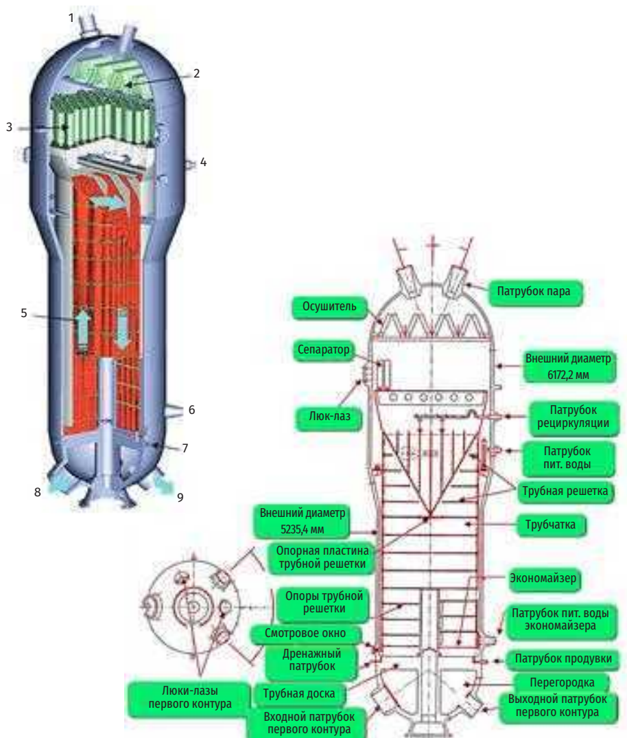
Рис. 3.69. Устройство парогенератора APR1400 и направление потока теплоносителя первого контура в теплообменных трубках.
