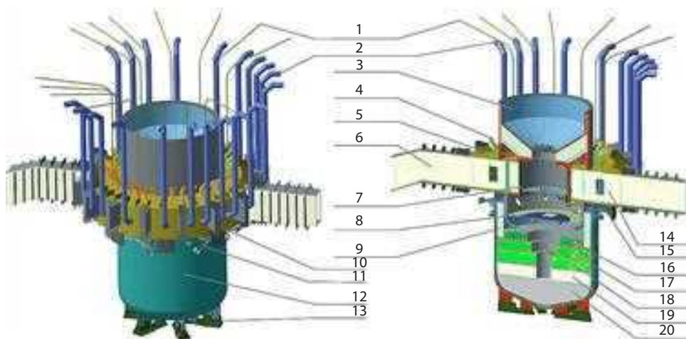
Рис. 2.29. Устройство локализации расплава активной зоны АЭС-2006.
