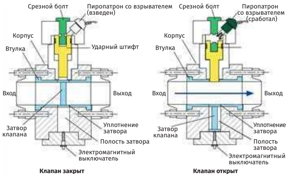
Рис. 3.11. Принцип действия пиропатронного клапана компенсатора в 4-й группе предохранительных клапанов системы компенсации давления в АР1000
