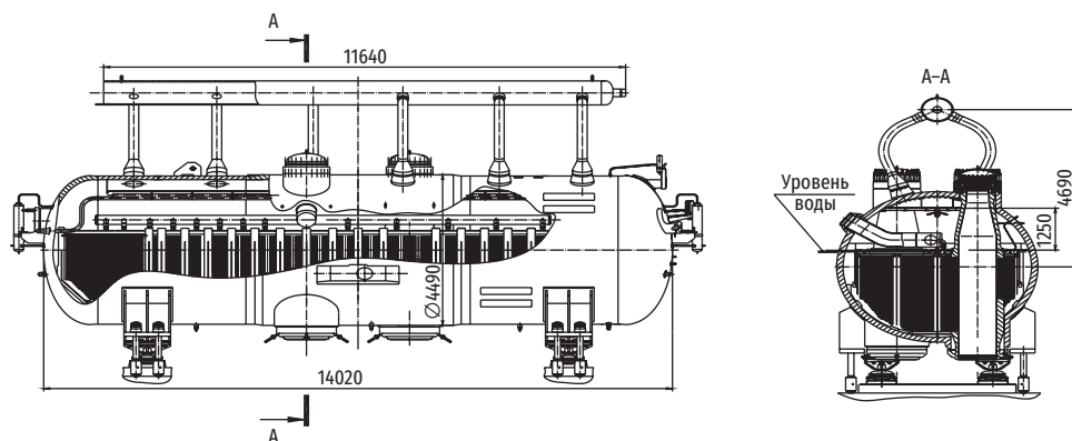
Рис. 2.80. Парогенератор ПГВ-1200МР
