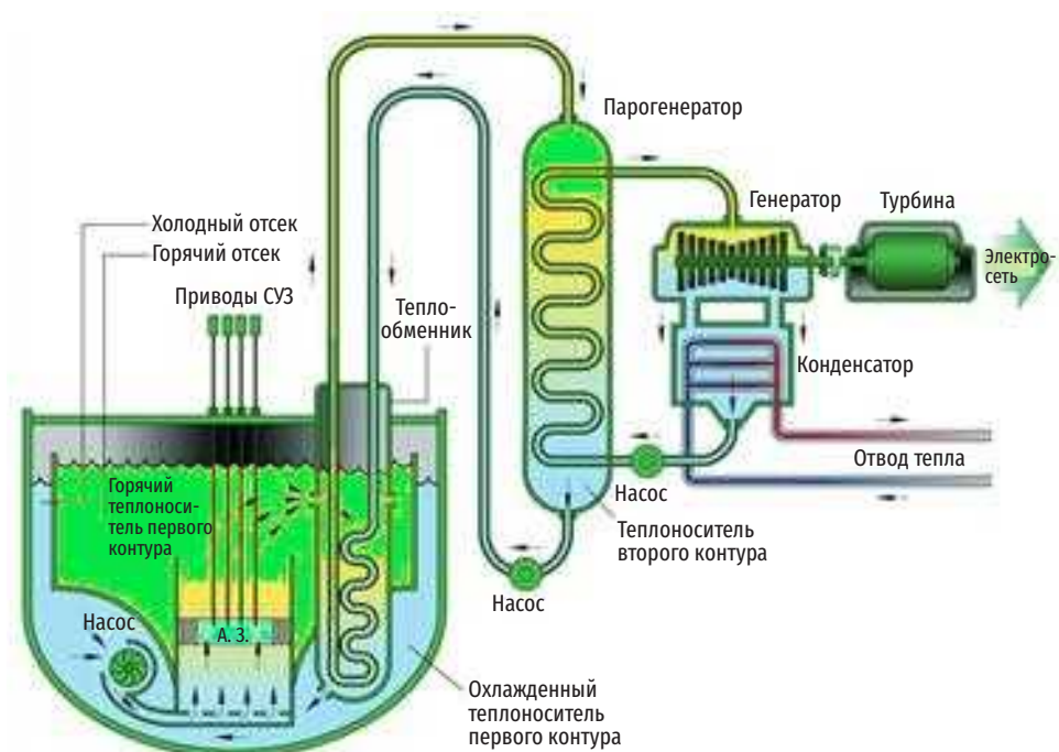
Рис. П2.22. Тепловая схема реактора на быстрых нейтронах с натриевым теплоносителем SFR
