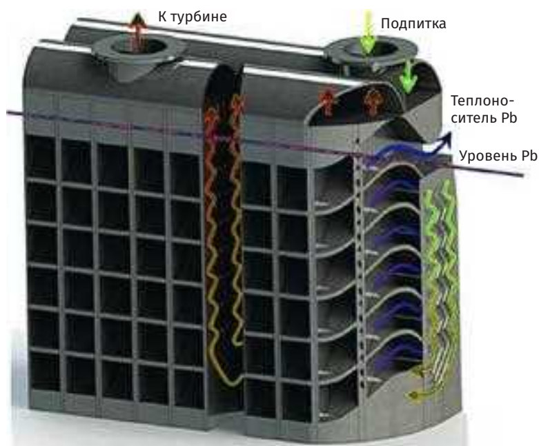
Рис. П2.21. Схематический вид компактного гибридного микроканального теплообменника СНМ РНХ
