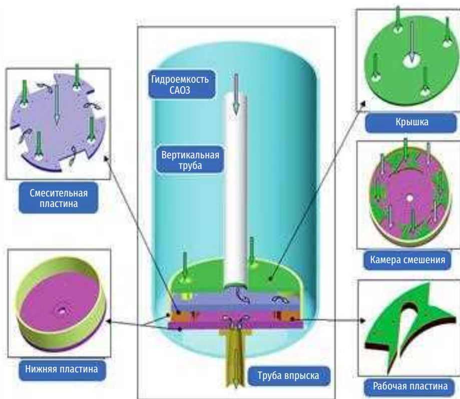
Рис. 3.72. Конструкция и элементы устройства профилирования потока (FD)
