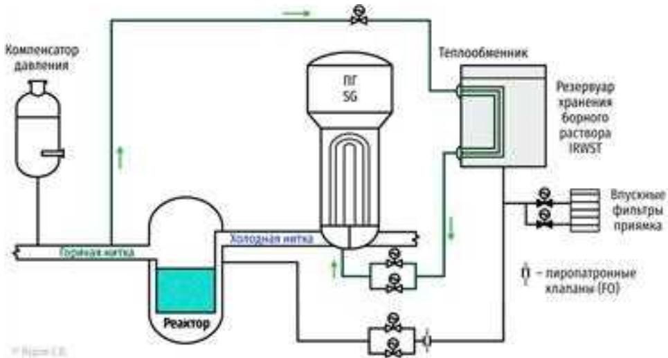
Рис. 3.18. Принципиальная схема пассивного отвода остаточного тепла активной зоны в проекте AP1000
