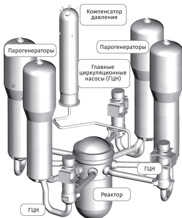
Рис. 3.25. Компоновка основного оборудования реакторной установки EPR-1600
