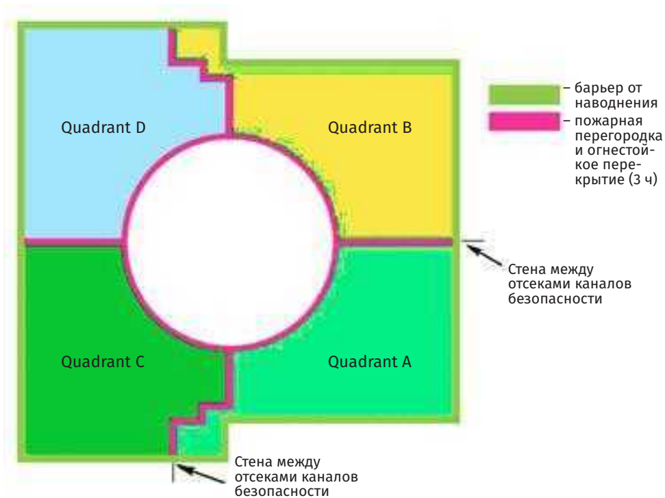
Рис. 3.83. Схема физических барьеров безопасности здания АВ APR1400
