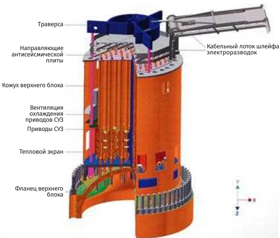
Рис. 3.91. Общий вид конструкций верхнего блока реактора HPR1000
