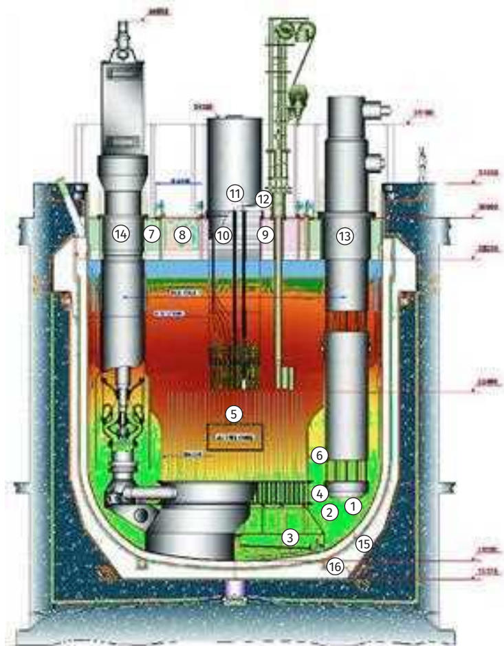
Рис. П2.25. Продольный разрез корпуса PFBR.
