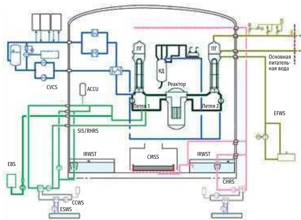
Рис. 3.40. Упрощенная схема конфигурации одного канала систем безопасности EPR-1600.
