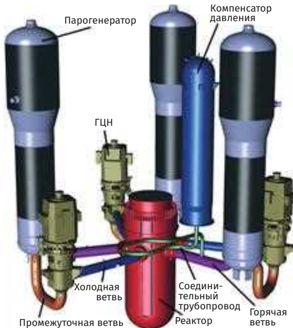
Рис. 3.85. Общий вид основного оборудования реакторной установки HPR1000
