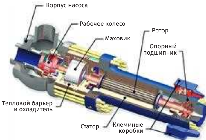
Рис. 3.12. Главный циркуляционный насос реактора AP1000
