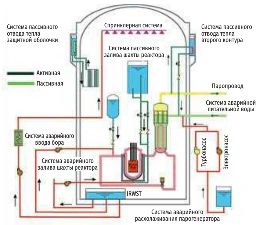
Рис. 3.104. Схема активных и пассивных систем безопасности HPR1000
