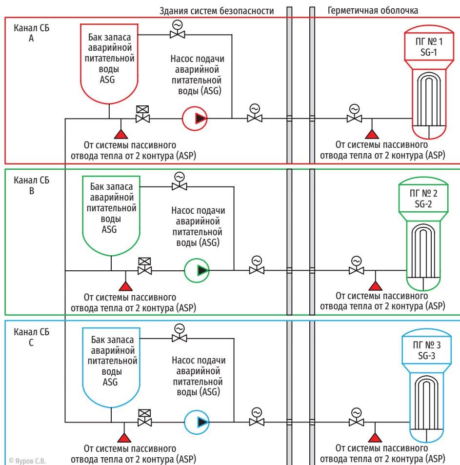
Рис. 3.108. Принципиальная схема аварийной системы питательной воды ПГ HPR1000 [ASG (EFWS)]
