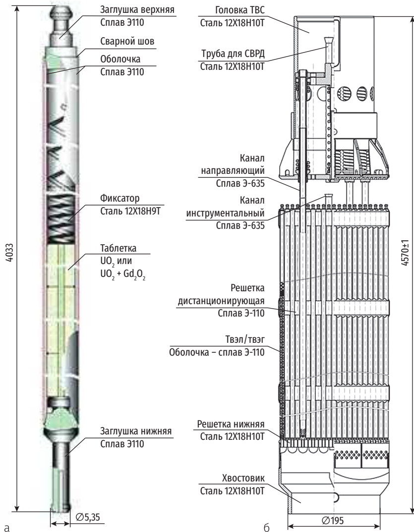
Рис. 2.11. Конструкция элементов активной зоны. Проект В-392М (НВАЭС-2).
