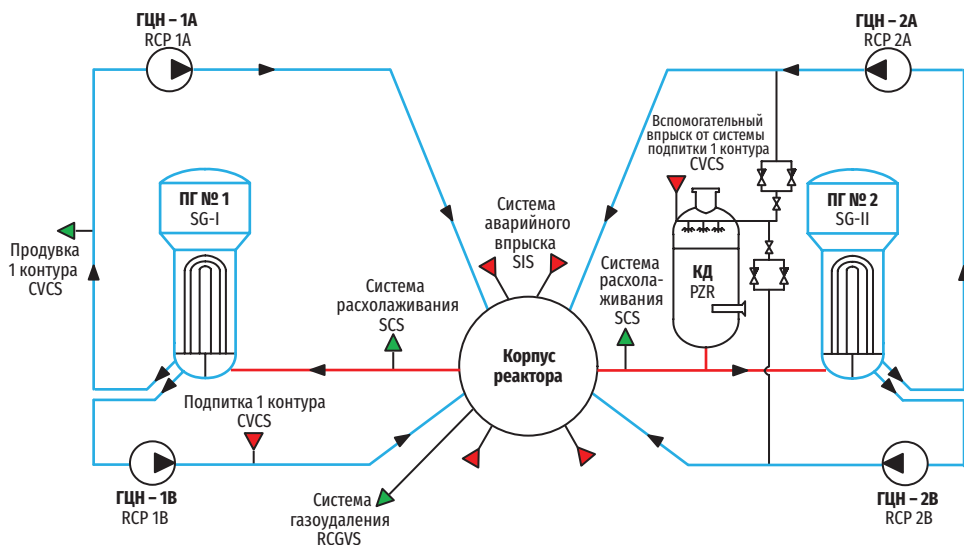
Рис. 3.51. Принципиальная схема первого контура APR1400
