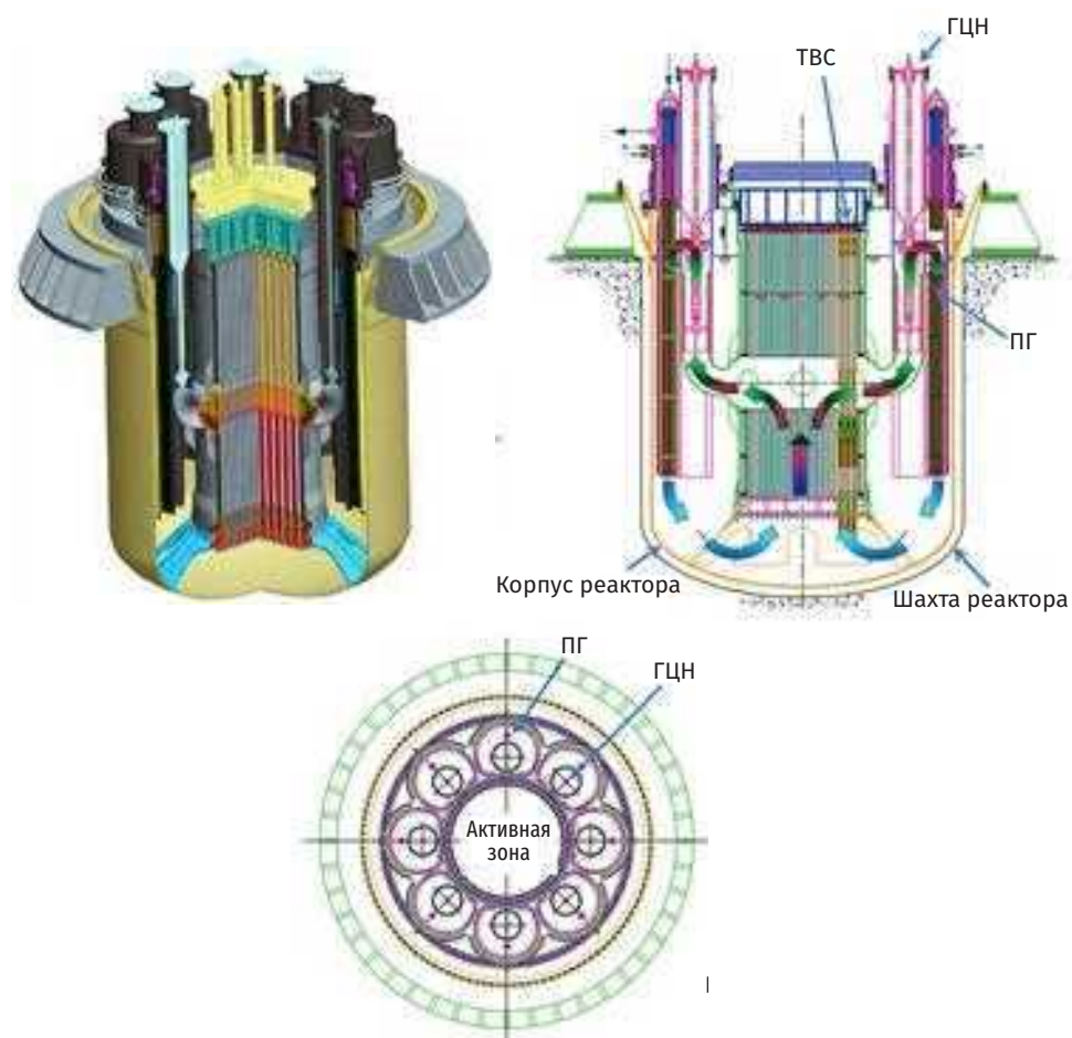
Рис. П2.13. Конструкция РУ ALFRED (проект LEADER) и контуры циркуляции теплоносителя в первом контуре
