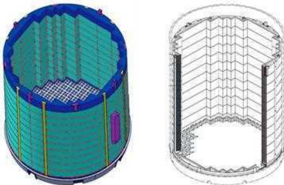
Рис. 3.30. Общий вид и секторальный разрез выгородки-отражателя EPR-1600
