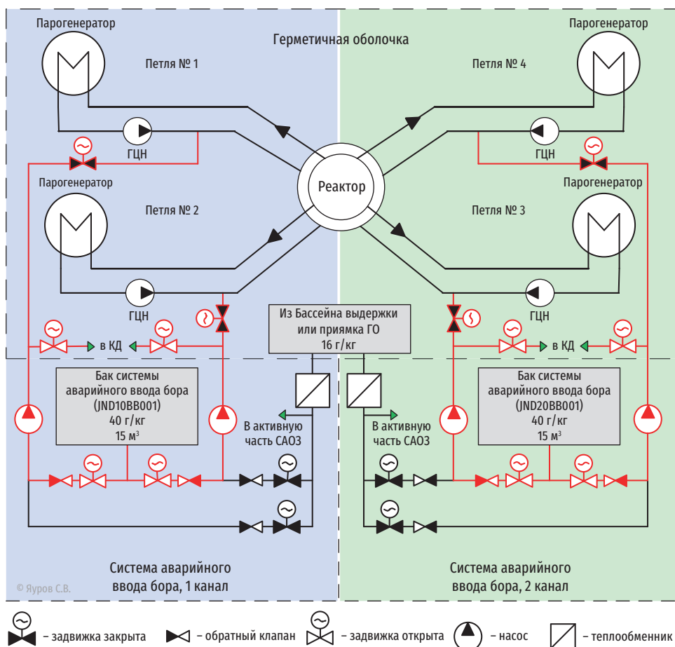
Рис. 2.22. Система аварийного ввода бора JND. Проект В-392М (НВАЭС-2)
