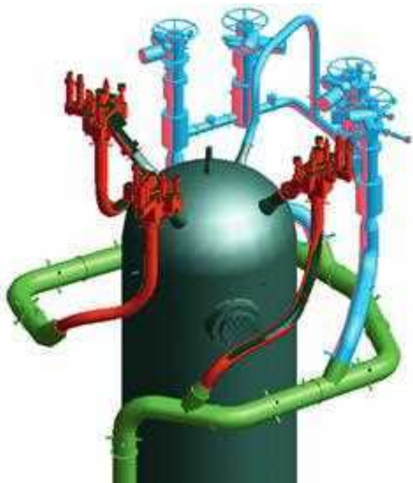
Рис. 3.99. Общий вид предохранительных и защитных клапанов КД (PSV, SADV) HPR1000
