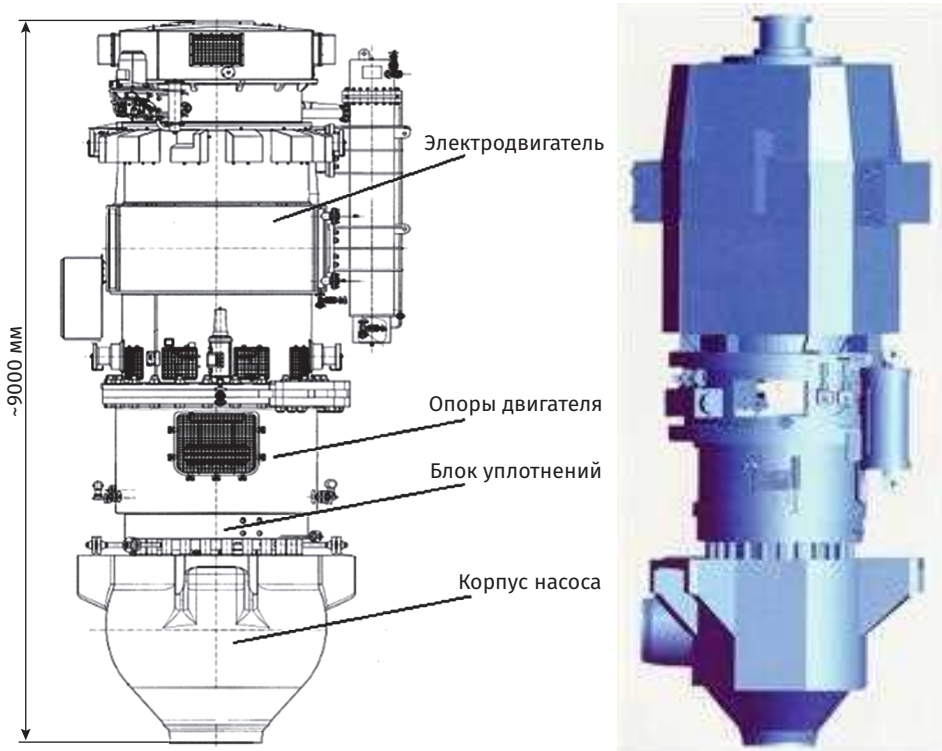
Рис. 3.100. Конструкция главного циркуляционного насоса HPR1000
