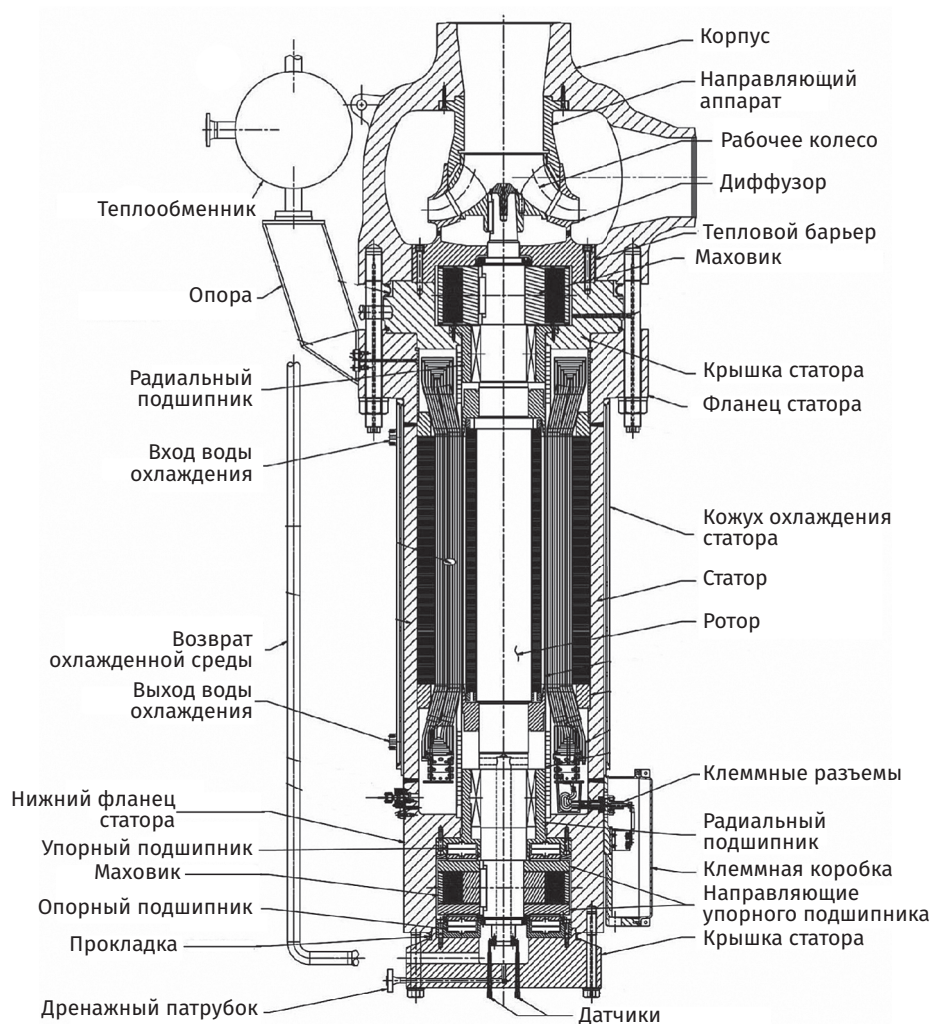
Рис. 3.13. Конструкция главного циркуляционного насоса реактора AP1000
