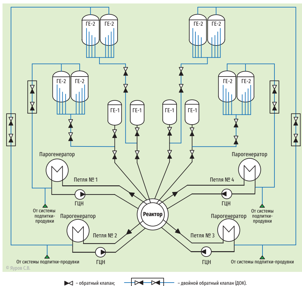
Рис. 2.24. Упрощенная схема пассивной части САОЗ. Проект В-392М (НВАЭС-2)
