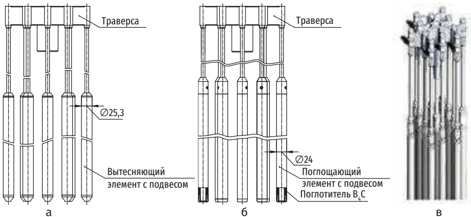
Рис. 2.78. Конструкция ВС СУЗ и ПС СУЗ.
