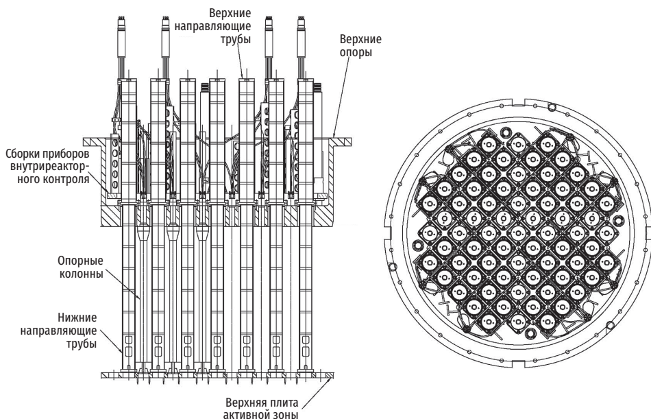
Рис. 3.6. Верхняя опорная конструкция активной зоны реактора AP1000
