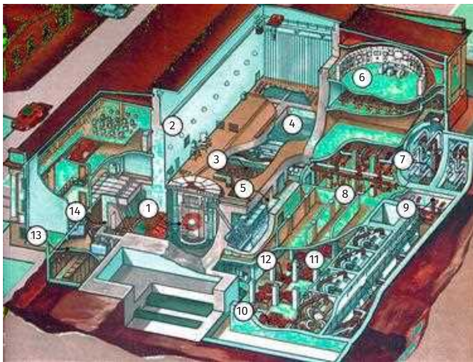
Рис. 1.6. Конструкция Обнинской АЭС.
