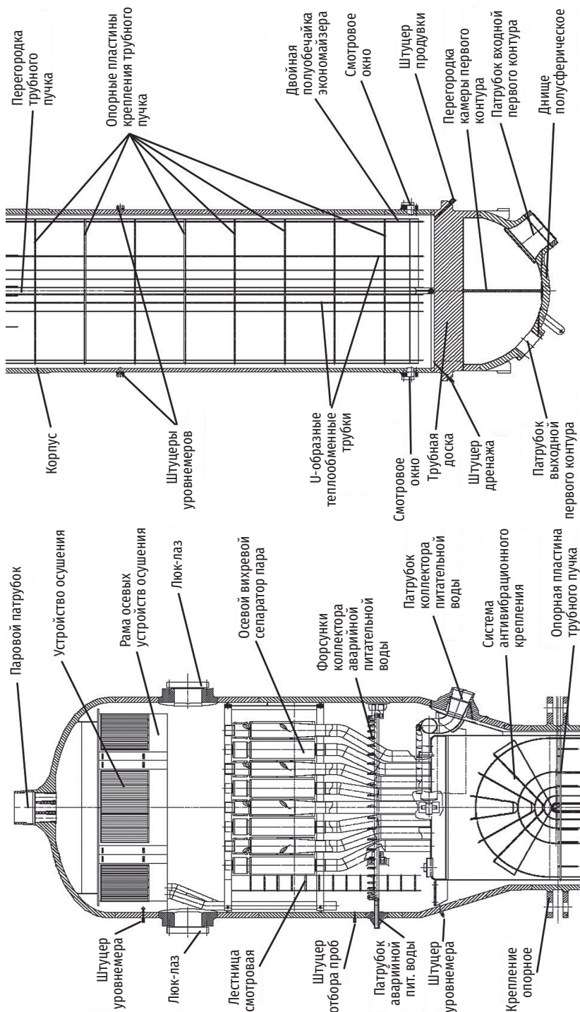
Рис. 3.39. Парогенератор EPR-1600 в разрезе
