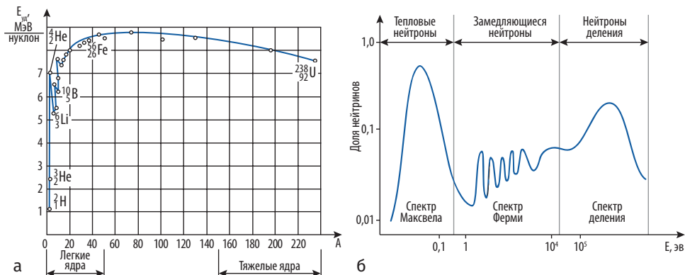
Рис. 1.2. Зависимость удельной энергии связи ядер от массового числа A (а); спектр нейтронов (б)
