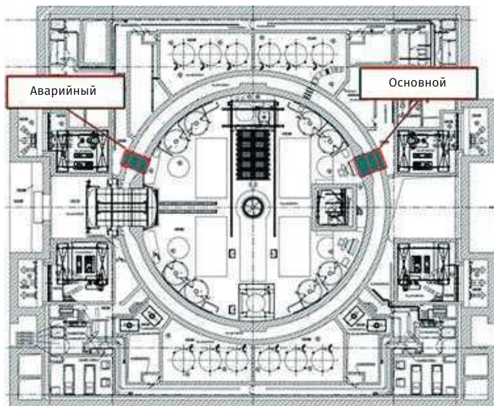
Рис. 2.67. Расположение шлюзов доступа персонала в реакторное здание проекта В-509 АЭС «Аккую»
