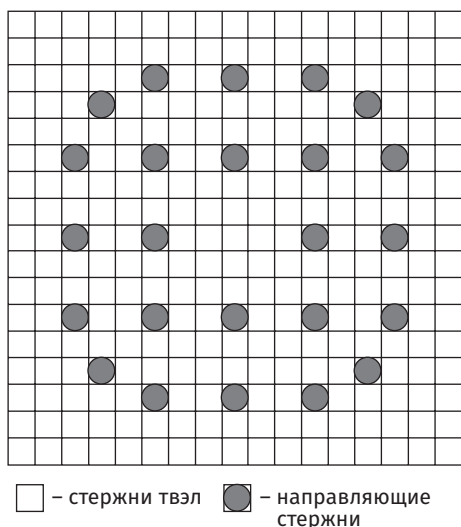
Рис. 3.32. Картограмма размещения твэл в решетке ТВС EPR-1600
