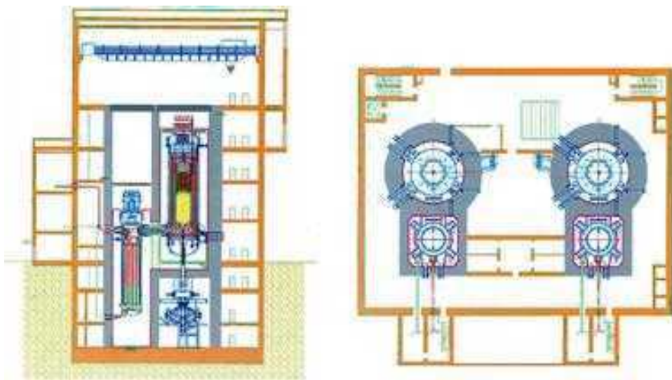
Рис. П2.44. Реакторное здание с размещением двух модулей реакторной установки HTR-PM
