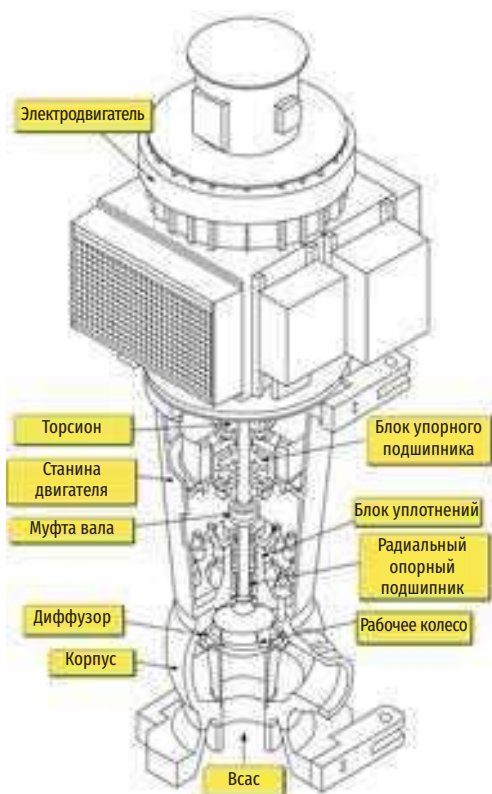
Рис. 3.66. Основные компоненты конструкции ГЦН APR1400
