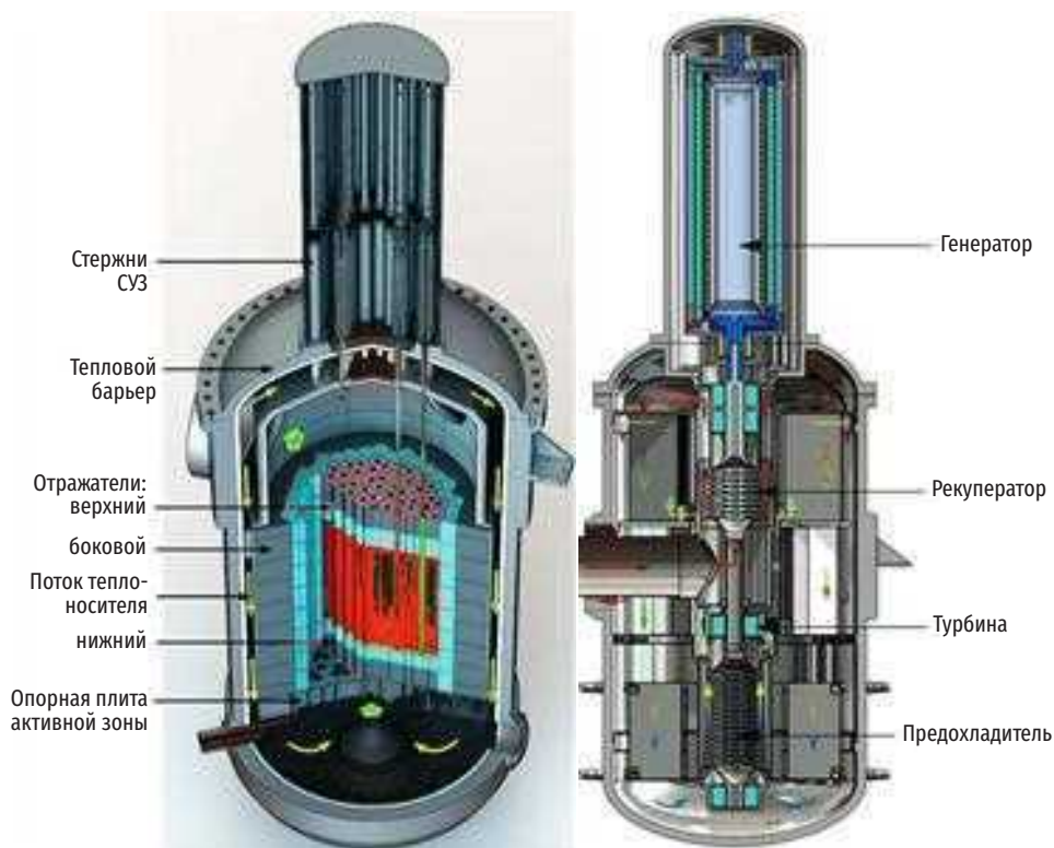
Рис. П2.8. Конструкция реакторной установки с потоками теплоносителя (слева), блока преобразования энергии (справа) в проекте EM 2
