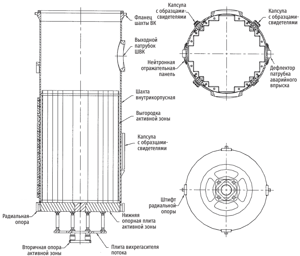
Рис. 3.5. Конструкция нижнего внутрикорпусного устройства реактора AP1000
