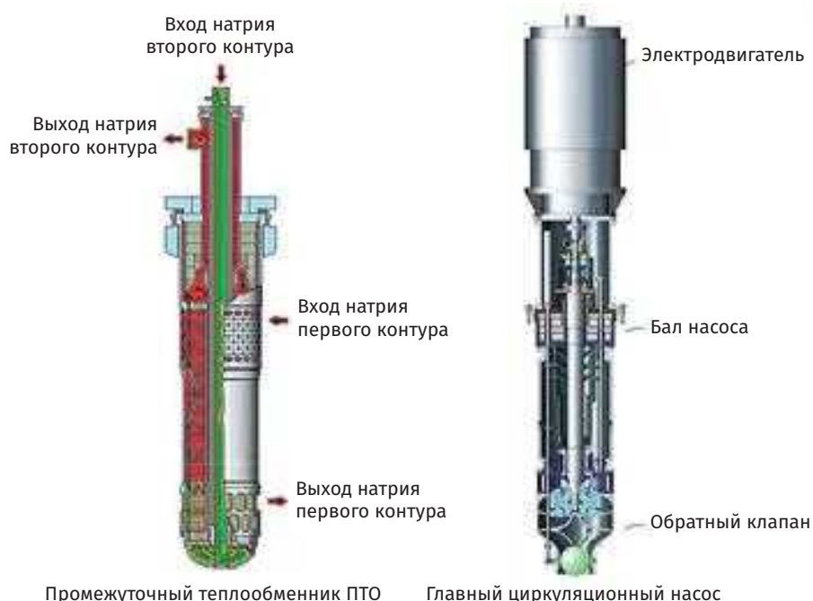
Рис. П2.28. Конструкция промежуточного теплообменника и главного циркуляционного насоса реактора БН-800
