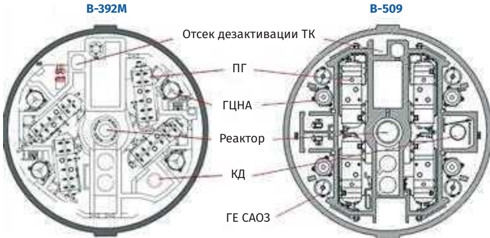
Рис. 2.68. Компоновка оборудования 1 контура проекта В-509 АЭС «Аккую» и проекта В-392М (НВАЭС-2)
