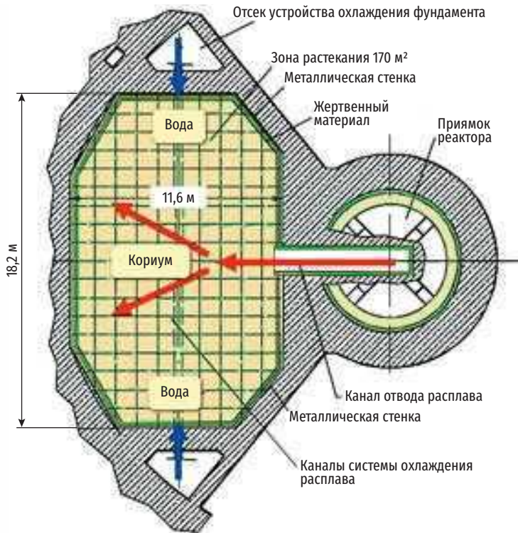
Рис. 3.43. Принцип действия системы стабилизации расплава активной зоны EPR-1600
