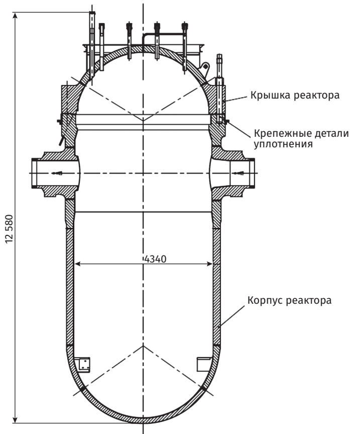
Рис. 3.90. Конструкция корпуса реактора HPR1000
