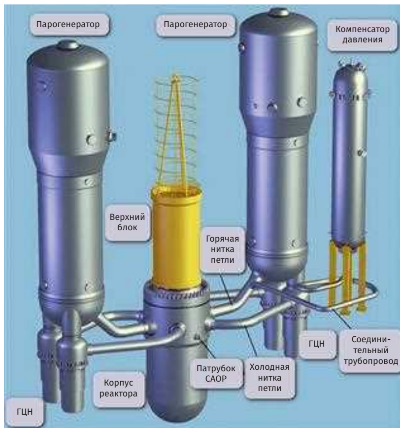
Рис. 3.1. Общий вид оборудования первого контура AP1000
