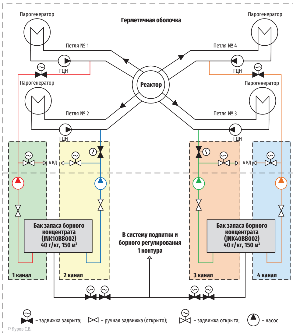
Рис. 2.34. Структура системы аварийного ввода бора JDN. Проект В-491 (ЛАЭС-2)
