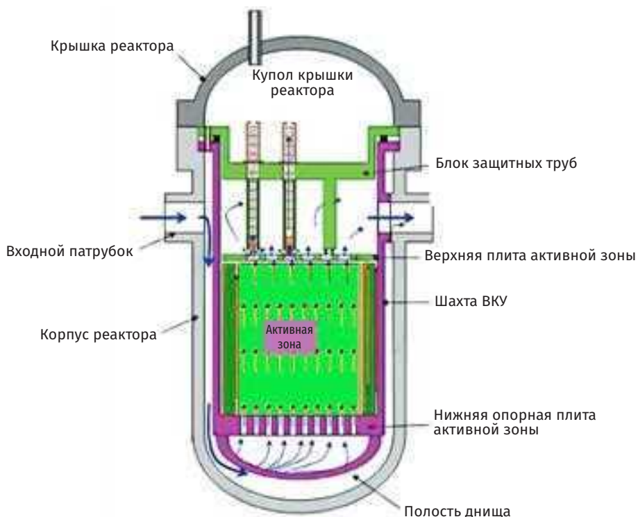
Рис. 3.89. Схема потоков теплоносителя в реакторе HPR1000
