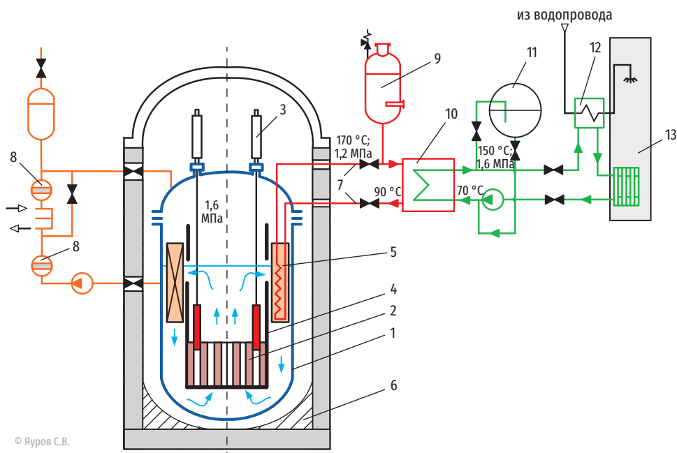
Рис. 1.25. Принципиальная схема реакторной установки АСТ-500.
