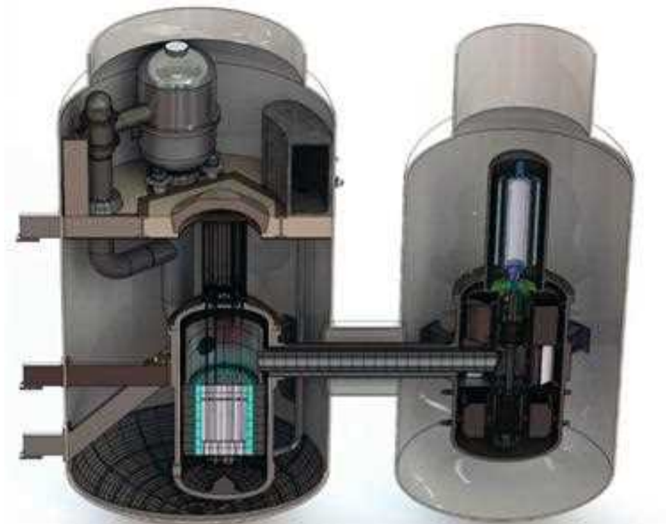
Рис. П2.7. Первый контур реакторной установки в двухкорпусном контейнменте (слева – реактор с системой прямого охлаждения, справа – интегральный турбогенераторный агрегат)
