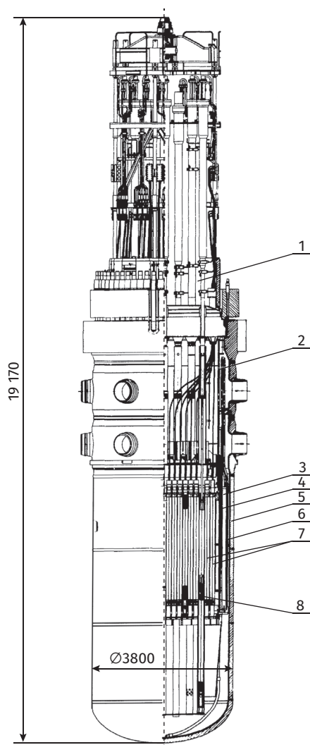
Рис. 1.8. Реактор В-1 (ВВЭР-210).
