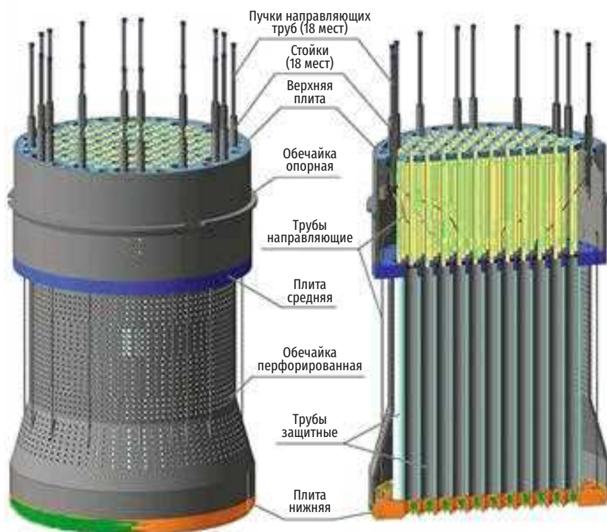
Рис. 2.8. Блок защитных труб реактора ВВЭР-1200. Проект В-392М (НВАЭС-2)
