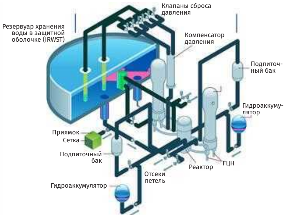
Рис. 3.16. Пассивная система охлаждения активной зоны (PXS) проекта AP1000
