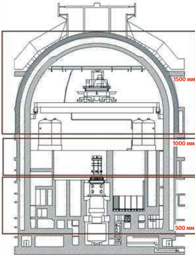
Рис. 2.66. Реакторное здание проекта В-509 АЭС «Аккую»
