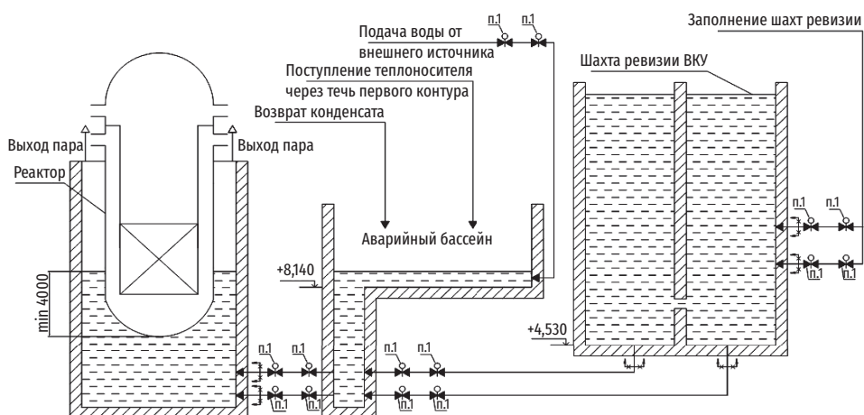
Рис. 2.83. Принципиальная гидравлическая схема подачи воды в шахту реактора
