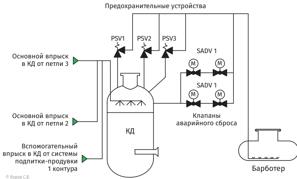
Рис. 3.98. Принципиальная схема системы поддержания давления первого контура HPR1000
