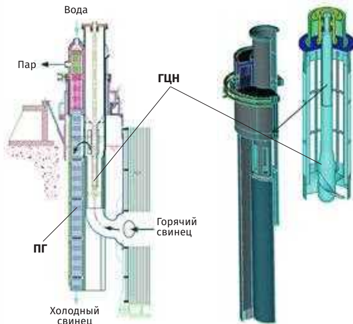
Рис. П2.15. Конструкция интегральной сборки ГЦН-ПГ реактора ALFRED
