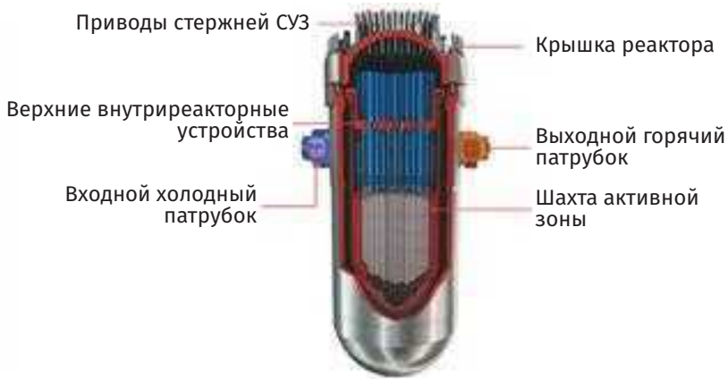
Рис. 3.87. Общий вид корпуса реактора с ВКУ HPR1000
