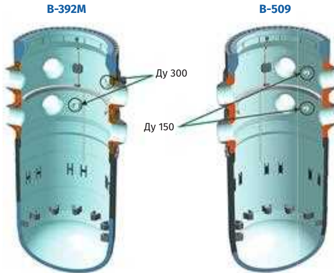
Рис. 2.51. Патрубки ГЕ САОЗ в реакторах проектов В-392М и В-509
