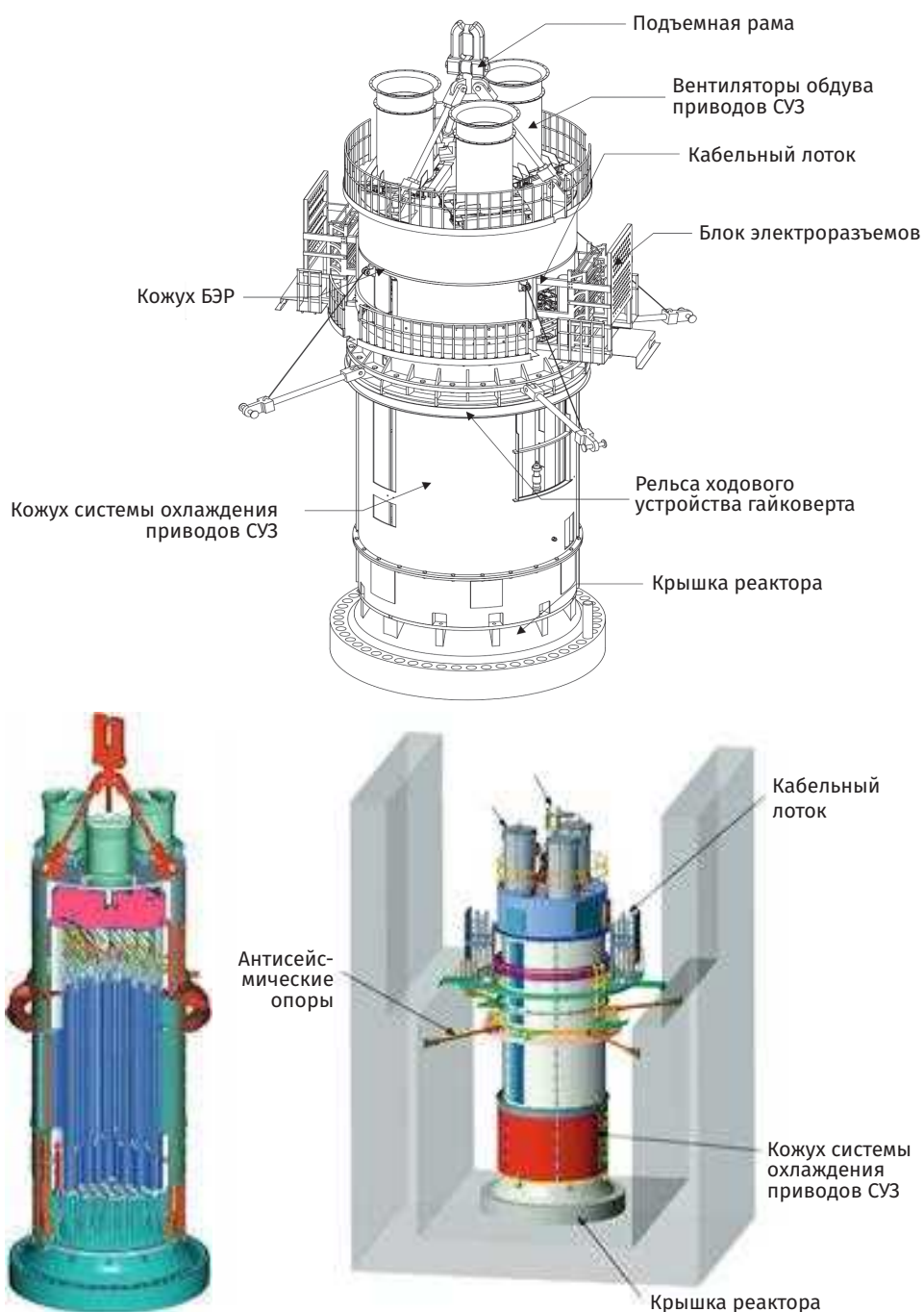
Рис. 3.55. Верхний блок реактора APR1400 с интегрированными системами в сборе с крышкой реактора
