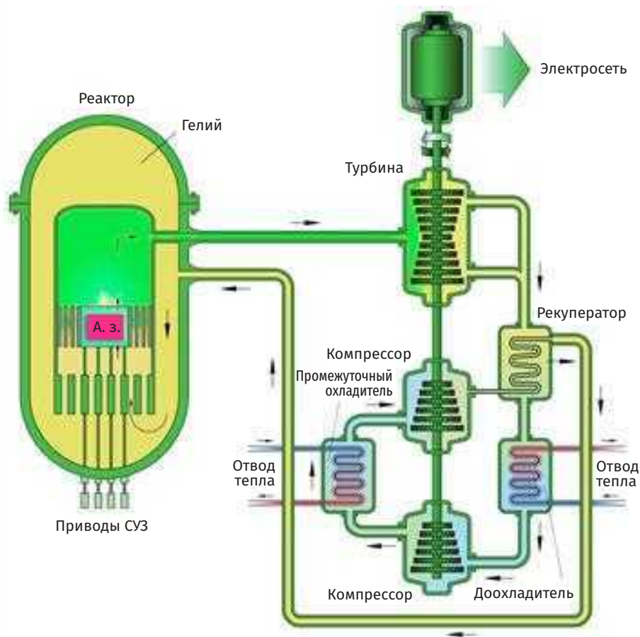
Рис. П2.3. Тепловая схема газоохлаждаемого реактора на быстрых нейтронах GFR
