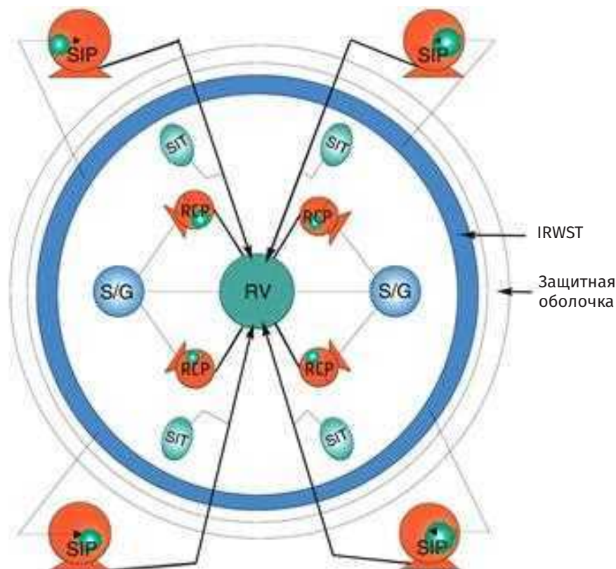
Рис. 3.71. Блок-схема каналов системы аварийного впрыска (SIS) APR1400.
