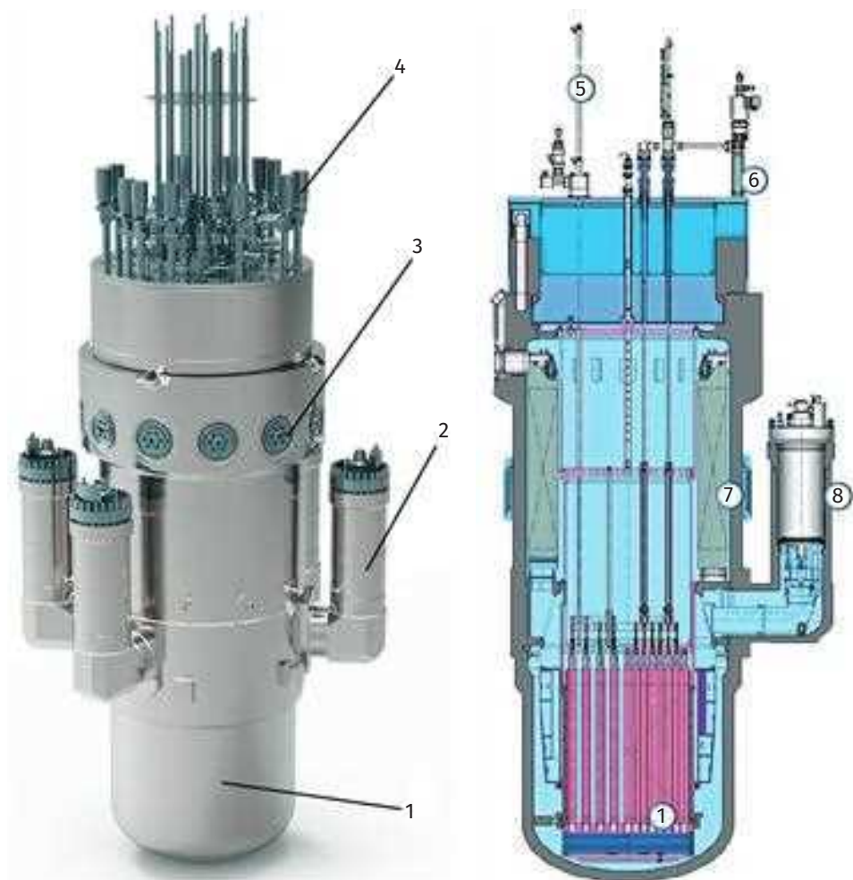
Рис. 1.22. Интегральный реактор РИТМ-200Н.
