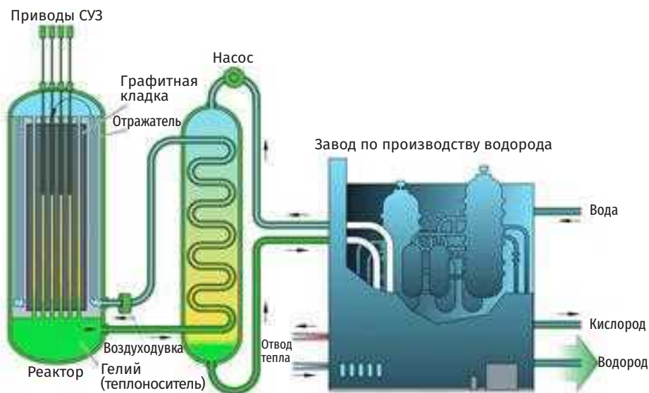
Рис.П2.39. Тепловая схема высокотемпературного газового реактора VHTR для производства водорода
