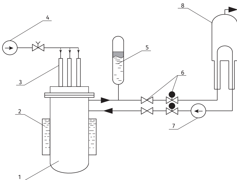
Рис. 1.10. Принципиальная схема РУ В-2 (ВВЭР-70).
