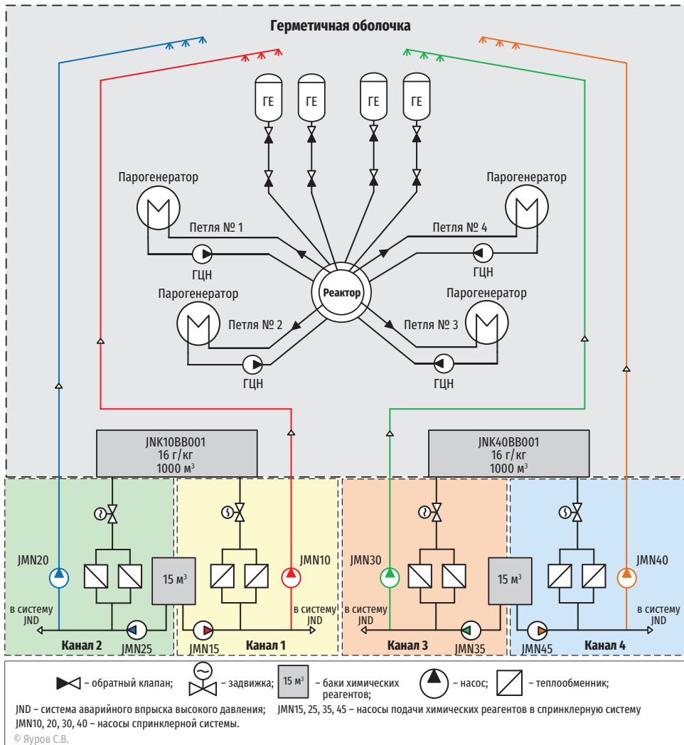
Рис. 2.41. Упрощенная схема спринклерной системы с баками химреагентов. Проект В-491 (ЛАЭС-2)
