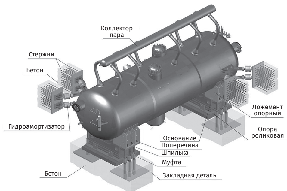
Рис. 2.18. Состав парогенератора ПГВ-1000МКП
