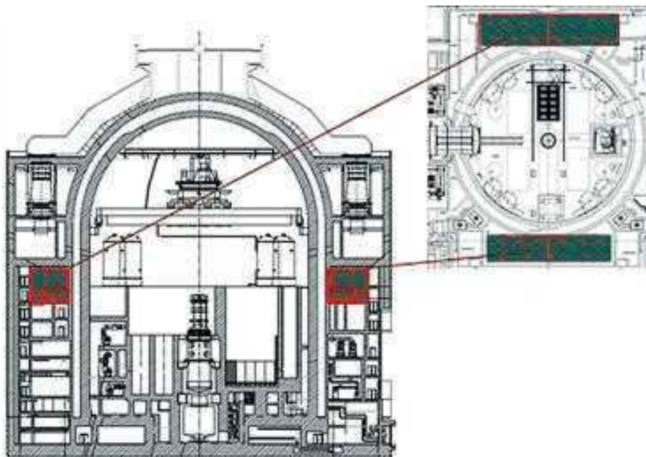
Рис. 2.60. Размещение GE-3 SAO3, проект В-509 (АЭС «Аккую»)
