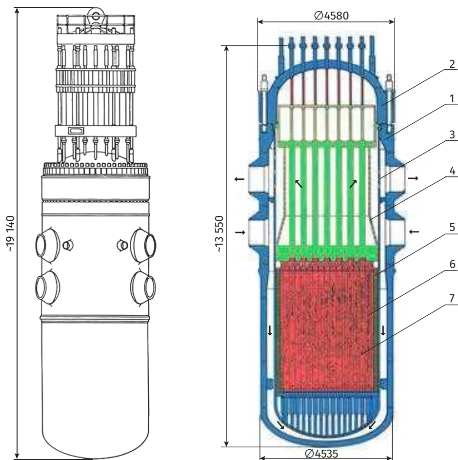
Рис. 1.13. Реактор ВВЭР-1000.
