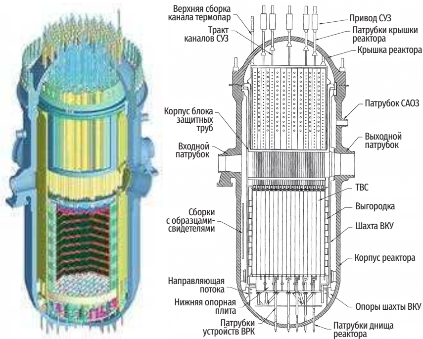
Рис. 3.52. Общий вид реактора APR1400 и внутрикорпусных устройств в разрезе
