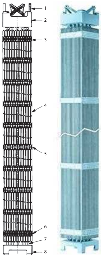
Рис. 3.33. Конструкция тепловыделяющих сборок. Радиальное поперечное сечение тепловыделяющей сборки и общий вид ТВС EPR-1600.
