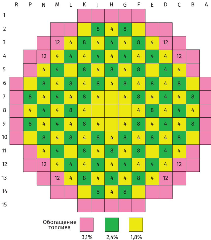
Рис. 3.93. Картограмма размещения в активной зоне ТВС с различной степенью обогащения топлива при начальной загрузке в реакторе HPR1000
