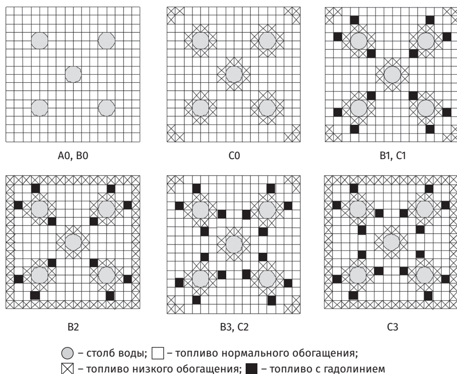
Рис. 3.63. Картограмма матриц TBC различных типов реактора APR1400
