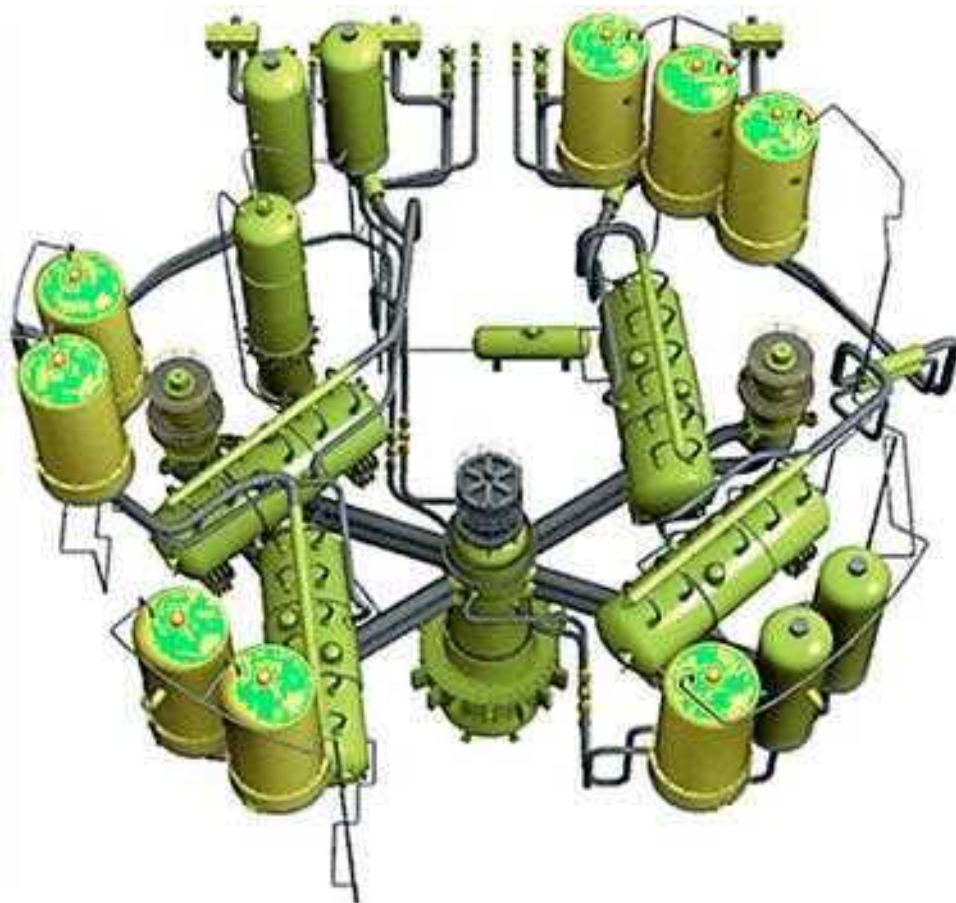
Рис. 1.15. Установка реакторная ВВЭР-1200. Проект В-392М (НВАЭС-2)
