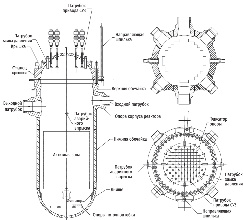
Рис. 3.4. Корпус реактора AP1000
