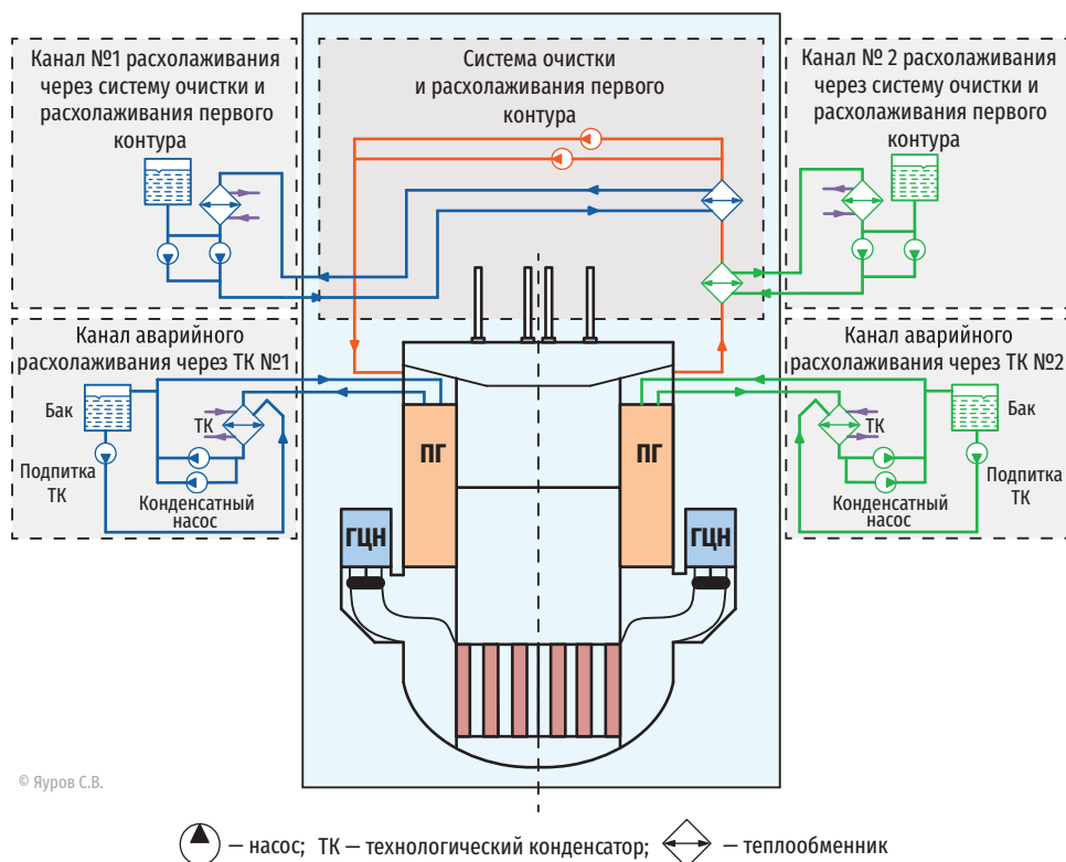
Рис. 1.23. Принципиальная схема активных каналов расхолаживания. РУ РИТМ-200Н
