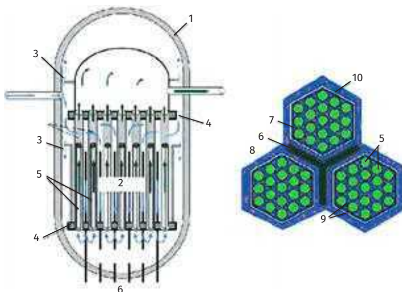
Рис. П2.32. Реактор SCWR INEEL – второй вариант реактора.
