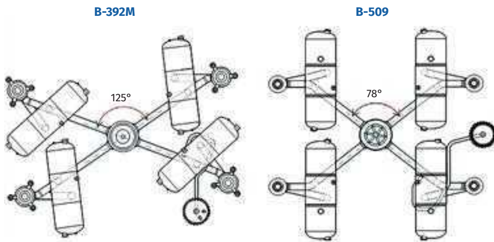
Рис. 2.49. Компоновка петель 1 контура проекта В-509 АЭС «Аккую» и проекта В-392М (НВАЭС-2)
