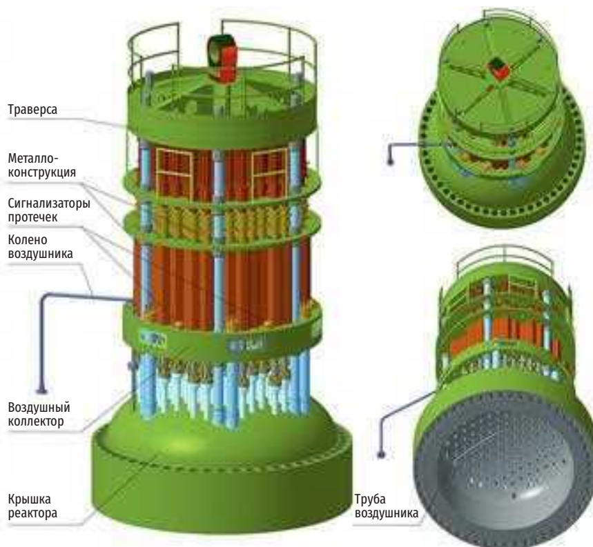
Рис. 2.9. Верхний блок реактора ВВЭР-1200. Проект В-392М (НВАЭС-2)
