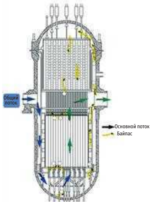
Рис. 3.52. Общий вид реактора APR1400 и внутрикорпусных устройств в разрезе
