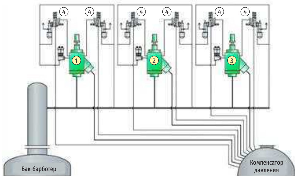
Рис. 3.36. Схема подключения импульсных предохранительных устройств компенсатора давления EPR-1600.
