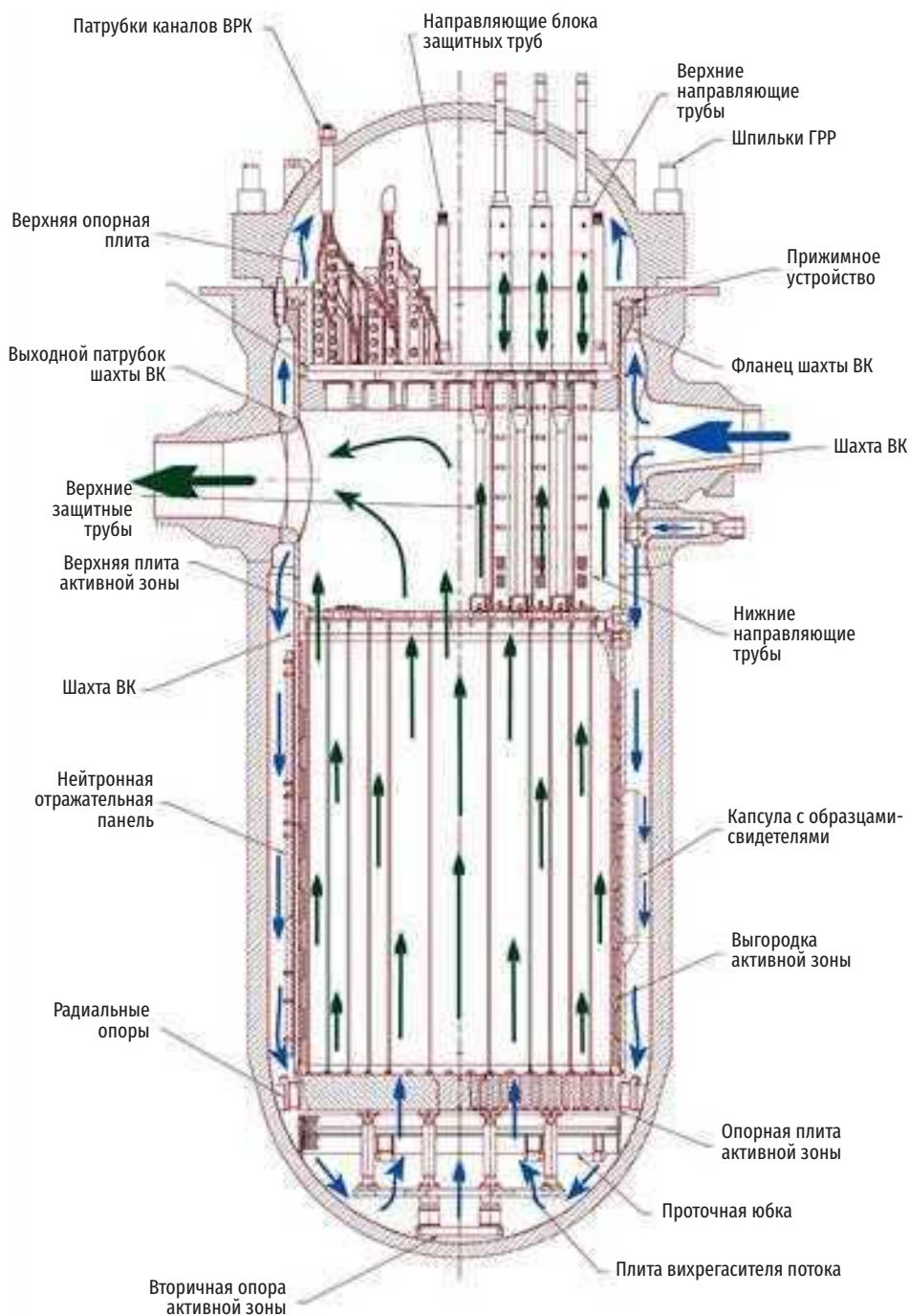
Рис. 3.3. Конструкция реактора AP1000
