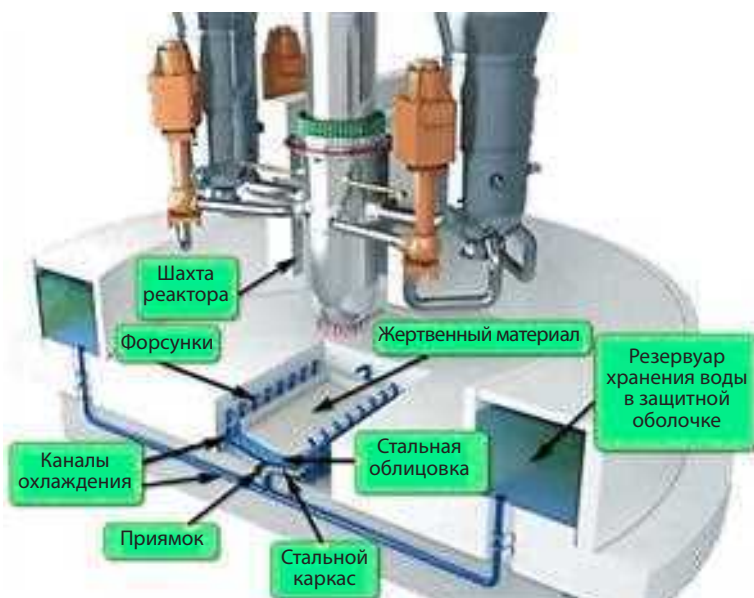
Рис. 3.81. Конструкция камеры для локализации расплава активной зоны реактора проекта EU-APR1400
