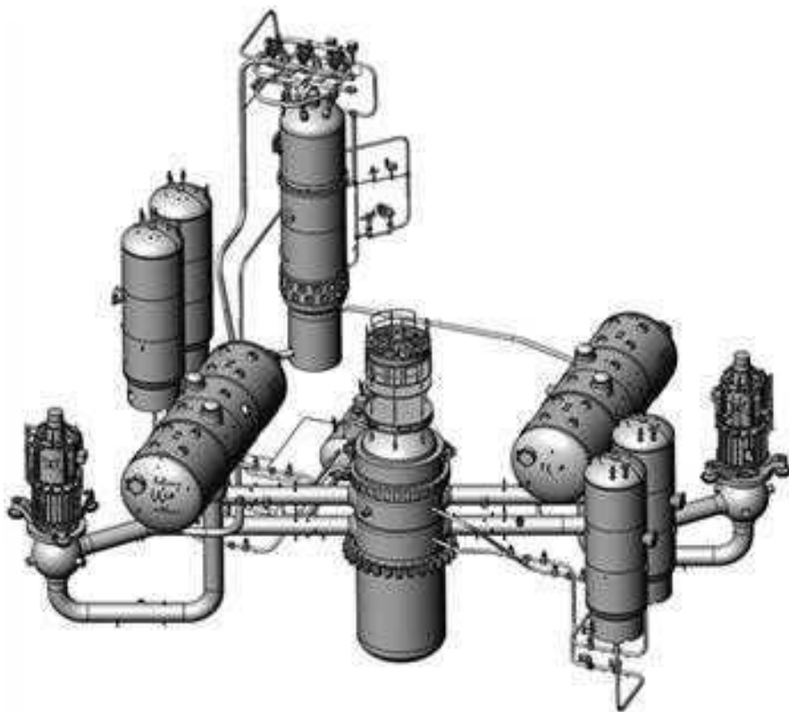
Рис. 2.74. Общий вид оборудования первого контура РУ В-551С
