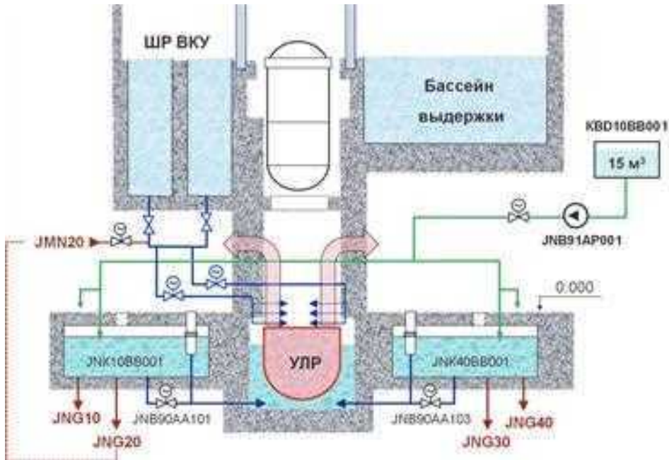
Рис. 2.43. Схема аварийного использования воды из шахты ревизии ВКУ. Проект В-491 (ЛАЭС-2)
