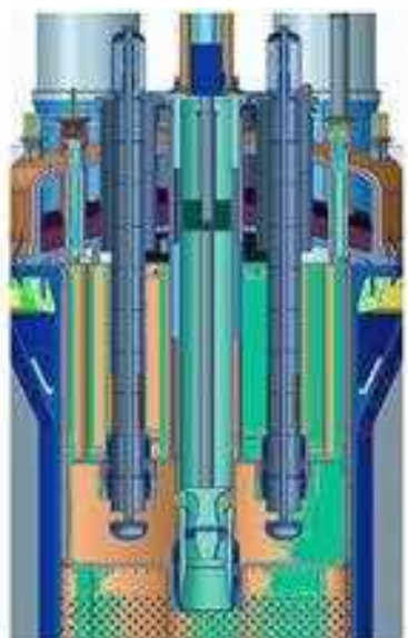
Рис. П2.19. Конструкция испытательной установки COMPLOT проекта MYRRHA ADS
