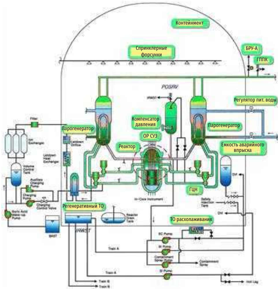
Рис. 3.70. Блок-схема систем безопасности РУ APR1400
