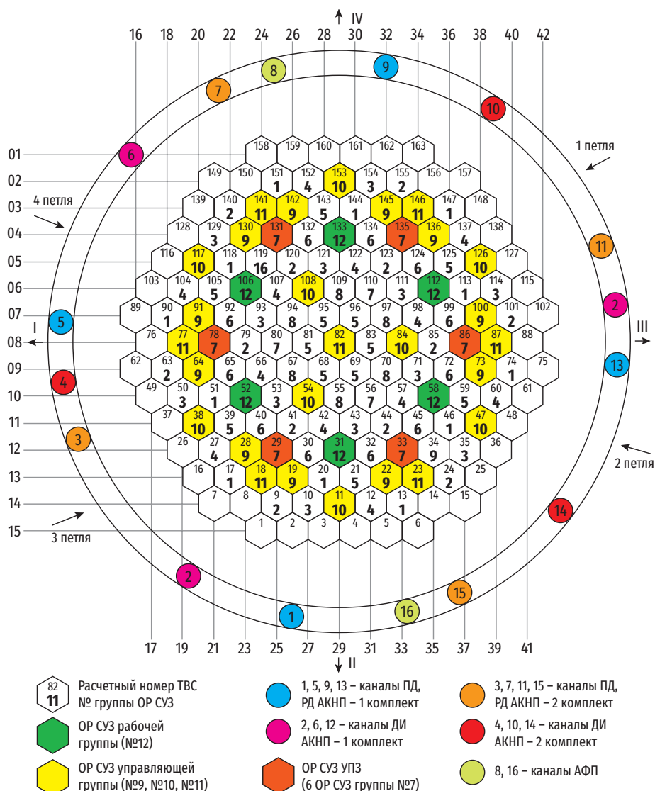
Рис. 2.14. Энергоблок № 1 НВАЭС-2: картограмма активной зоны, распределение ОР СУЗ по группам, схема расположения каналов АКНП
