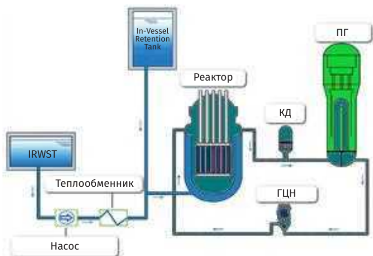
Рис. 3.112. Схема аварийного заполнения реакторной шахты и охлаждения корпуса реактора [ECS (ECS)] РУ HPR1000
