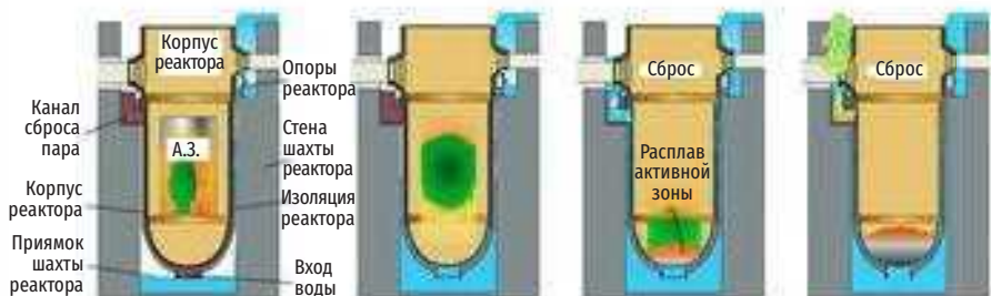
Рис. 3.22. Схема процесса охлаждения и удержания расплава активной зоны AP1000
