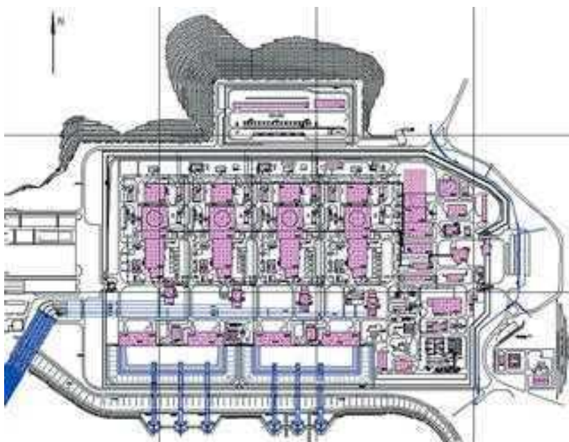
Рис. 2.65. Схема генерального плана АЭС «Аккую», проект В-509
