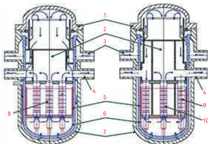
Рис. П2.38. Проекты реакторов ВВЭР-СКД. Двухзаходный (слева) и однозаходный (справа) варианты.
