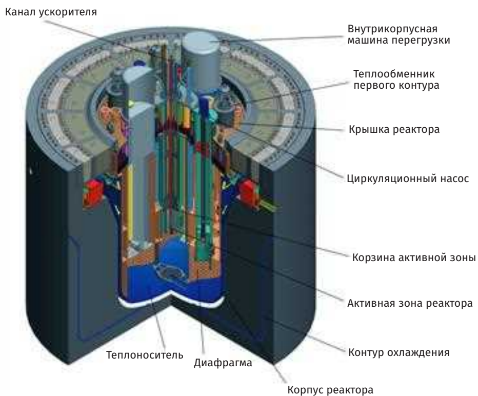
Рис. П2.17. Конструкция гибридного исследовательского реактора проекта MYRRHA ADS
