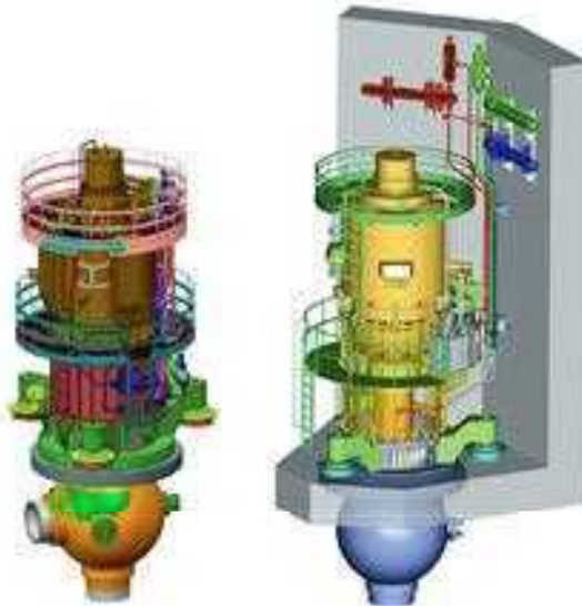
Рис. 2.55. ГЦНА-1753 (проект В-509) и ГЦНА-1391 (проект В-392М)
