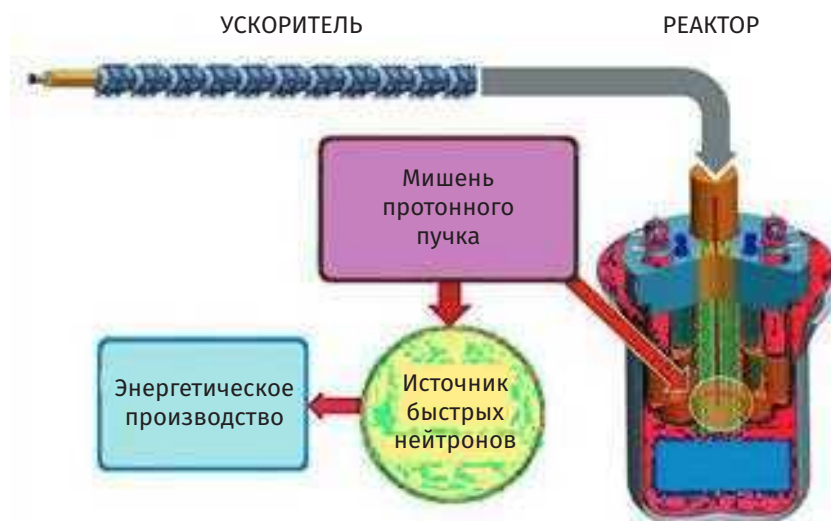
Рис. П2.18. Схема принципа действия реакторной установки MYRRHA ADS
