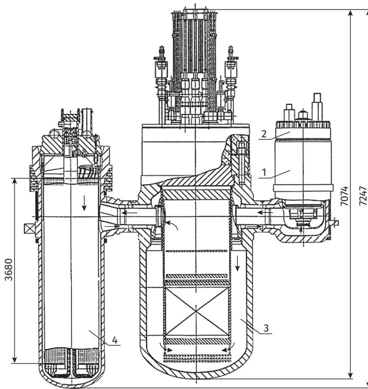
Рис. 1.21. Интегральный парогенерирующий блок РУ КЛТ-40С.
