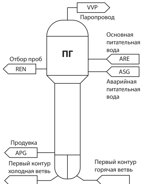
Рис. 3.103. Принципиальная схема парогенератора HPR1000
