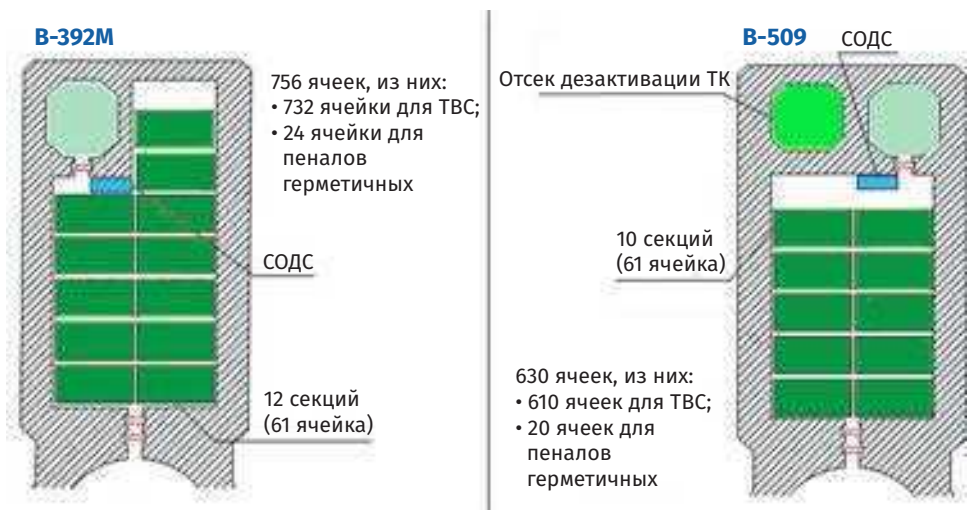
Рис. 2.71. Компоновка бассейна выдержки проекта В-509 АЭС «Аккую» и проекта В-392М (НВАЭС-2)
