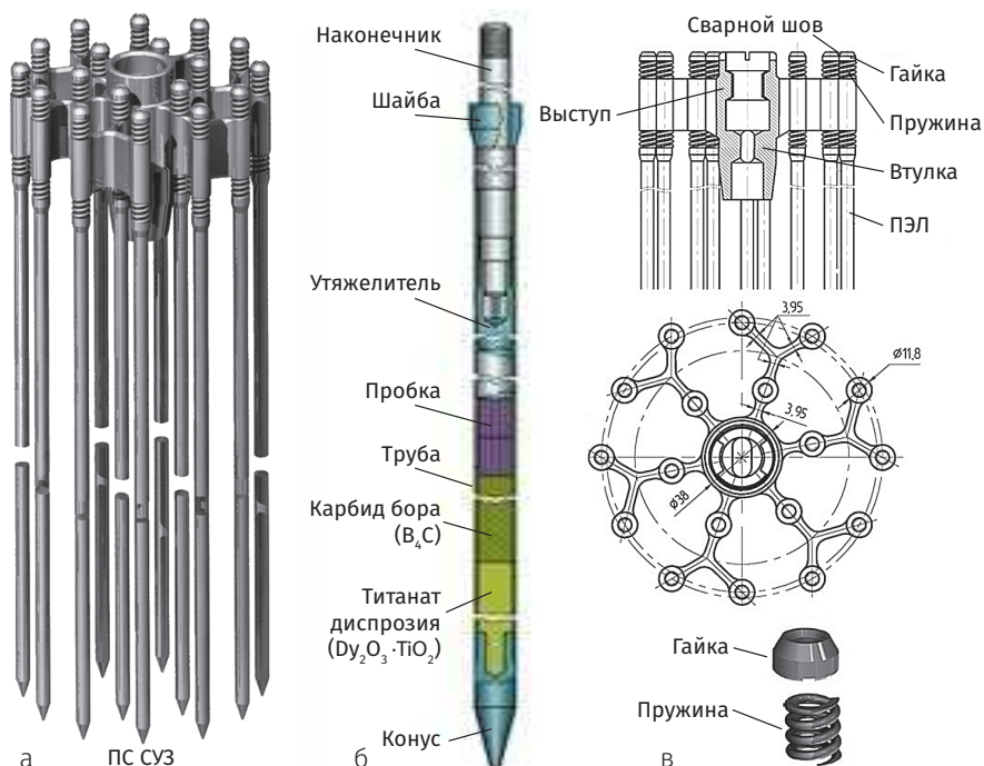
Рис. 2.13. Конструкция ПС СУЗ.
