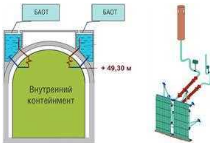
Рис. 2.42. Размещение оборудования СПОТ 3О по высоте. Проект В-491 (ЛАЭС-2)
