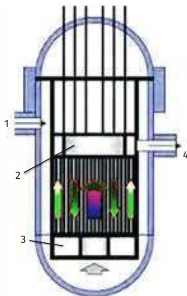
Рис. П2.33. Трехзаходная схема циркуляции теплоносителя в HPLWR.
