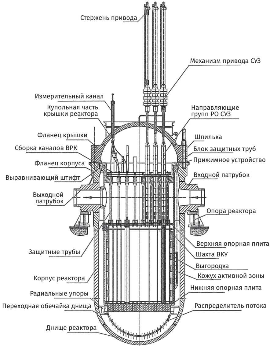
Рис. 3.92. Конструкция внутрикорпусных устройств реактора HPR1000
