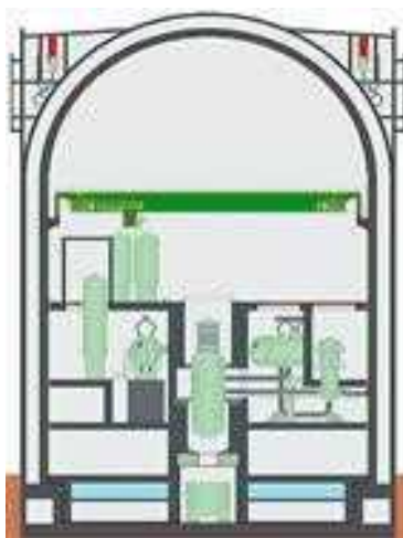
Рис. 2.46. Принципиальная схема ЗЛА. Проект В-491 (ЛАЭС-2)
