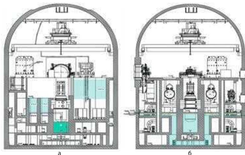
Рис. 2.82. Организация залива шахты реактора.
