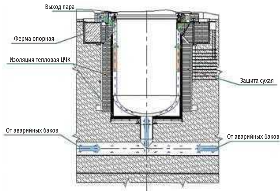
Рис. 2.84. Схема циркуляции воды в системе СУРОК с ее выпариванием через шахту реактора
