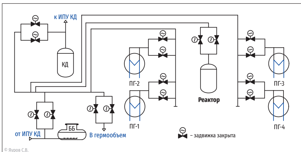
Рис. 2.63. Система аварийного газоудаления. Проект В-509 (АЭС «Аккую»)
