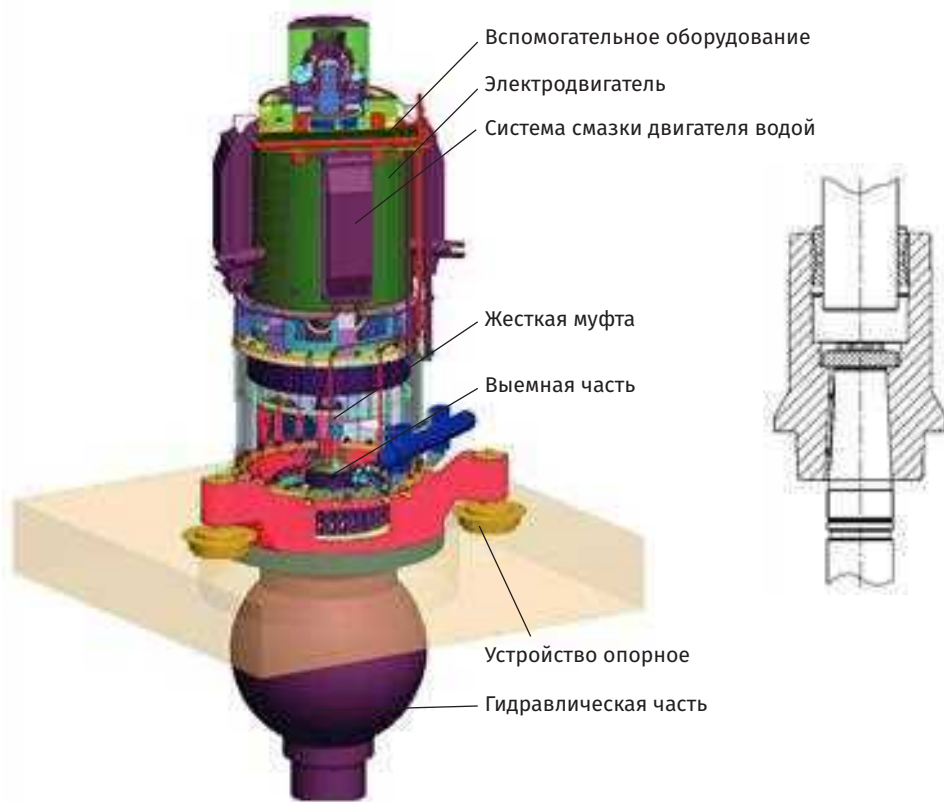
Рис. 2.79. Конструкция ГЦНА
