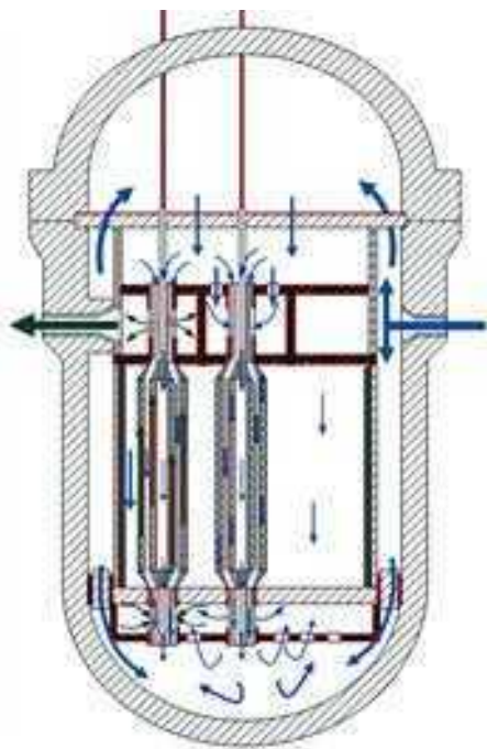
Рис. П2.36. Циркуляция потоков в реакторе CSR-1000
