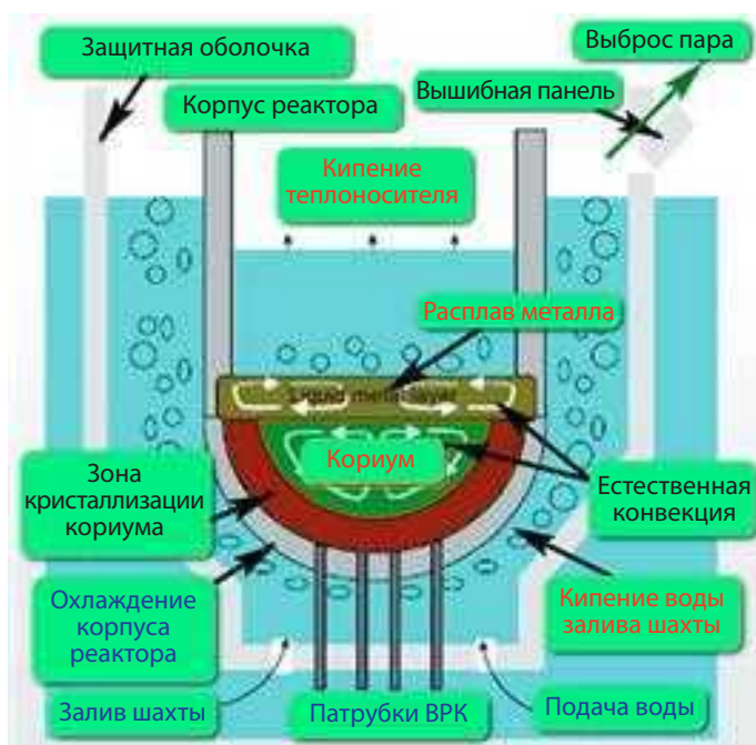
Рис. 3.80. Схема охлаждения корпуса реактора APR1400 при аварии с плавлением активной зоны
