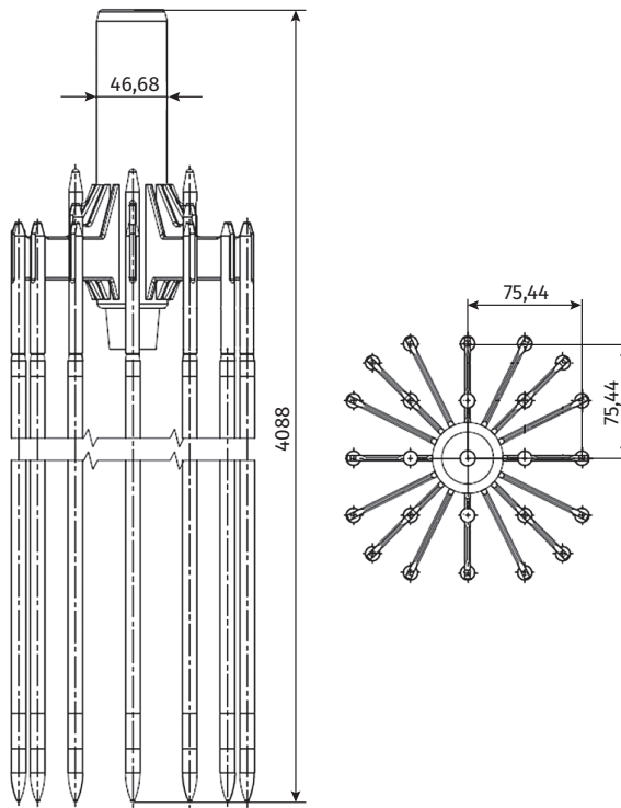
Рис. 3.95. Узел управления штанговым кластером СУЗ HPR1000
