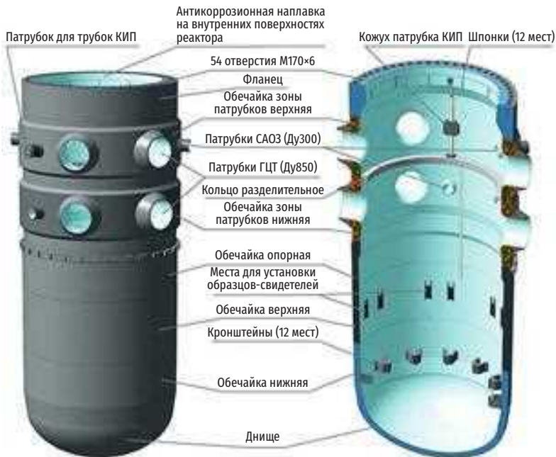
Рис. 2.5. Корпус реактора ВВЭР-1200. Проект В-392М (НВАЭС-2)
