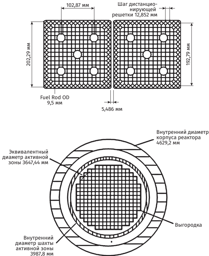
Рис. 3.61. Схема размещения активной зоны в поперечном сечении корпуса реактора APR1400
