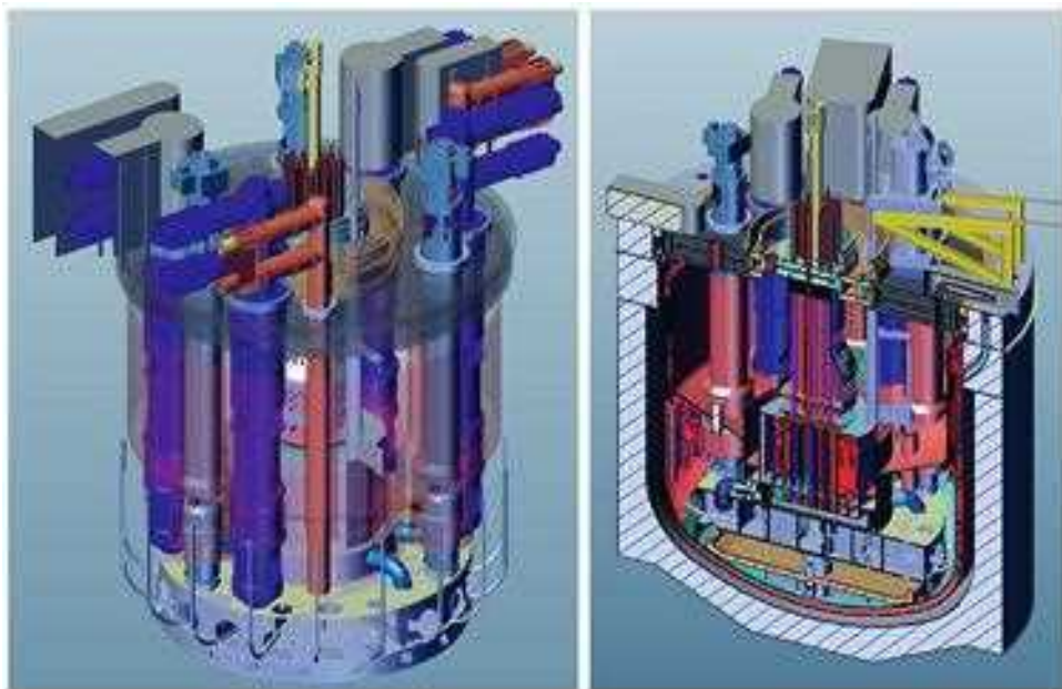
Рис. П2.23. Общий вид конструкции реактора ASTRID
