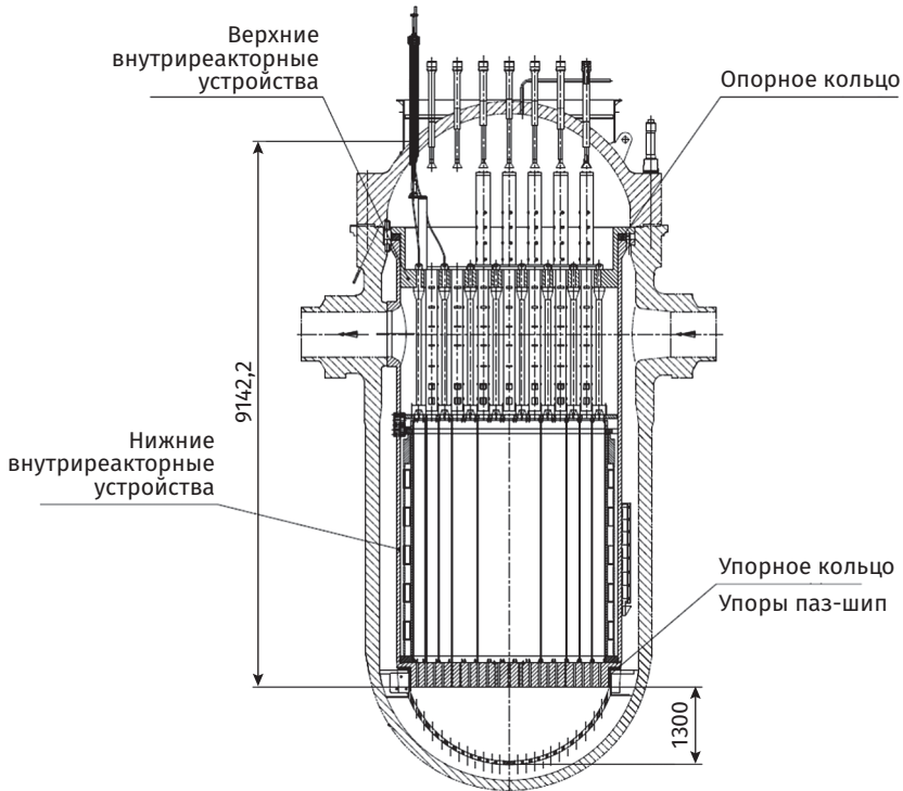
Рис. 3.88. Общий вид устройств реактора HPR1000
