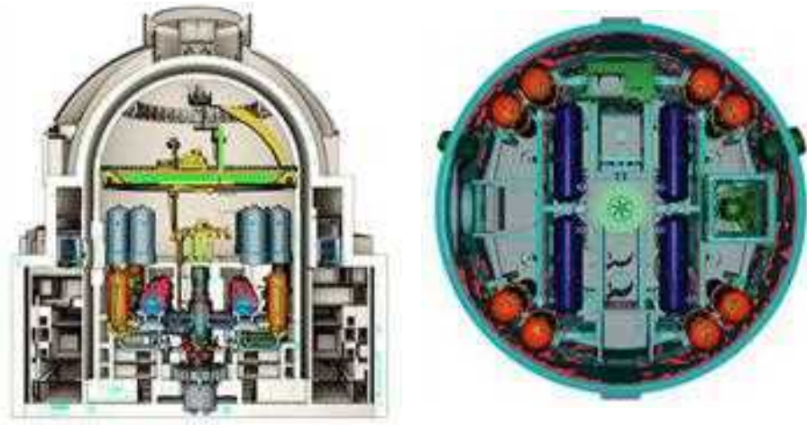
Рис. 2.73. Расположение оборудования в гермооболочке проекта ВВЭР-ТОИ
