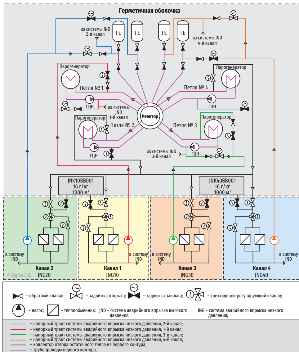
Рис. 2.37. Схема четырех каналов системы отвода остаточного тепла JNA. Проект В-491 (ЛАЭС-2)
