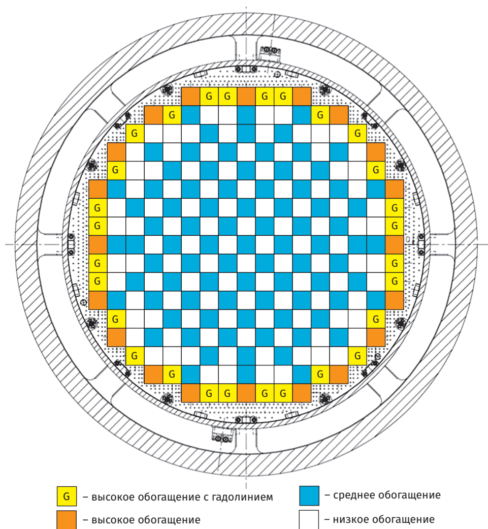
Рис. 3.31. Картограмма активной зоны реактора EPR-1600
