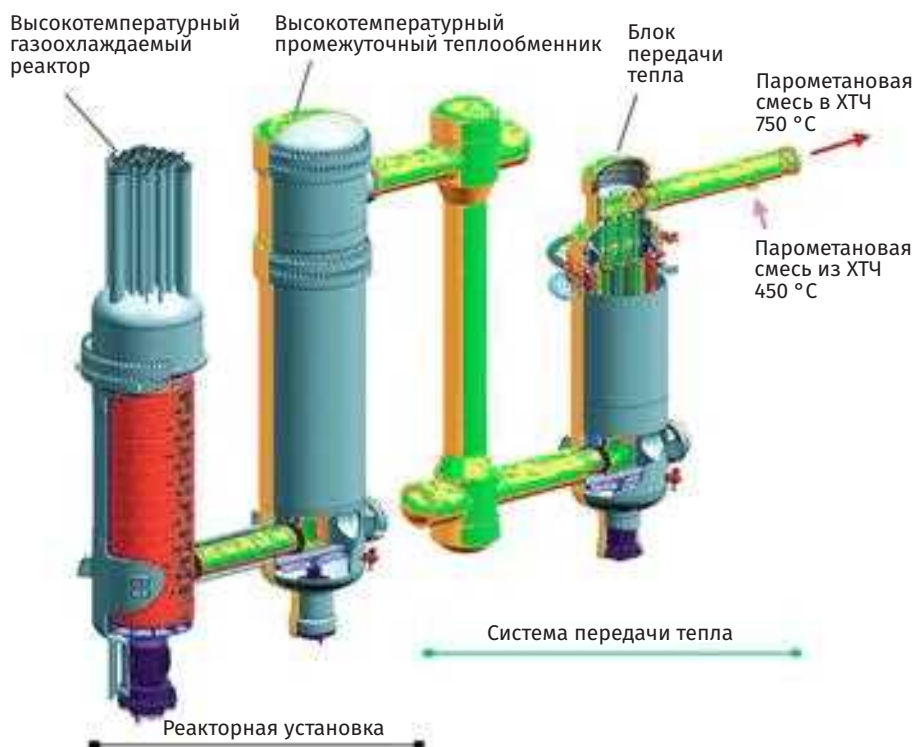
Рис. П2.43. Компоновка ядерной части АЭТС с РУ ВТГР-200В и системы передачи тепла
