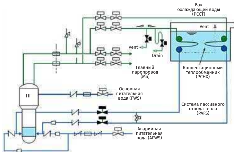
Рис. 3.75. Блок-схема и принципиальная схема канала системы пассивного отвода тепла (PAFS) APR+
