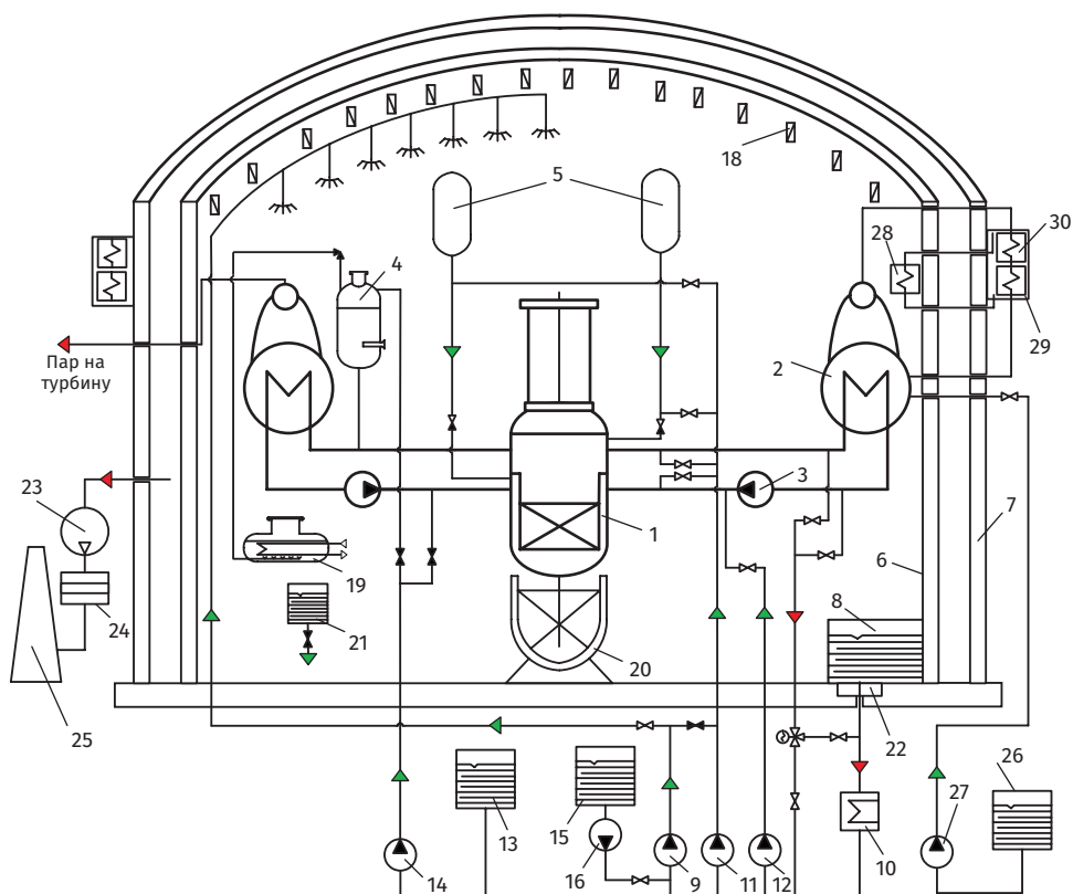
Рис. 2.33. Общая структура систем безопасности проекта РУ В-491 (ЛАЭС-2).
