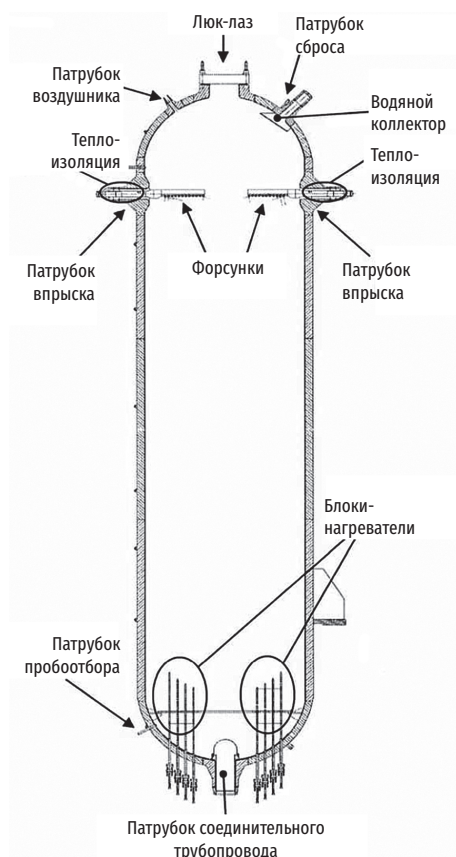
Рис. 3.35. Компенсатор давления EPR-1600 в разрезе
