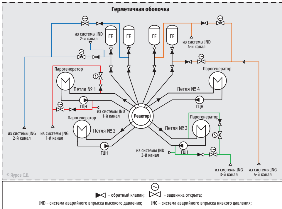
Рис. 2.38. Упрощенная схема пассивной части CAO3. Проект В-491 (ЛАЭС-2)
