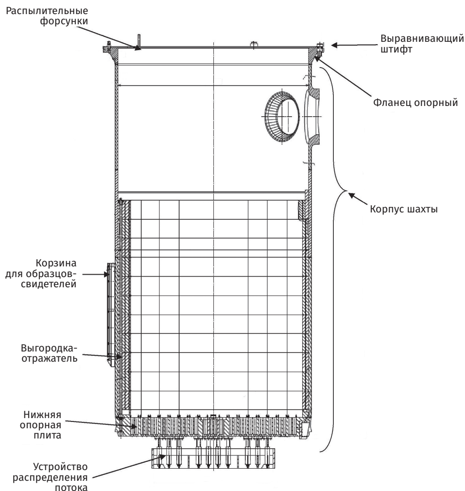
Рис. 3.29. Разрез шахты активной зоны реактора EPR-1600 с выгородкой-отражателем обеспечивают однородное охлаждение активной зоны. Нижние внутрикорпусные устройства ограничивают механические нагрузки от основных компонентов и позволяют загружать, выгружать и перегружать ТВС. Нижние внутренние устройства служат для достижения однородного распределения потока теплоносителя в активной зоне, чтобы свести к минимуму увеличение подъемных сил на тепловыделяющие сборки и вибрации топливных стержней, вызванных движением теплоносителя первого контура за счет работы ГЦН.
