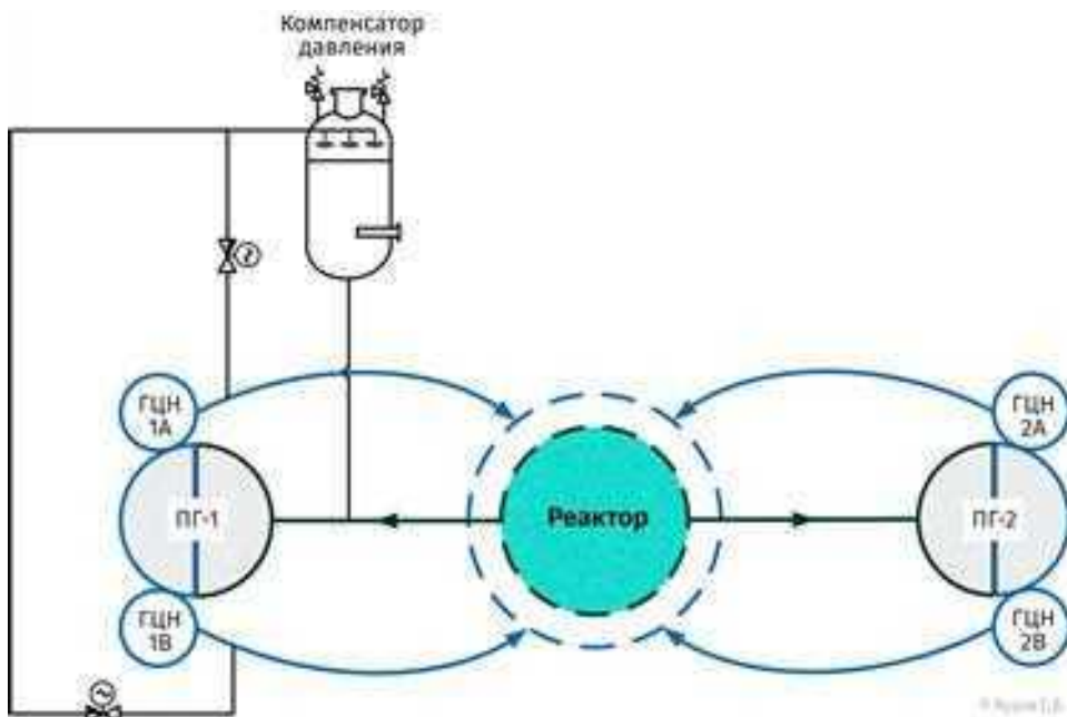
Рис. 3.2. Принципиальная схема первого контура — системы охлаждения реактора (RCS) AP1000
