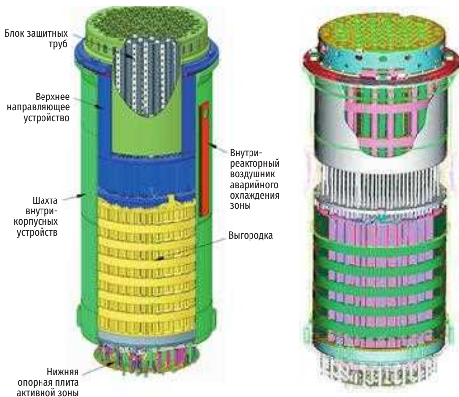
Рис. 3.56. Конструкция и компоненты внутрикорпусных устройств реактора APR1400
