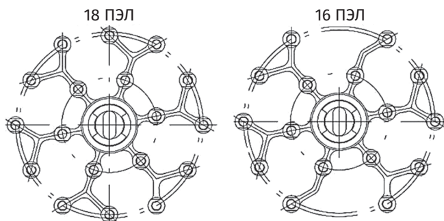
Рис. 2.54. Конструкция ПС СУЗ проекта В-509
