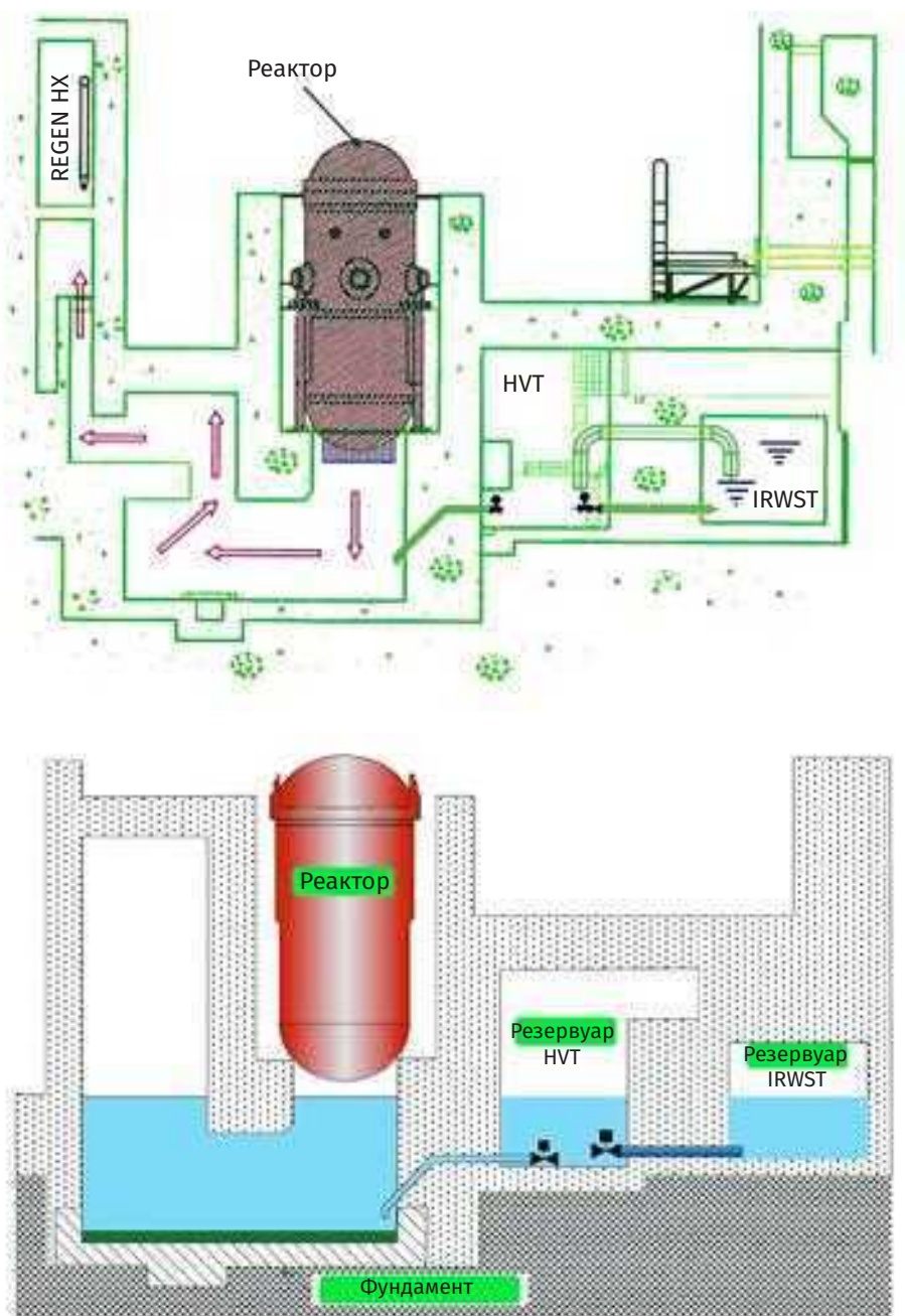
Рис. 3.79. Общая конструкция шахты реактора и схема принципа действия системы затопления шахты реактора (CFS) APR1400
