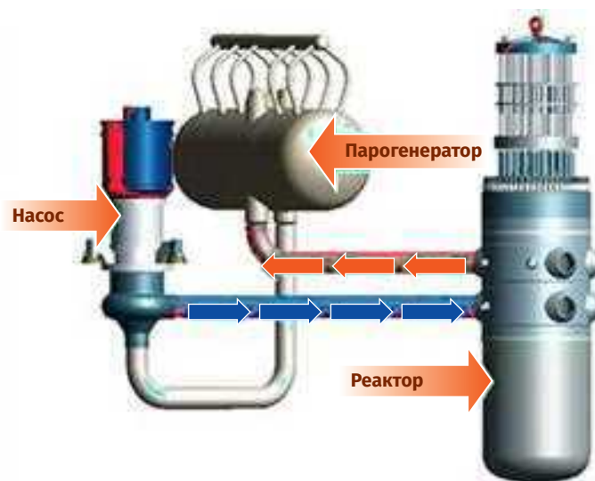
Рис. 2.3. Циркуляционная петля первого контура ВВЭР-1200. Проект В-392М (НВАЭС-2)
