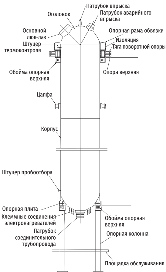
Рис. 3.9. Конструкция компенсатора давления и опорной системы AP1000
