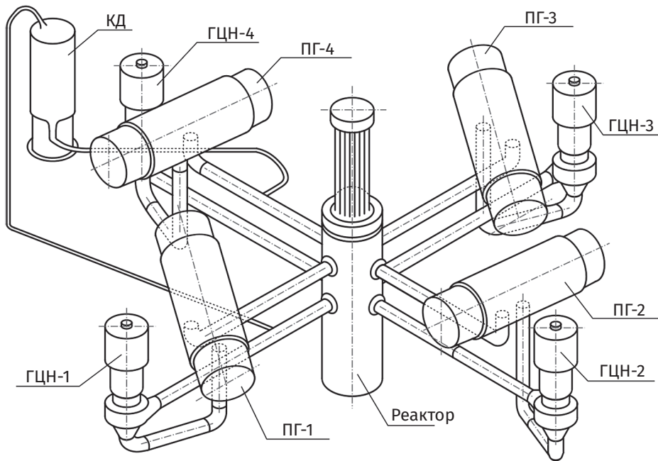
Рис. 1.14. Схема оборудования первого контура ВВЭР-1000.
