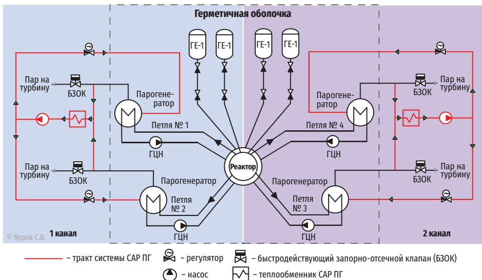
Рис. 2.61. Система аварийного расхолаживания ПГ, проект В-509 (АЭС «Аккую»)
