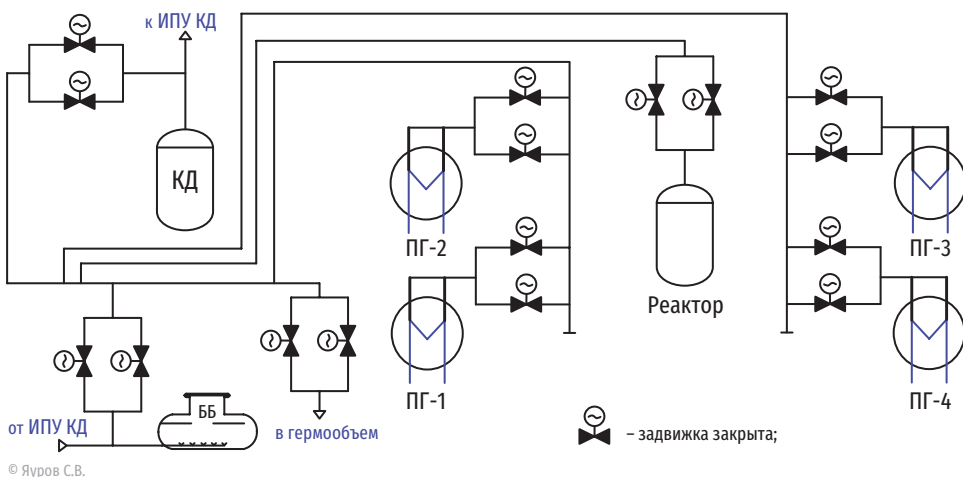
Рис. 2.27. Система аварийного газоудаления. Проект В-392М (НВАЭС-2)
