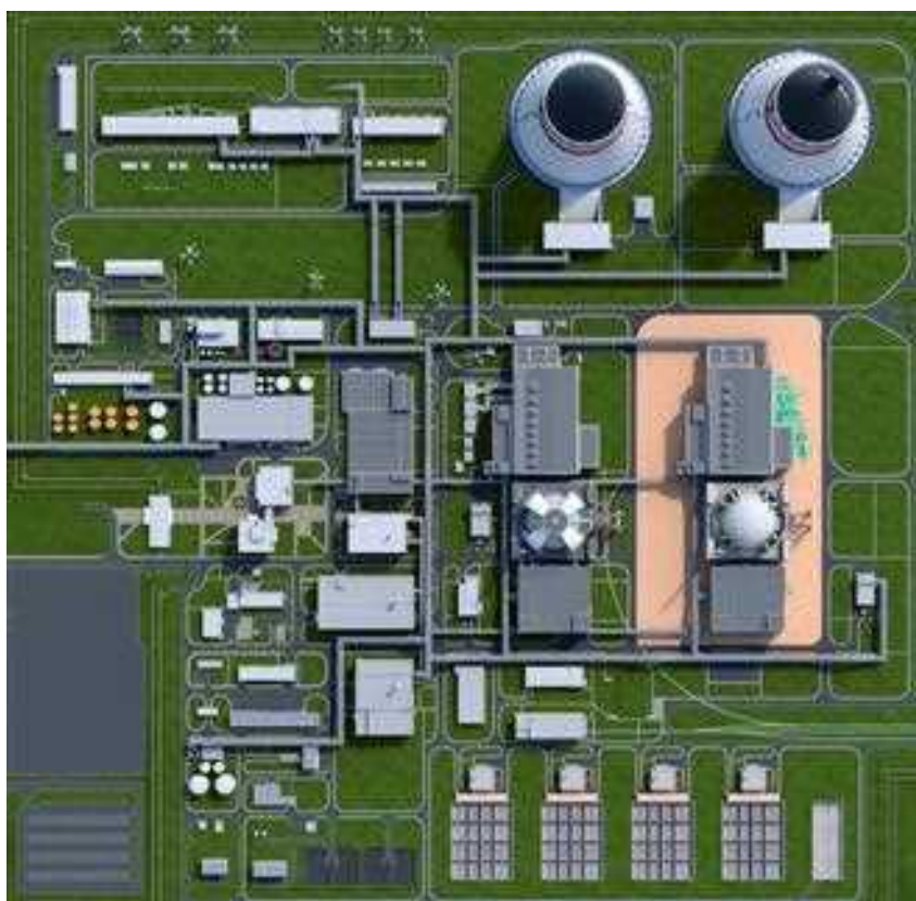
Рис. 2.31. Схема генерального плана Нововоронежской АЭС-2 с энергоблоками №1 и №2
