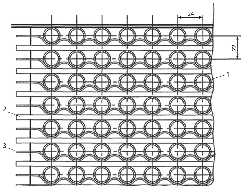
Рис. 2.19. Коридорная компоновка теплообменных труб ПГВ-1000МКП.
