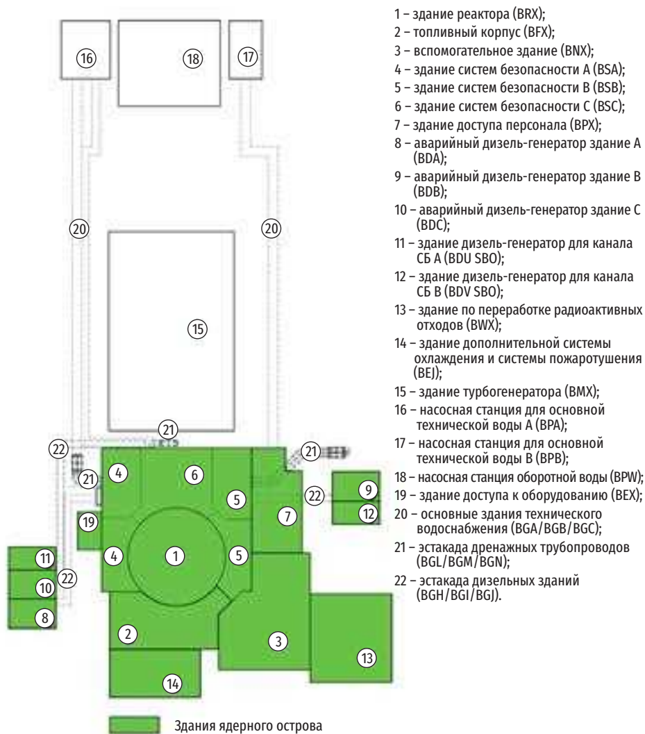
Рис. 3.114. Типичная компоновка зданий площадки для одного блока HPR 1000
