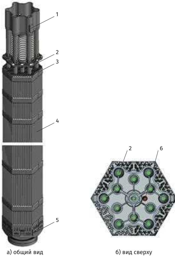
Рис. 2.77. Тепловыделяющая сборка РУ проекта В-551С.
