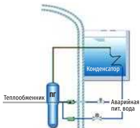
Рис. 3.108. Принципиальная схема аварийной системы питательной воды ПГ HPR1000 [ASG (EFWS)]
