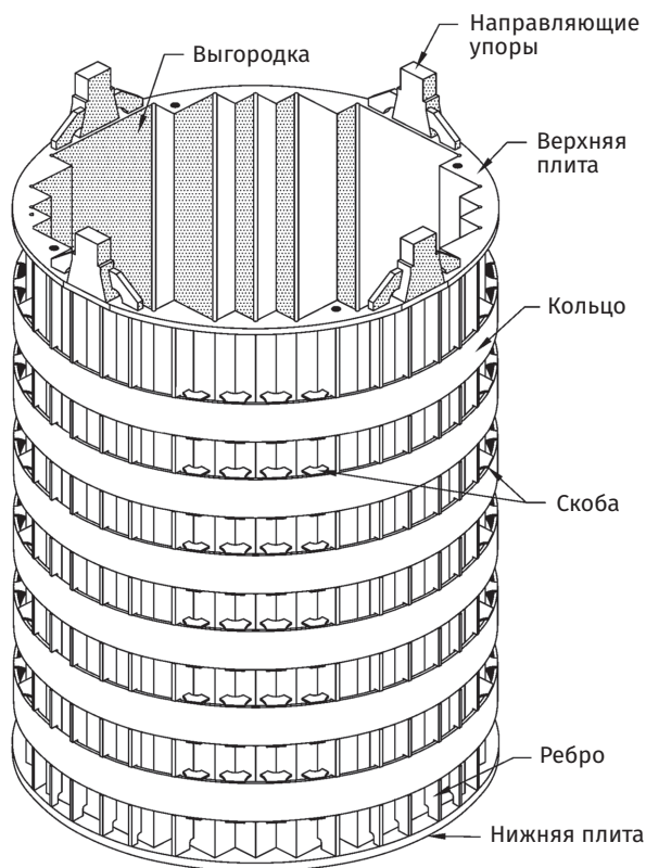
Рис. 3.59. Выгородка активной зоны РУ APR1400
