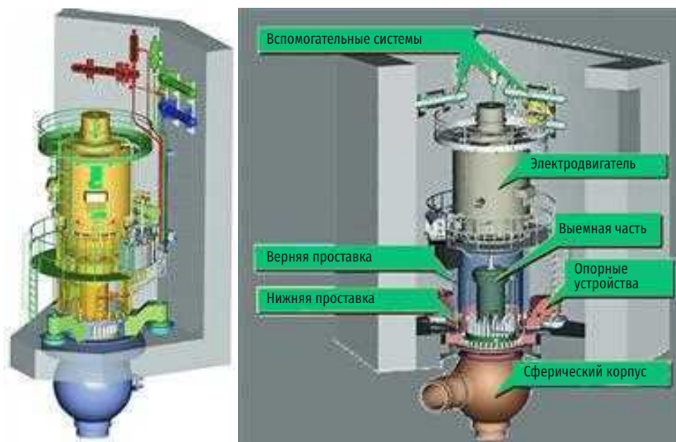
Рис. 2.16. Общий вид ГЦНА-1391
