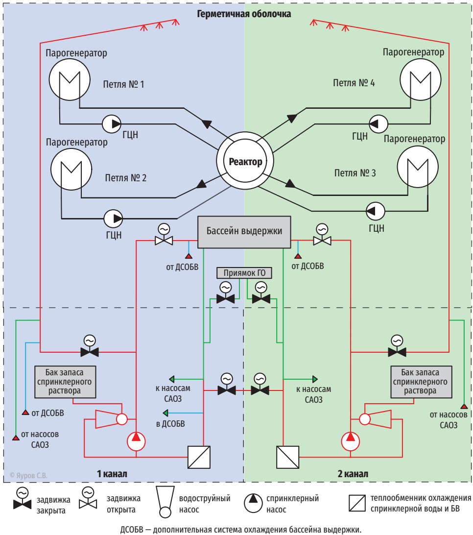
Рис. 2.64. Технологическая схема системы JMN. Проект В-509 (АЭС «Аккую»)
