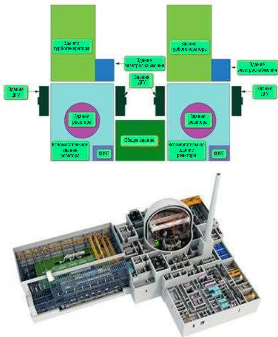
Рис. 3.82. Общее расположение зданий площадки с двумя энергоблоками APR1400
