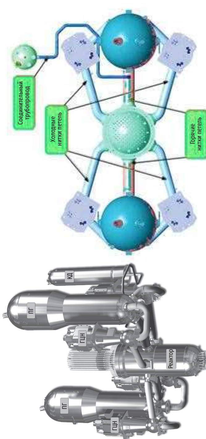
Рис. 3.50. Общий вид основного оборудования реакторной установки APR1400
