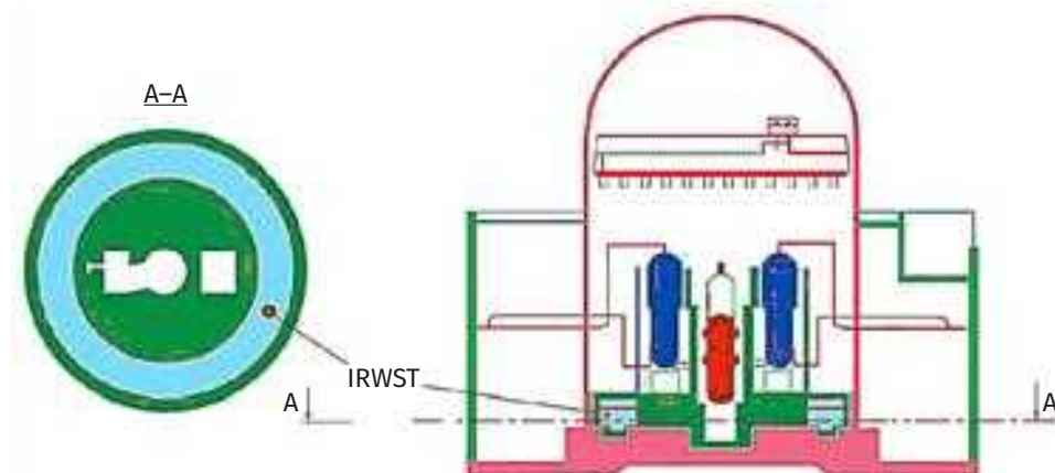
Рис. 3.73. Расположение кольцевого резервуара для хранения воды в защитной оболочке APR1400 (IRWST)
