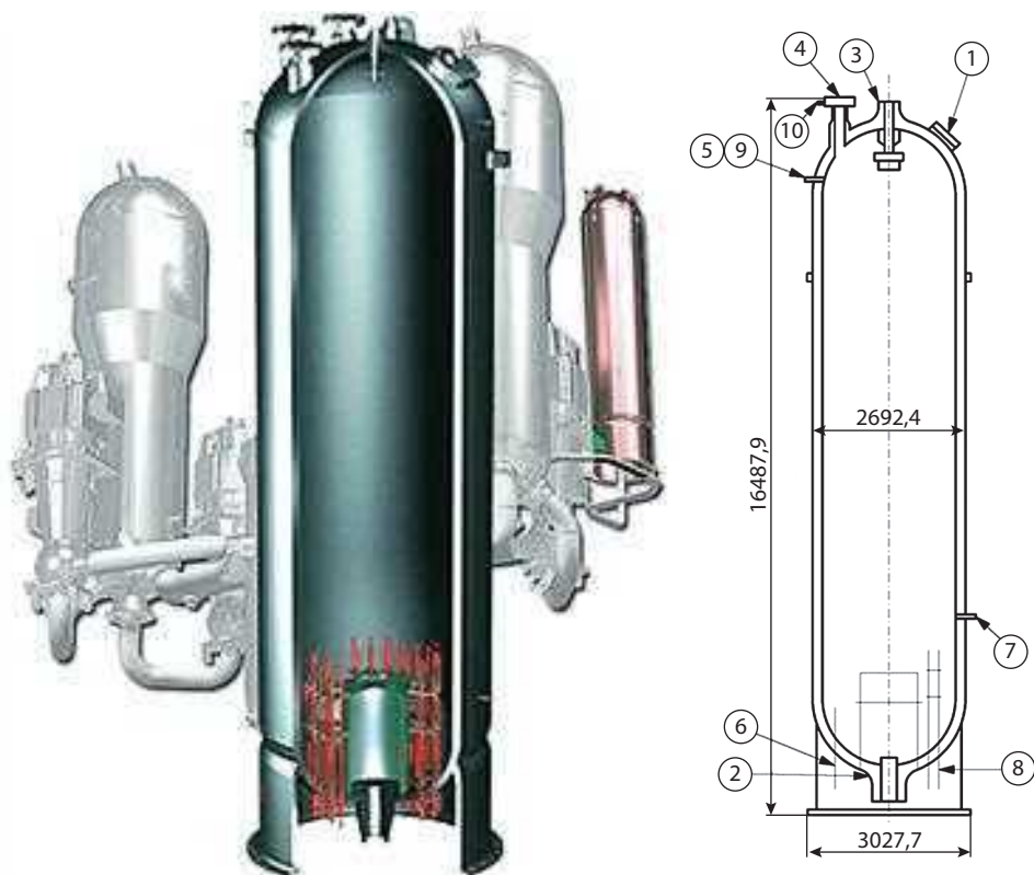
Рис. 3.65. Конструкция, патрубки и основные размеры компенсатора давления APR1400.
