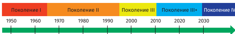
Рис. П2.1. Развитие реакторных установок
