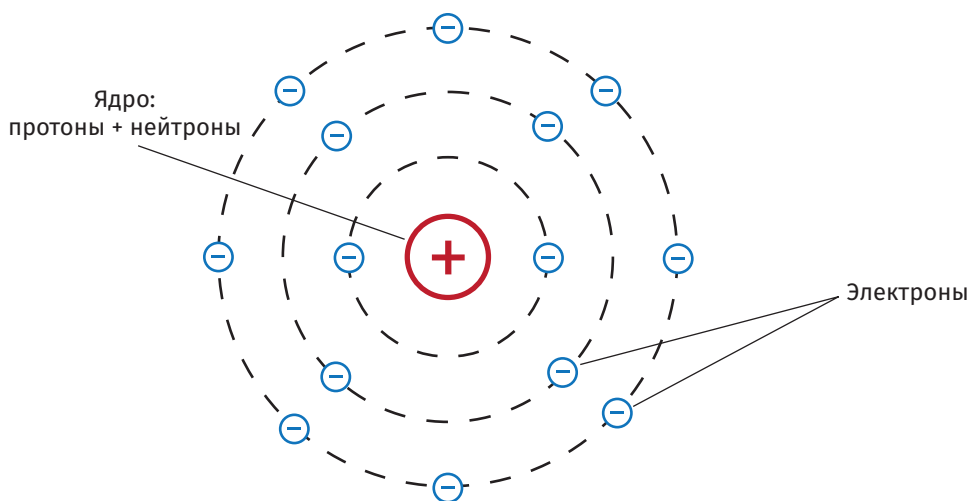
Рис. 1.1. Планетарная модель атома
