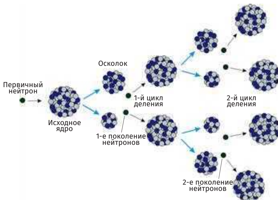
Рис. 1.3. Цепная реакция деления
