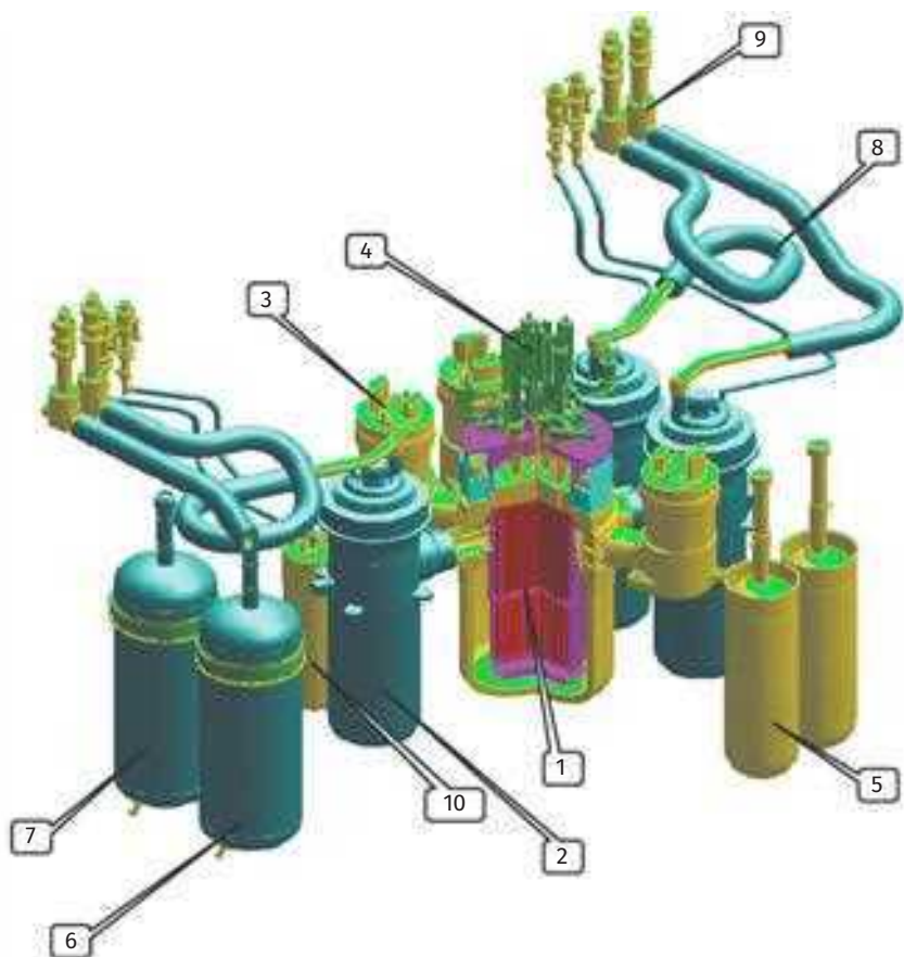
Рис. 1.20. Реакторная установка КЛТ-40С.
