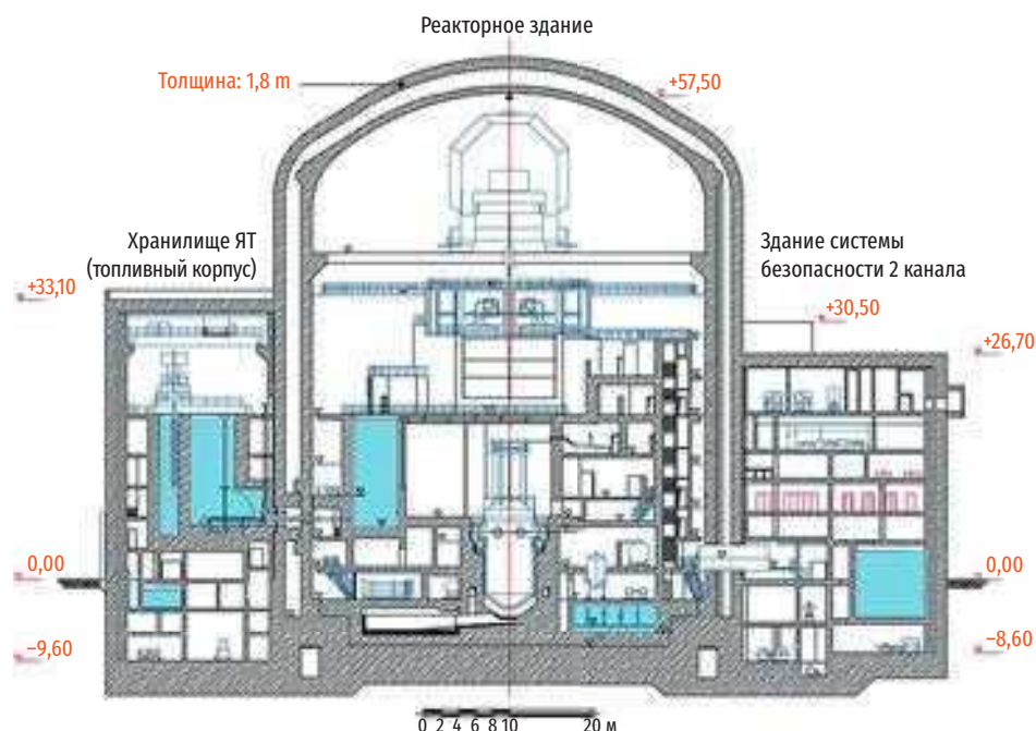
Рис. 3.48. Расположение систем РУ в реакторном здании энергоблока с EPR-1600 (вертикальный разрез)
