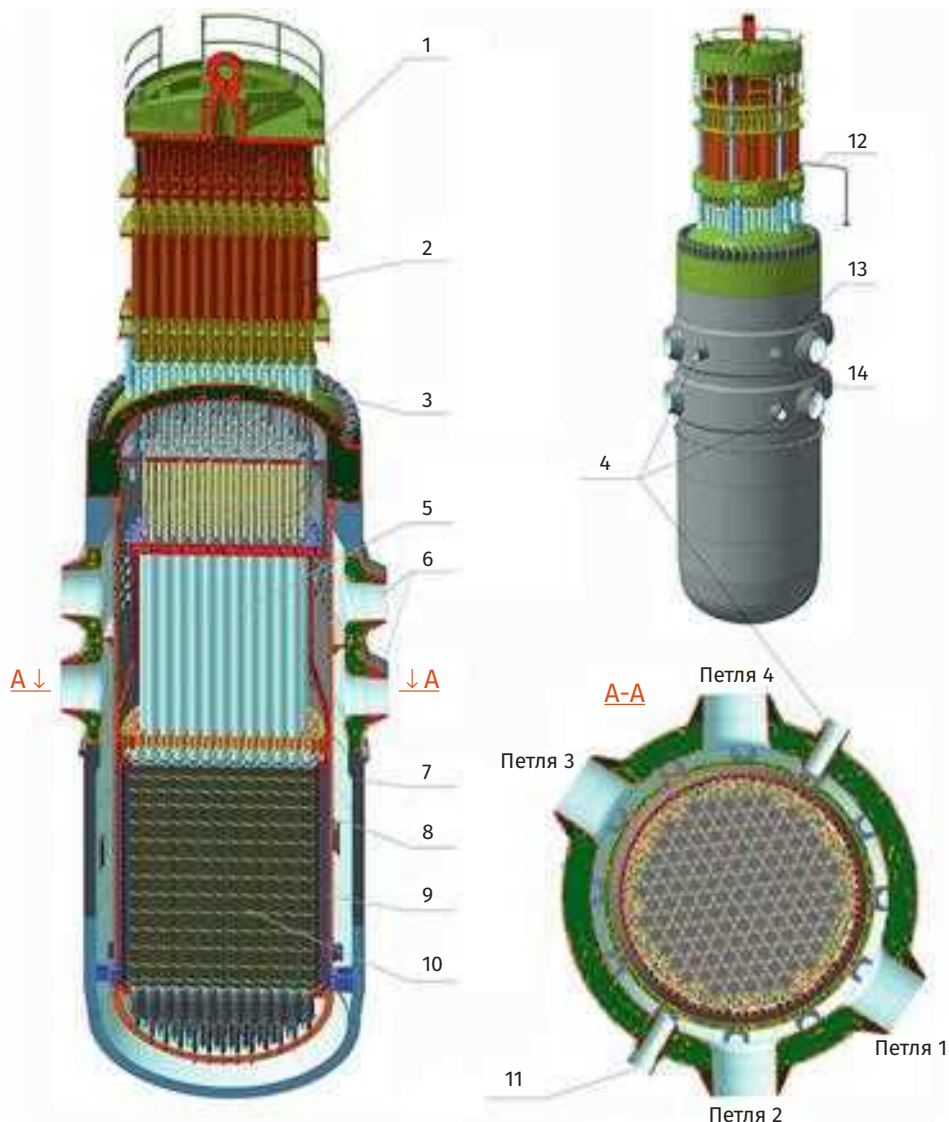
Рис. 2.4. Конструкция реактора ВВЭР-1200. Проект В-392М (НВАЭС-2).
