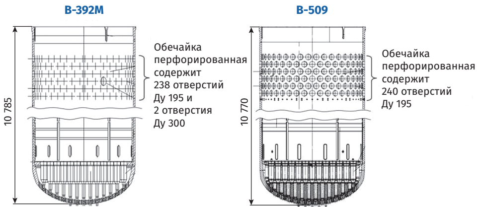
Рис. 2.52. Сравнение шахт внутрикорпусных проектов В-392М и В-509
