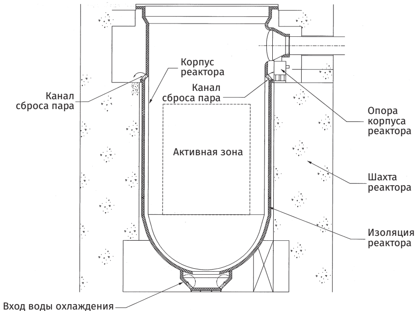
Рис. 3.20. Конструкция системы удержания расплава активной зоны AP1000
