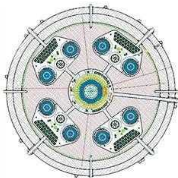
Рис. П2.12. Конструкция РУ БРЕСТ-ОД-300 (вид сверху)
