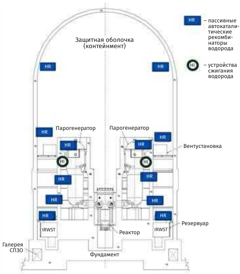
Рис. 3.78. Схема размещения пассивных автокаталитических рекомбинаторов водорода и электротермических устройств сжигания водорода в объеме защитной оболочки APR1400
