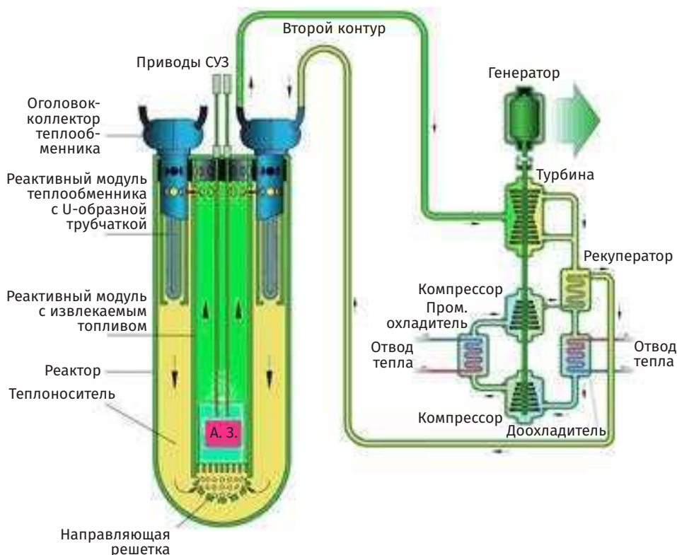
Рис. П2.9. Тепловая схема реактора на быстрых нейтронах со свинцовым теплоносителем LFR
